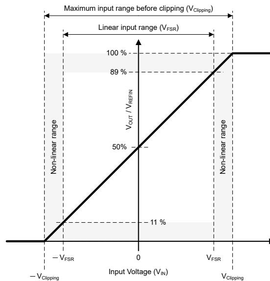
图 7-3. AMC0x02R 的输入到输出传送曲线
