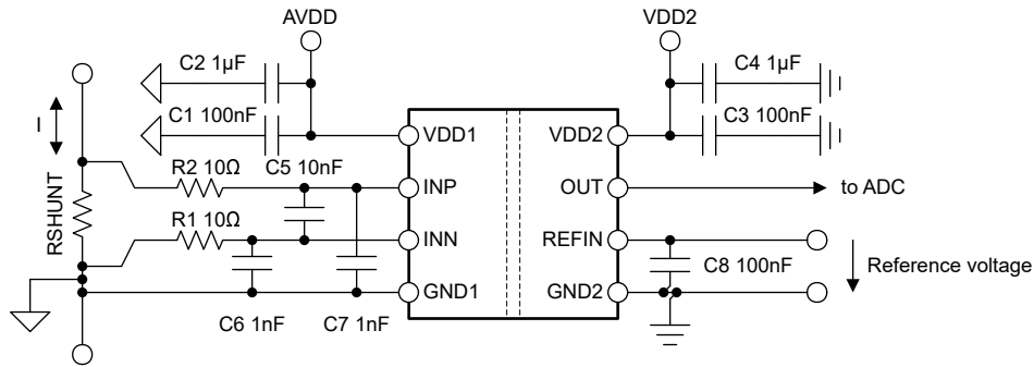
图 8-6. AMC0x02R 去耦
