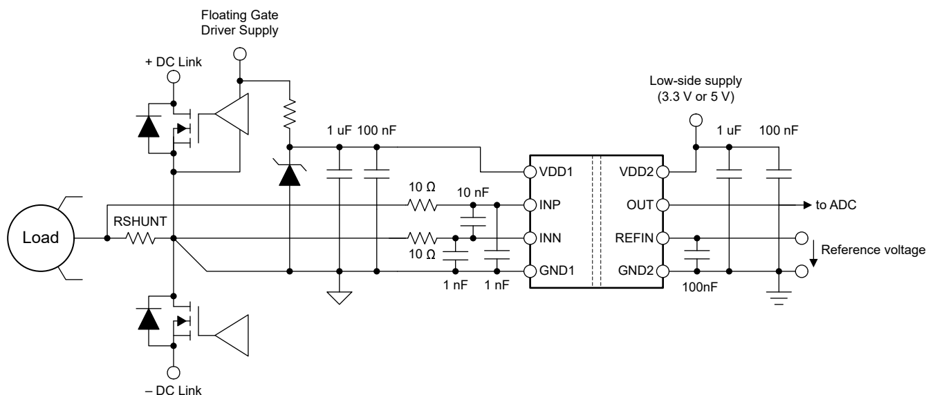
图 8-1. 在典型应用中使用 AMC0x02R 进行电流检测
