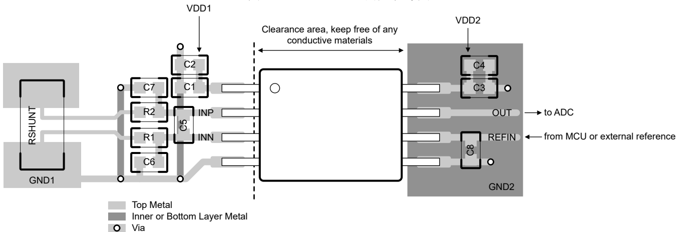
图 8-7. AMC0x02R 的建议布局
