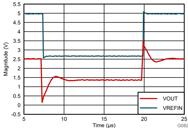
图 8-5. AMC0x02R 的参考输入阶跃响应
