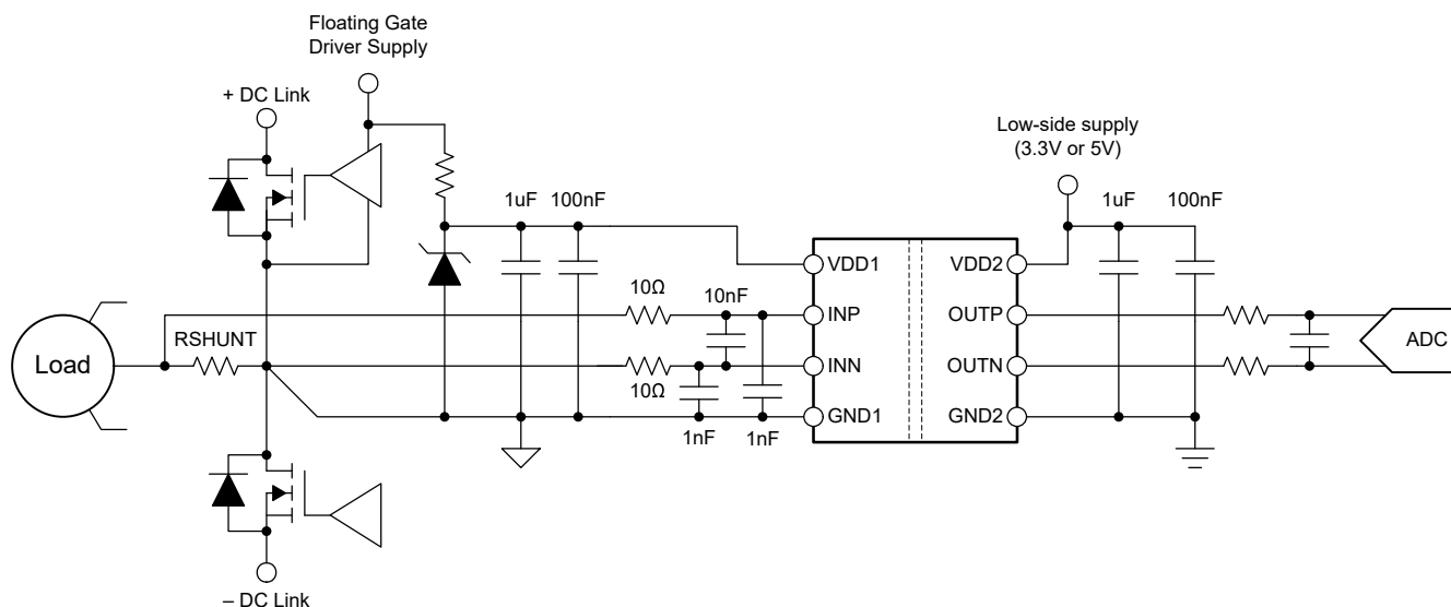
图 8-1. 在典型应用中使用 AMC0x02D 进行电流检测
