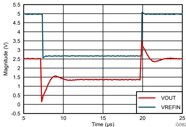
图 8-5. AMC0x02R 的参考输入阶跃响应
