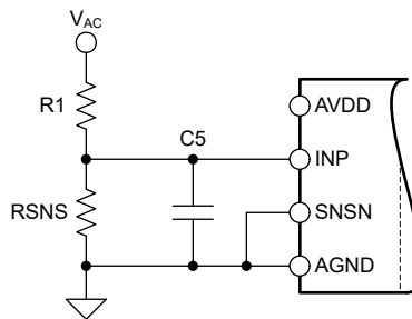
图 7-2. 输入滤波器
