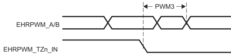
图 6-44. EHRPWM Switching Characteristics
