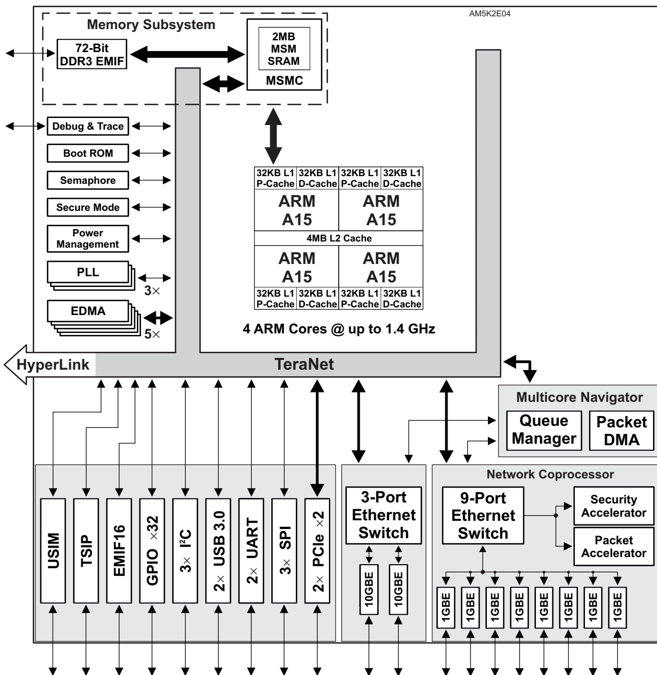
图 1-1. AM5K2E04 功能框图
