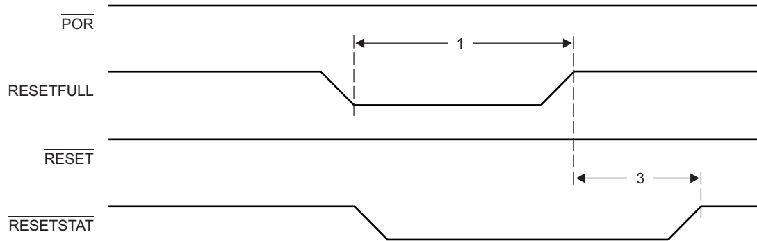
图 10-4. RESETFULL Reset Timing
