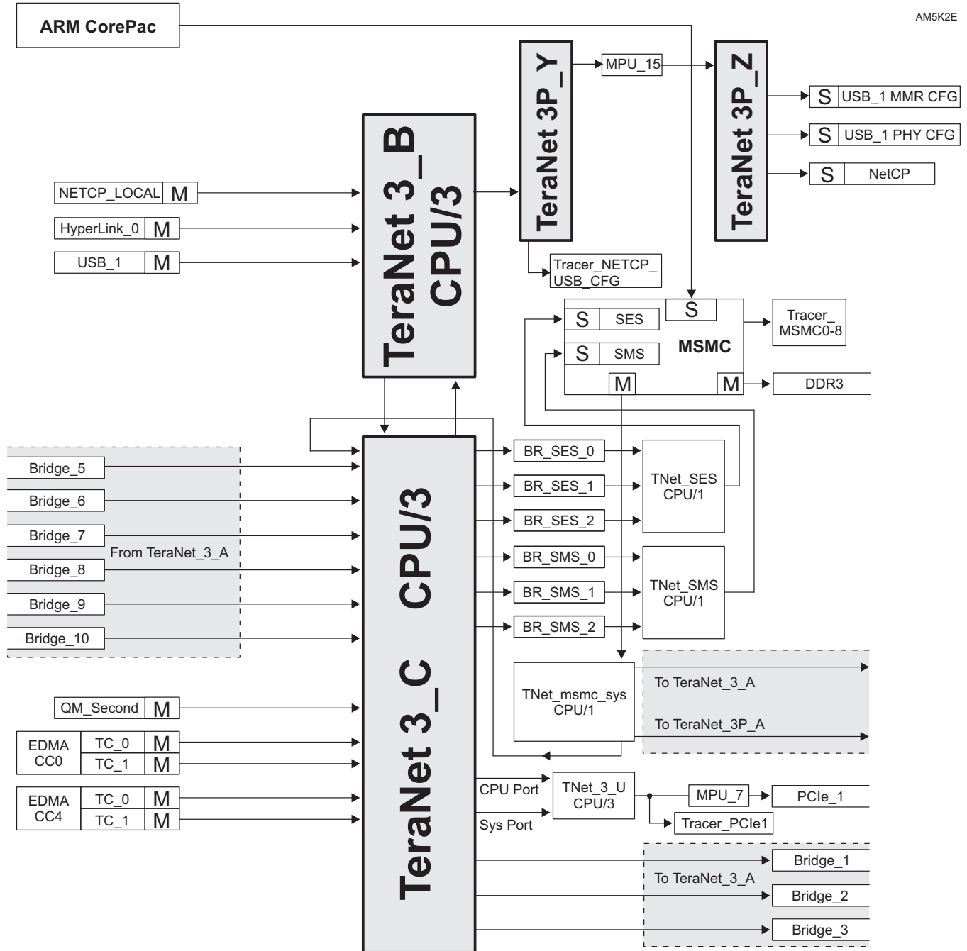
图 7-3. TeraNet 3_C
