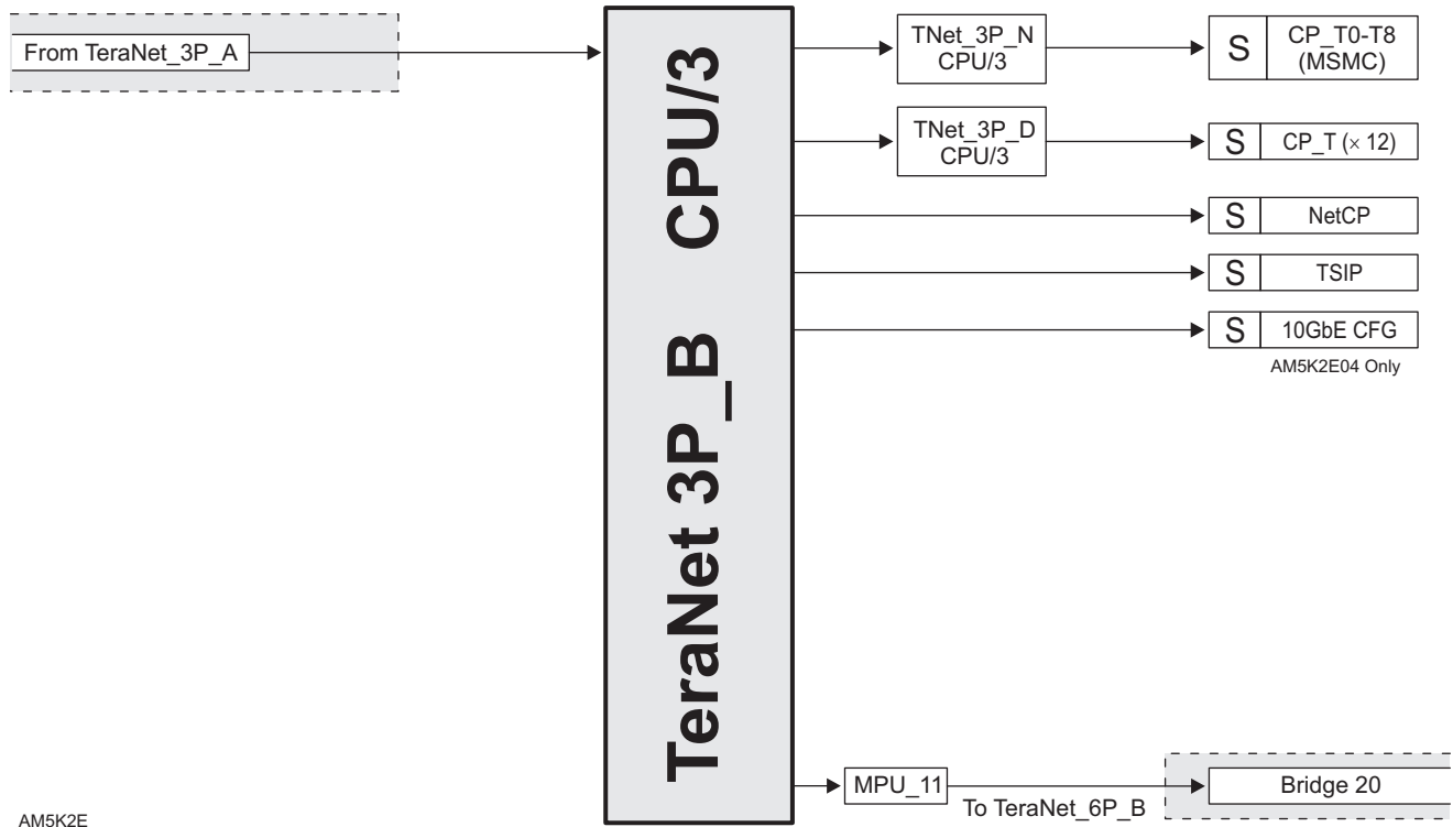
图 7-5. TeraNet 3P_B
