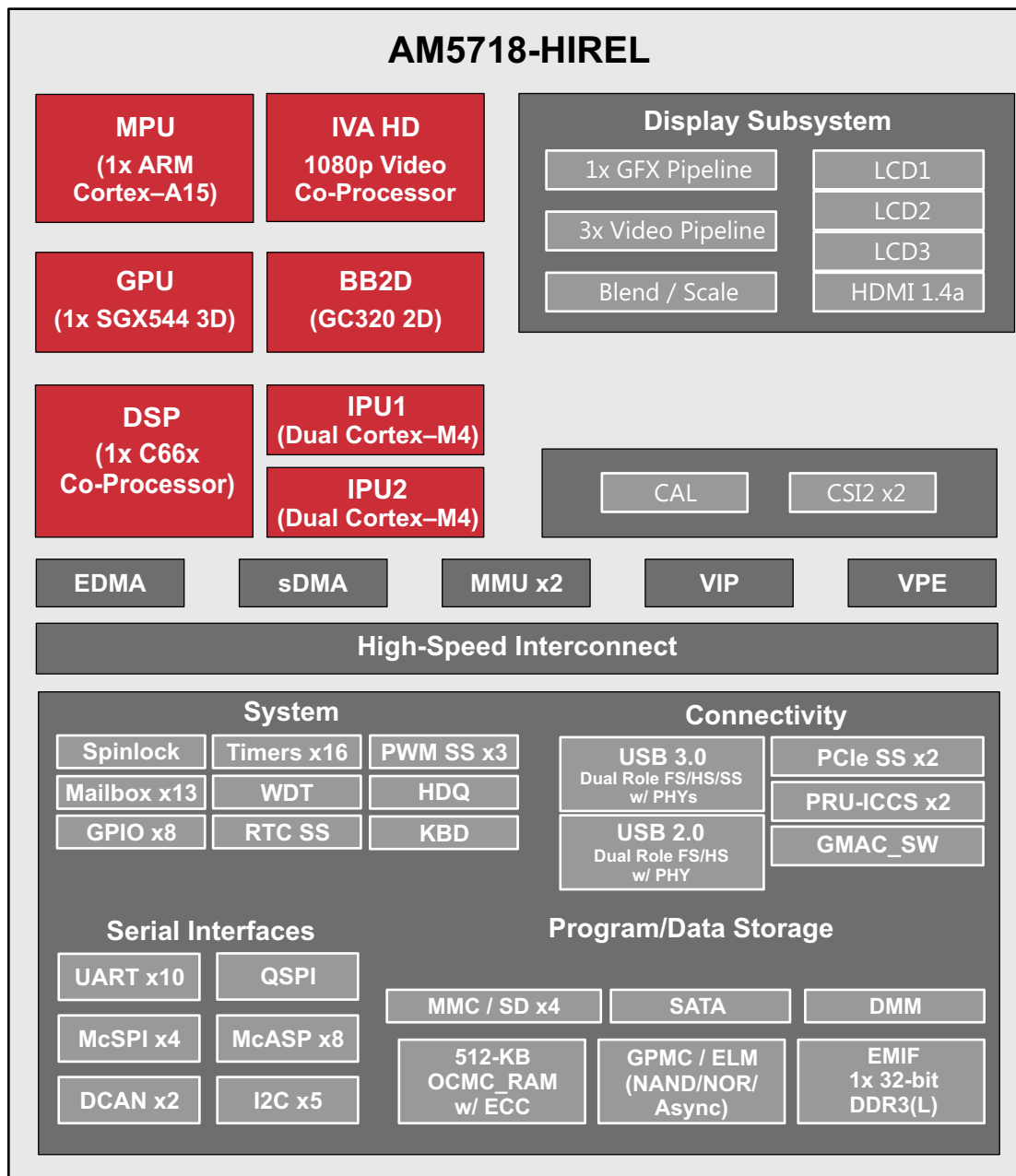
图 1-1. AM5718-HIREL 方框图
