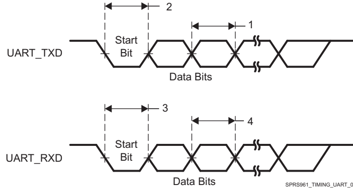
图 5-45. UART Timing
