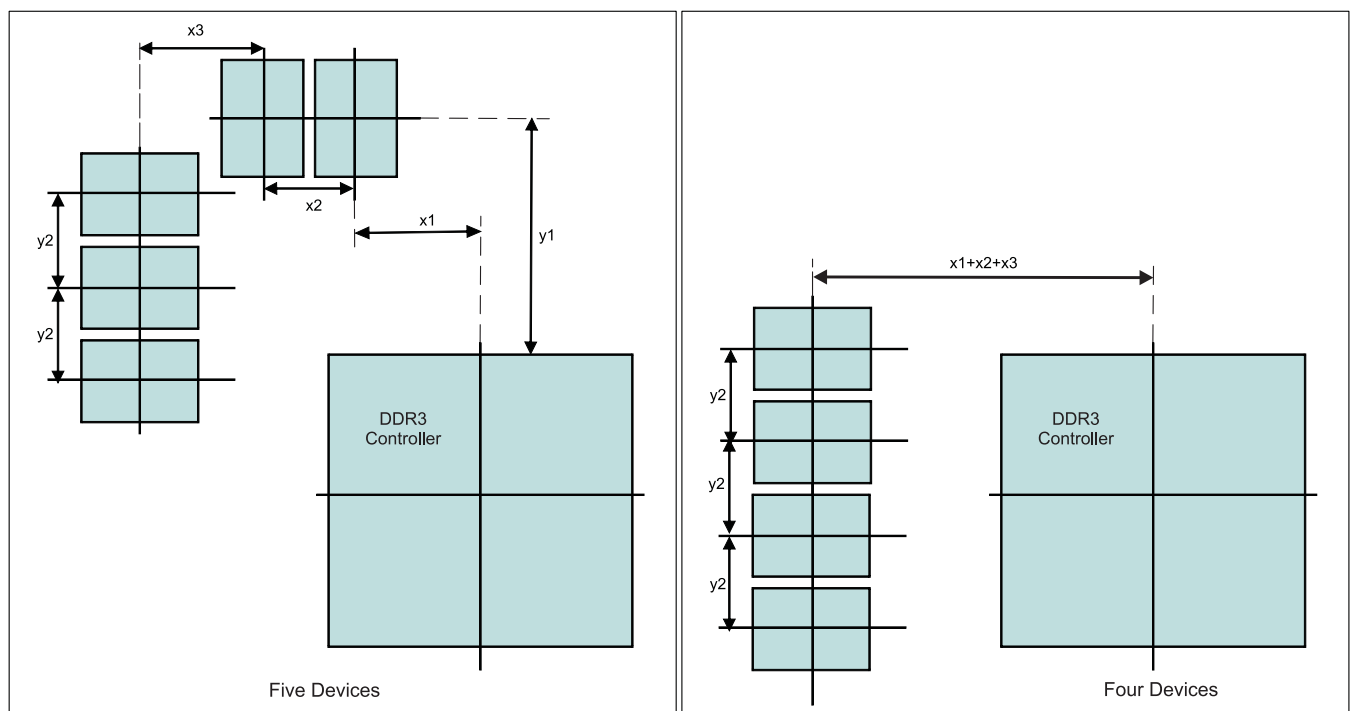
图 7-4. Placement Specifications
