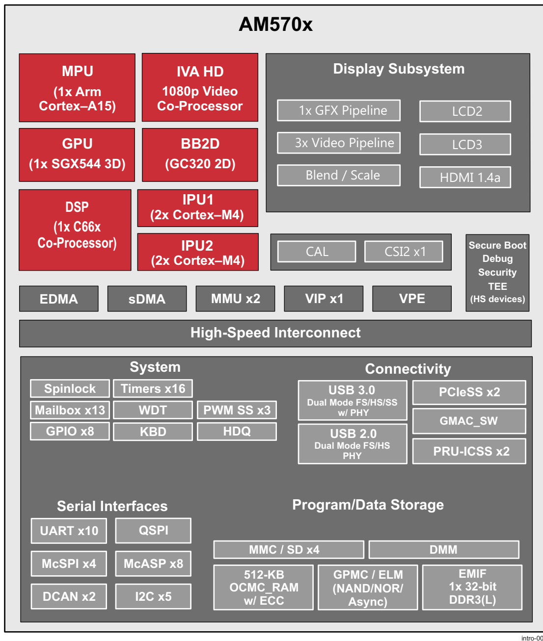
图 1-1. AM570x 方框图
