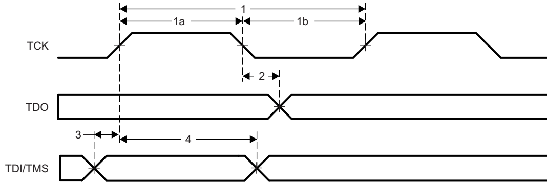
图 5-125. JTAG Timing
