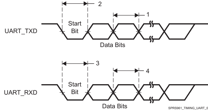
图 5-45. UART Timing
