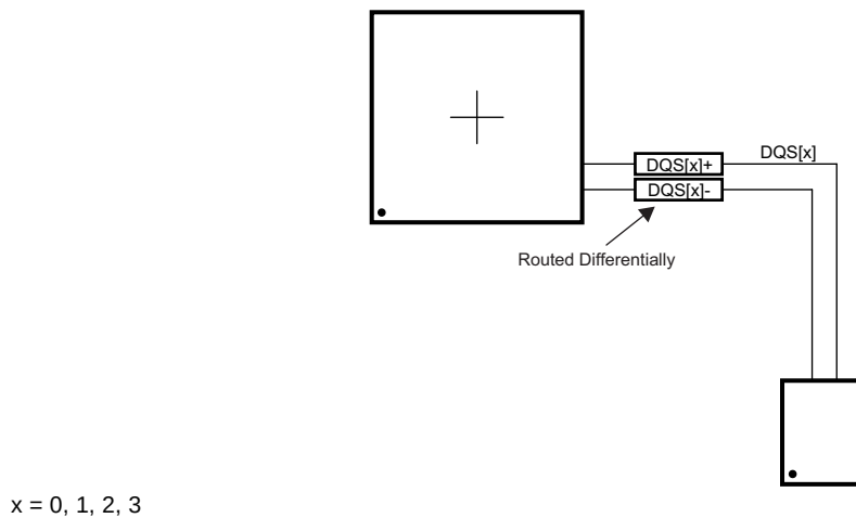
图 5-85. DQS[x] Routing
