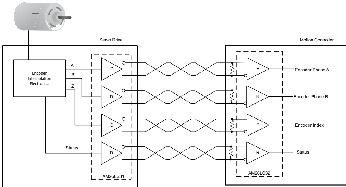
图 8-1. 编码器应用
