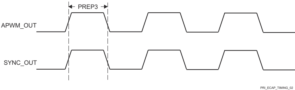
图 6-67. PRU-ICSS ECAP 开关特性
