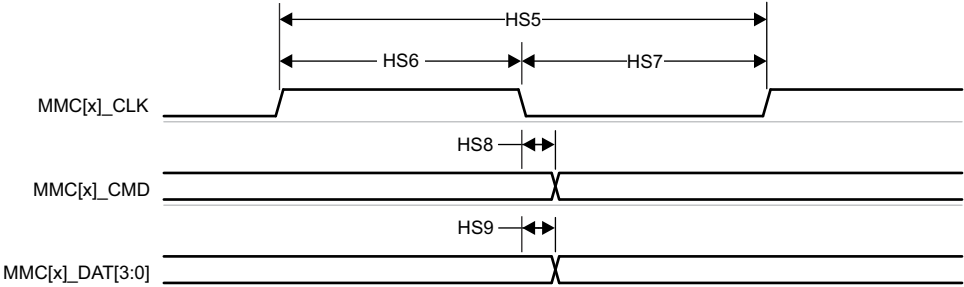
图 6-49. MMC - 高速 - 发送模式
