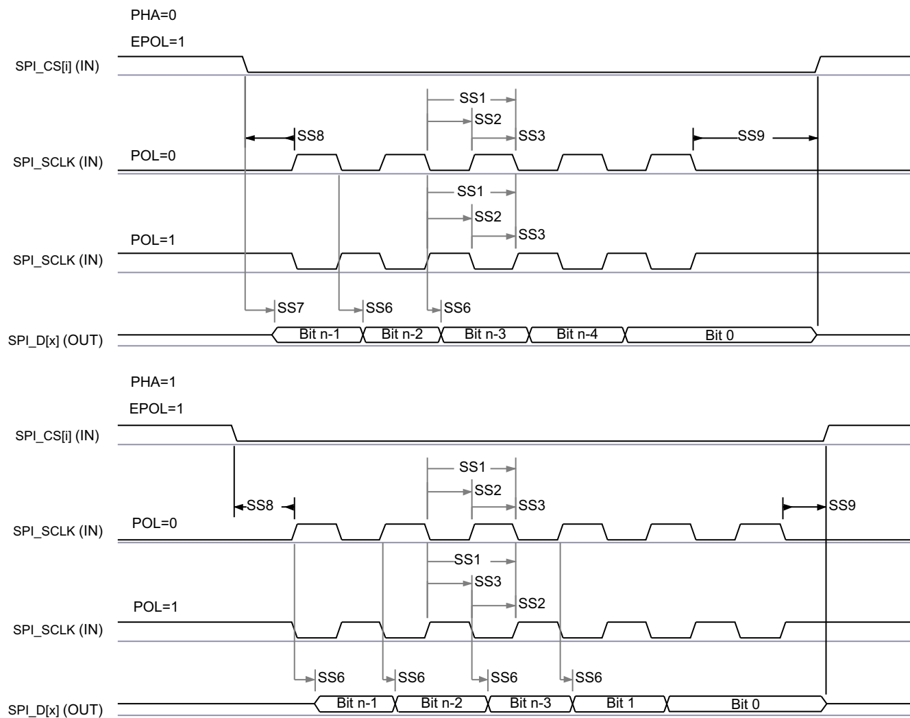
图 6-45. SPI 外设模式发送时序
