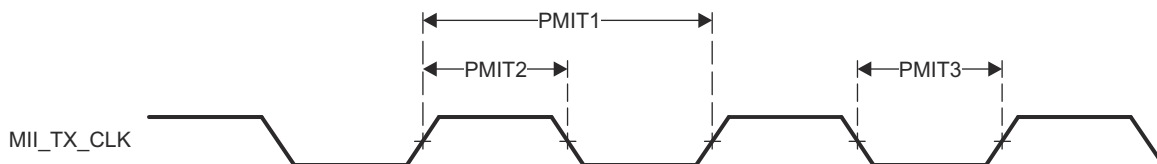
图 6-71. PRU-ICSS MII[x]_TX_CLK 时序
