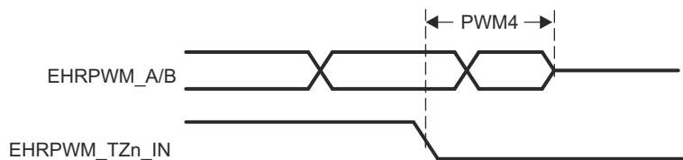
图 6-22. EHRPWM_TZn_IN 至 EHRPWM_A/B 高阻态开关特性
