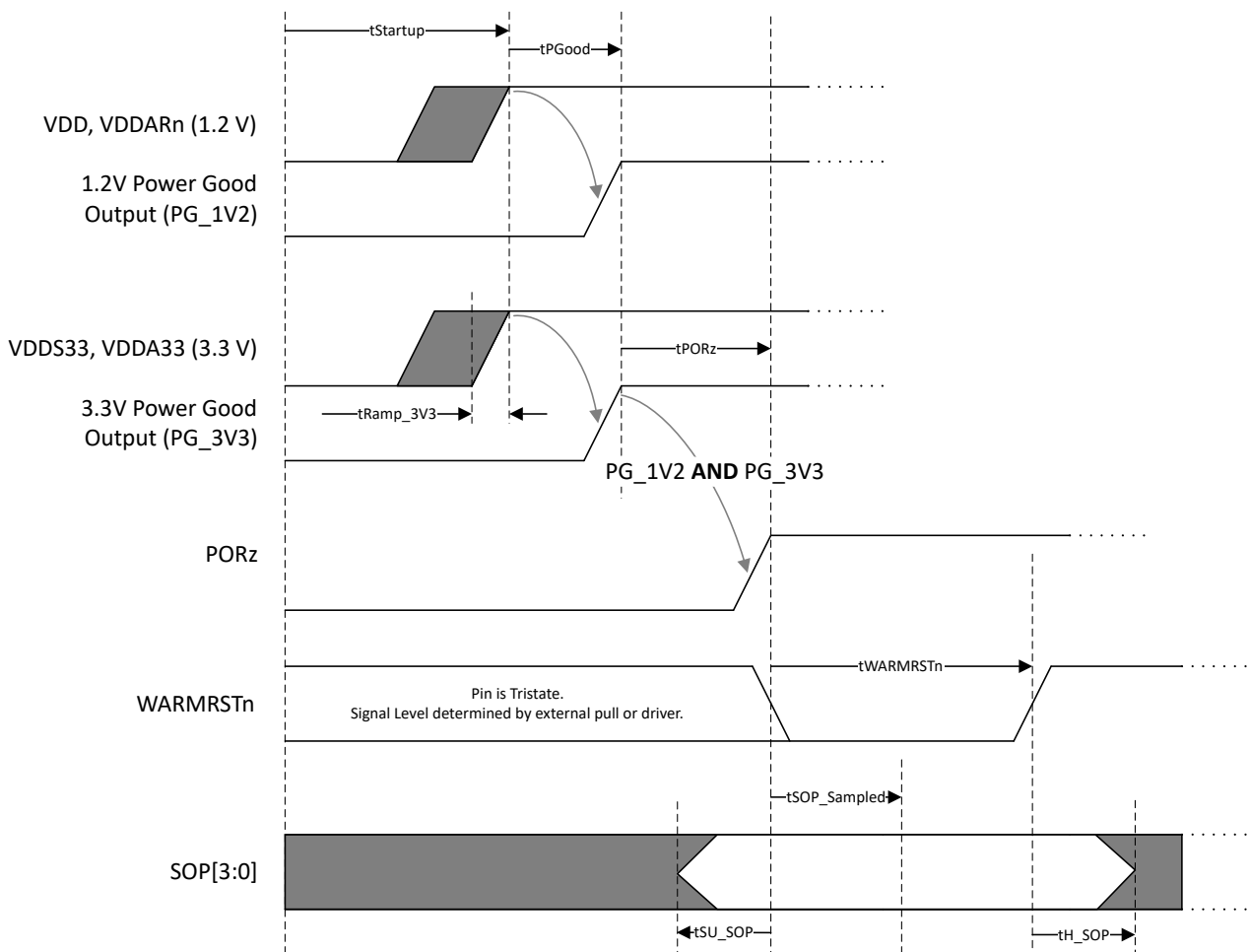
图 6-1. 加电时序
