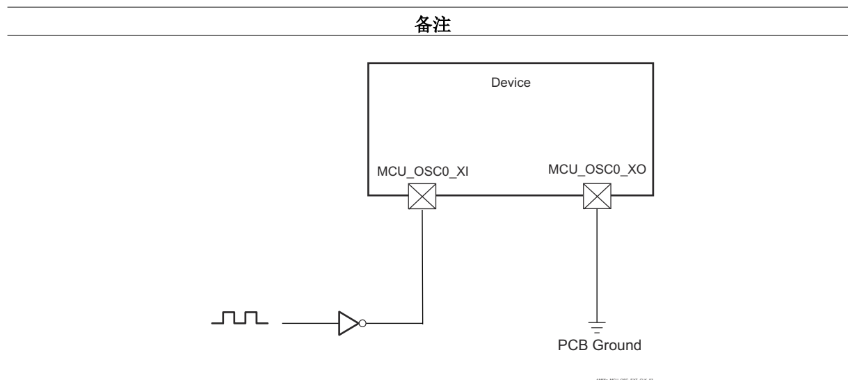
图 6-8. 1.8V LVCMOS 兼容时钟输入
