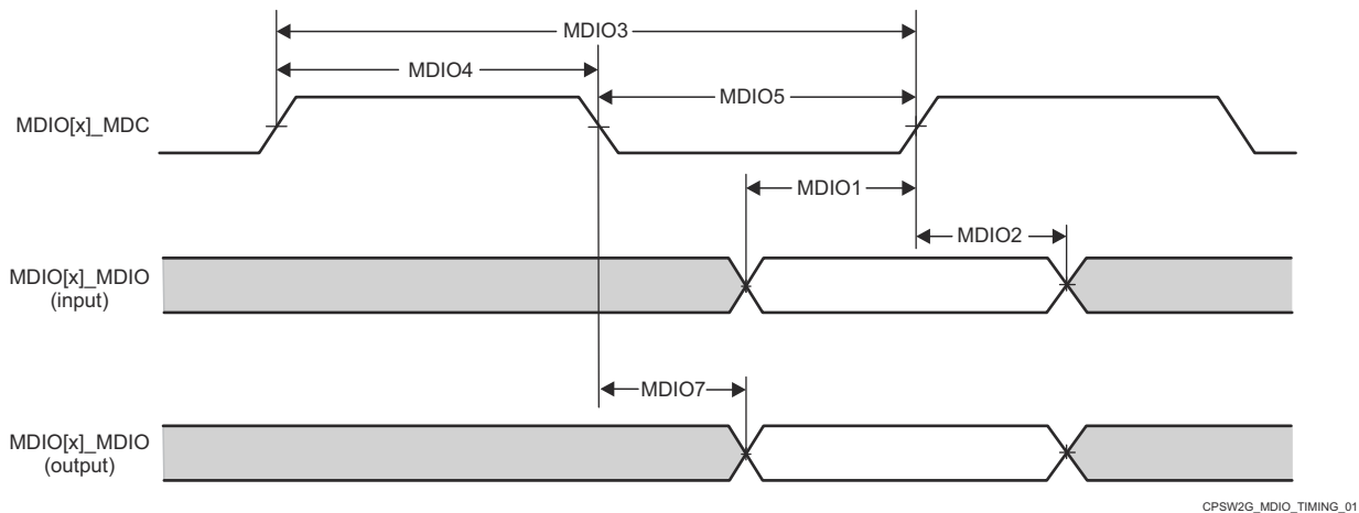
图 6-68. PRU-ICSS MDIO 时序要求和开关特性
