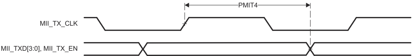
图 6-72. PRU-ICSS MII[x]_TXD[3:0]、MII[x]_TX_EN 时序
