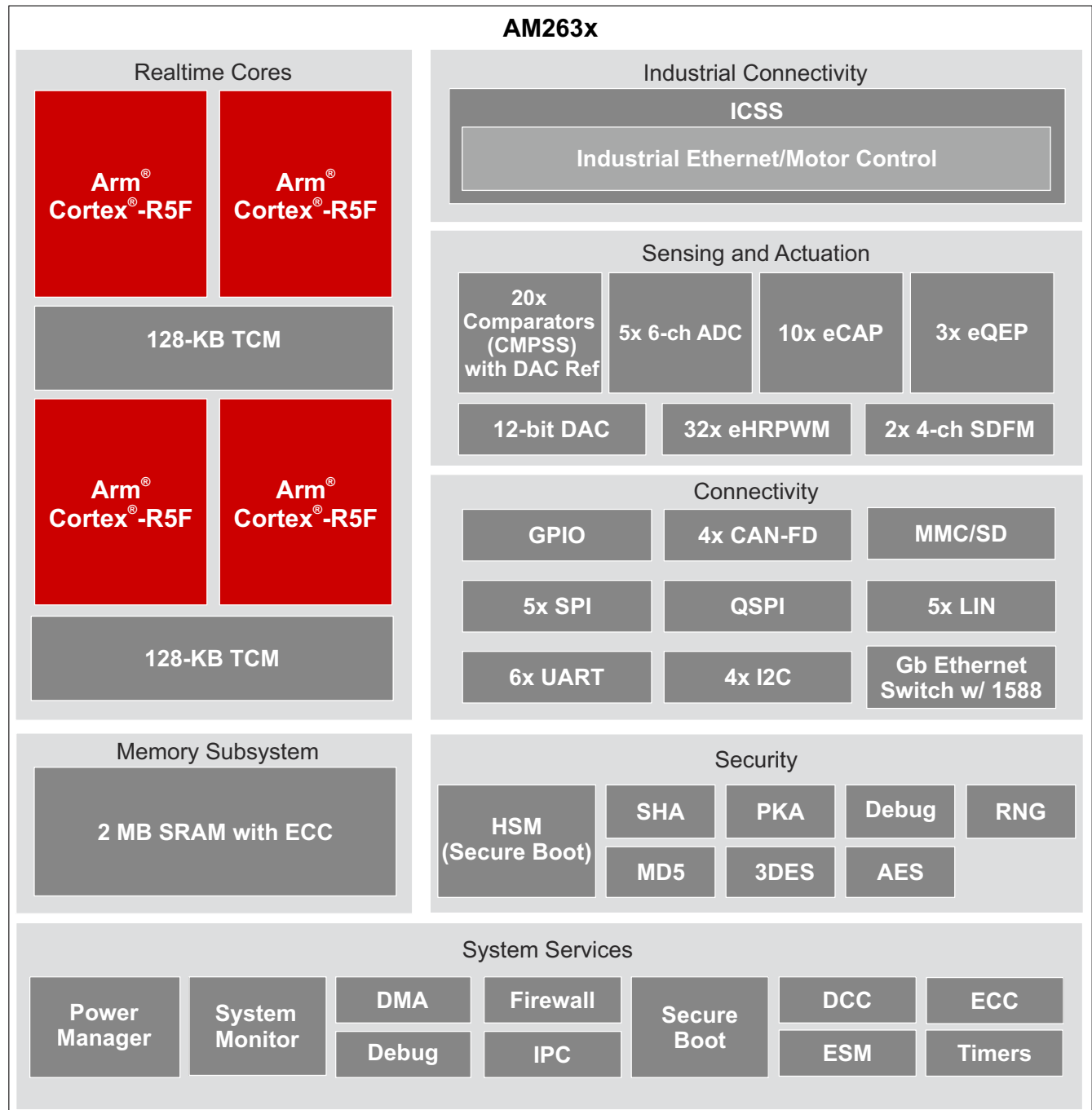
图 3-1. 功能方框图
