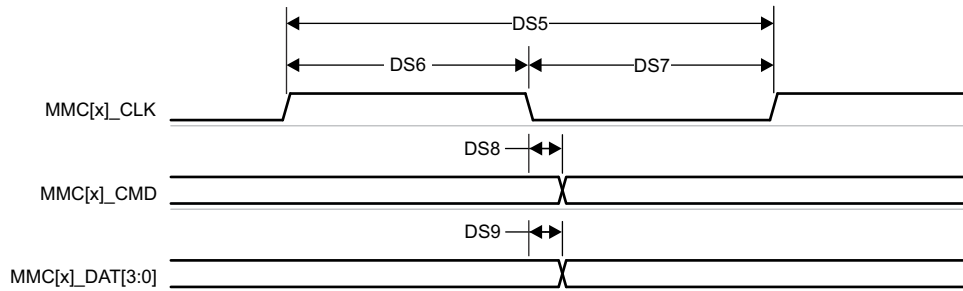
图 6-47. MMC- 默认速度 - 发送模式
