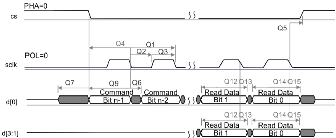
图 6-50. QSPI 时序要求
