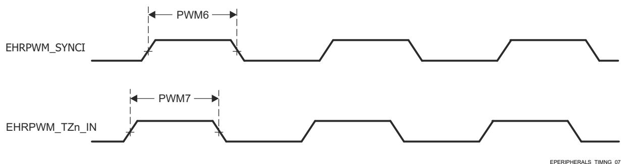
图 6-19. EPWM 时序要求
