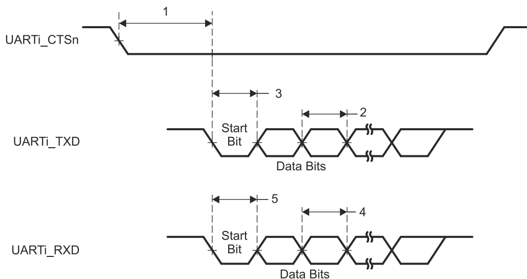
图 6-73. UART 时序要求和开关特性
