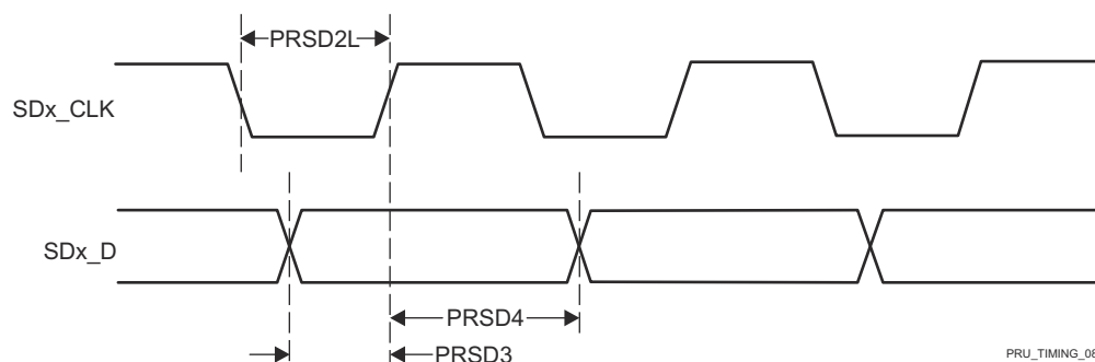
图 6-58. PRU-ICSS PRU SD_CLK 上升有效沿
