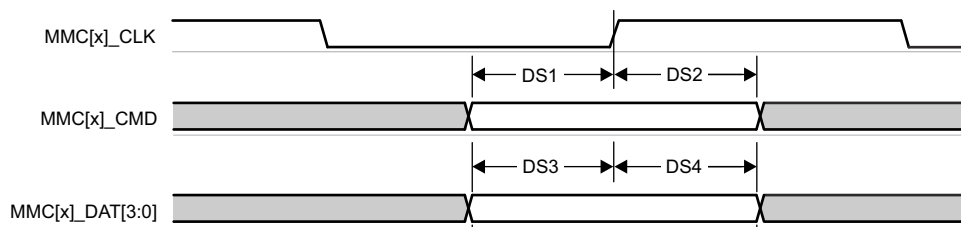
图 6-46. MMC - 默认速度 - 接收模式
