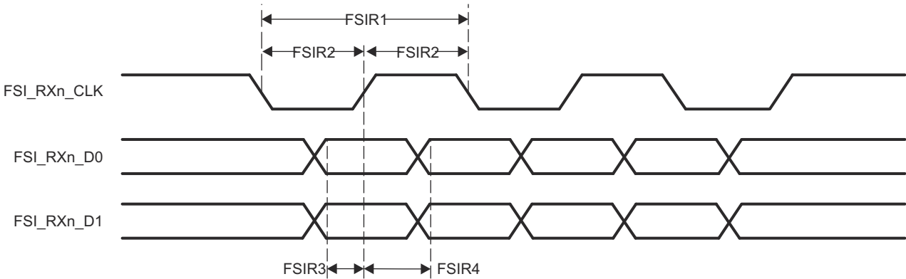
图 6-24. FSI 时序要求
