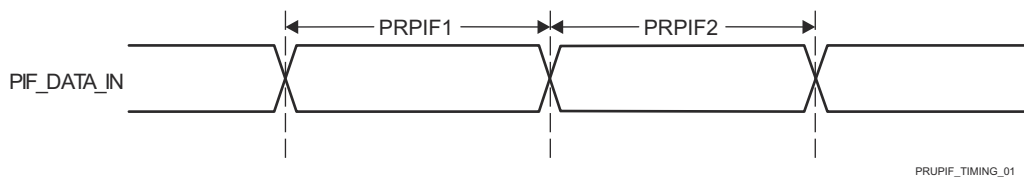
图 6-59. PRU-ICSS PRU 外设接口时序要求
