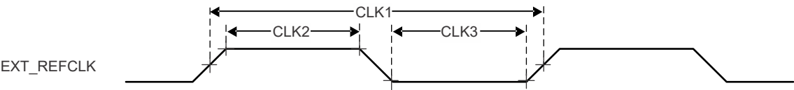
图 6-9. 时钟时序要求
