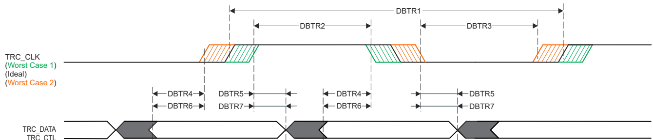
图 6-75. 布线开关特性
