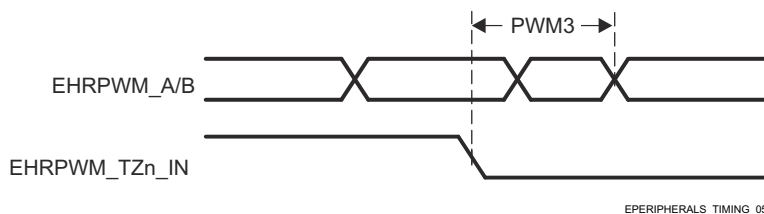
图 6-21. EHRPWM_TZn_IN 至 EHRPWM_A/B 强制开关特性
