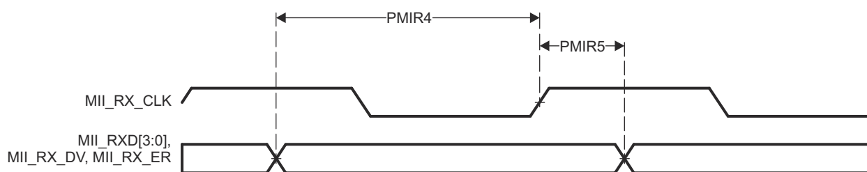
图 6-70. PRU-ICSS MII[x]_RXD[3:0]、MII[x]_RX_DV 和 MII[x]_RX_ER 时序
