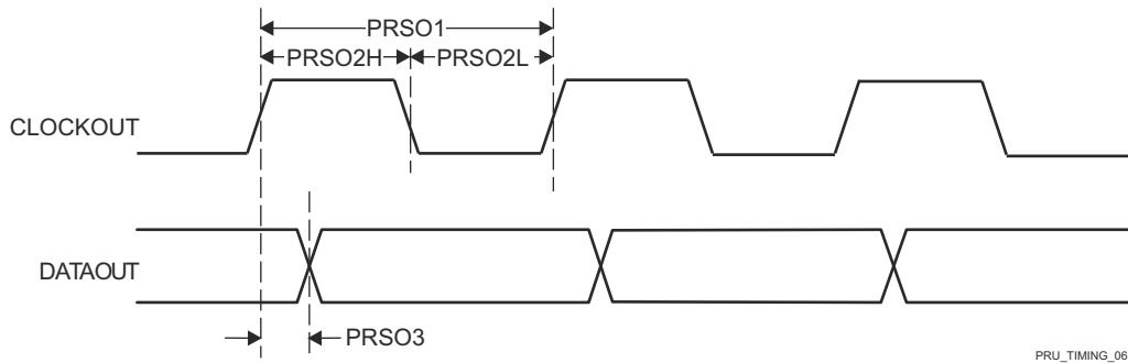
图 6-56. PRU-ICSS PRU 移出时序
