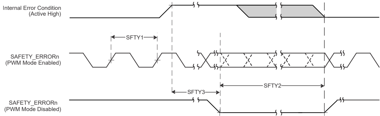
图 6-6. MCU_SAFETY_ERRORn 时序要求和开关特性
