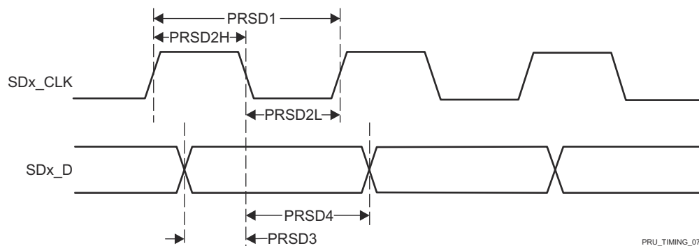
图 6-57. PRU-ICSS PRU SD_CLK 下降有效沿
