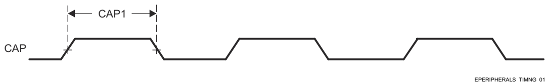
图 6-17. ECAP 时序要求
