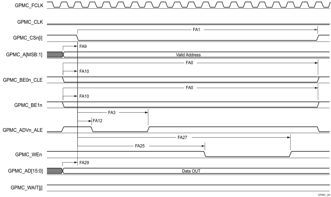
图 6-35. GPMC 和 NOR 闪存 - 异步写入 - 单字
