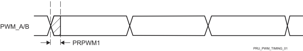
图 6-61. PRU-ICSS PWM 时序
