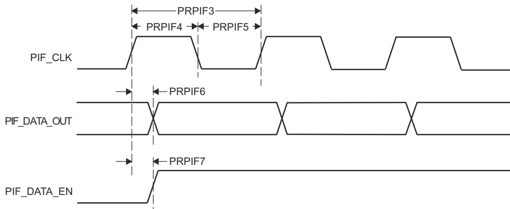
图 6-60. PRU-ICSS PRU 外设接口开关特性
