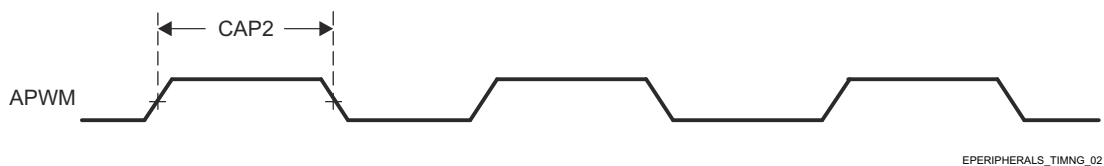
图 6-18. ECAP 开关特性
