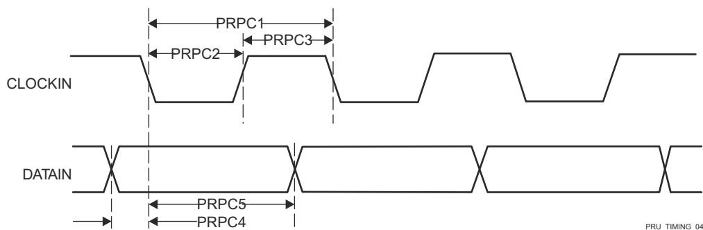
图 6-54. PRU-ICSS PRU 并行采集时序要求 - 下降沿模式
