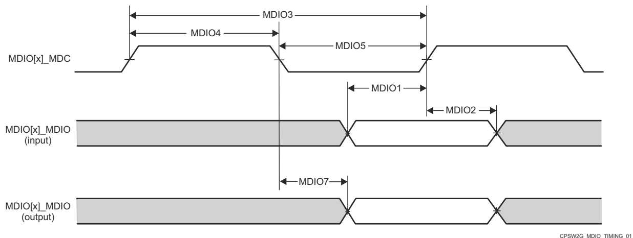
图 6-11. CPSW MDIO 时序要求和开关特性
