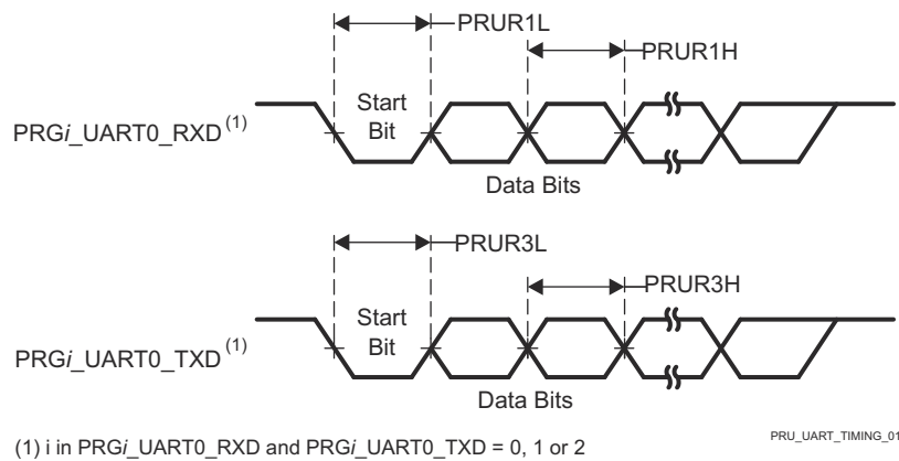
图 6-65. PRU-ICSS UART 时序要求和开关特性
