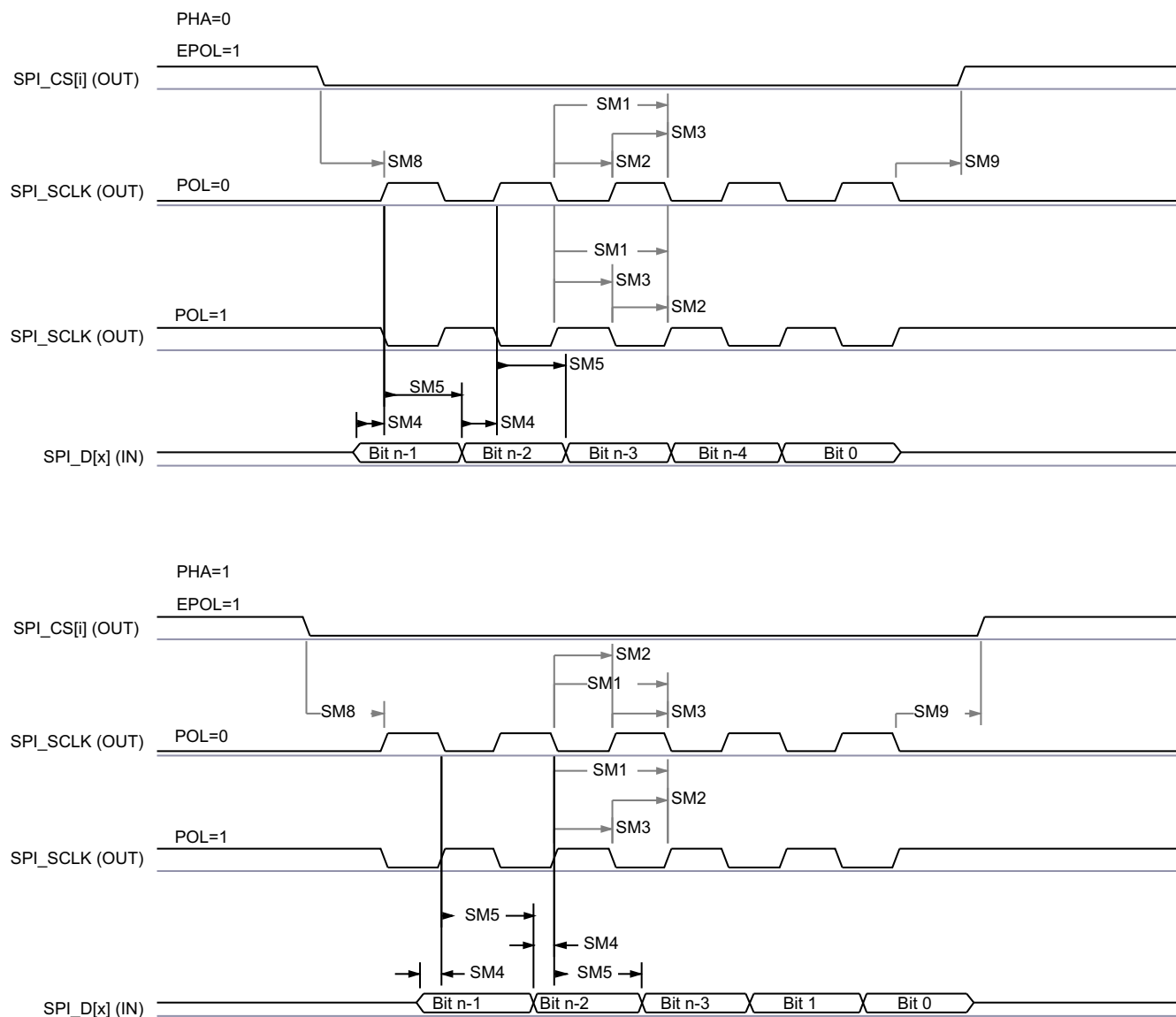
图 6-42. SPI 控制器模式接收时序
