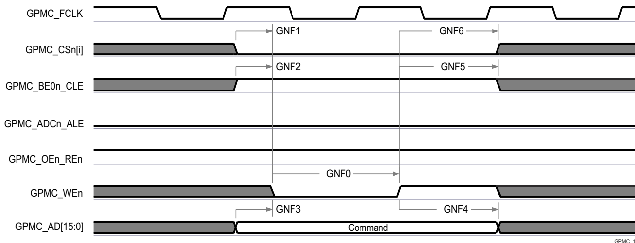
图 6-38. GPMC 和 NAND 闪存 - 命令锁存周期
