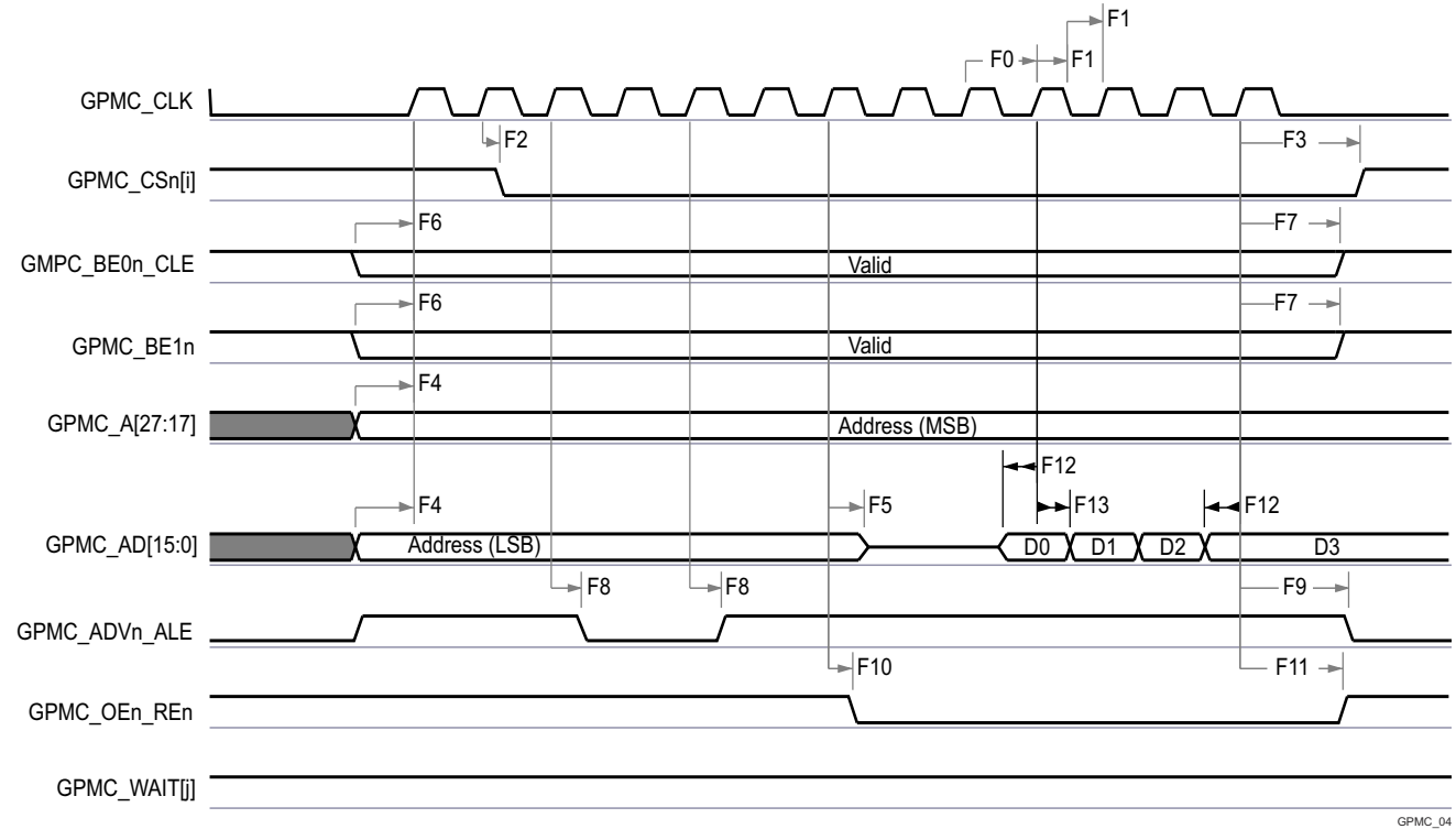
图 6-29. GPMC 和 NOR 闪存 - 同步突发写入 (GPMCFCLKDIVIDER = 0)
