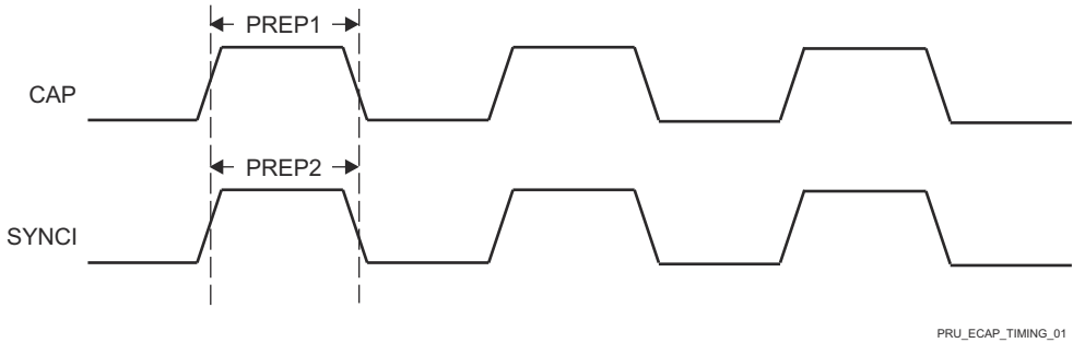
图 6-66. PRU-ICSS ECAP 时序
