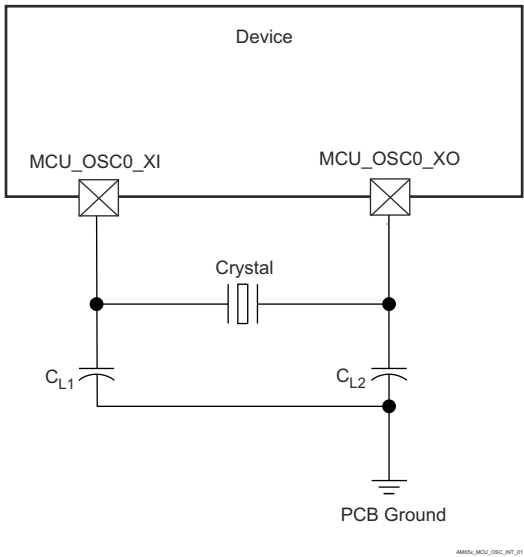
图 6-7. MCU_OSC0 晶体实现
