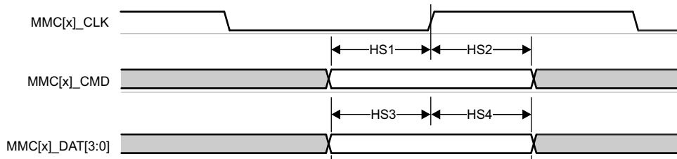
图 6-48. MMC - 高速 - 接收模式
