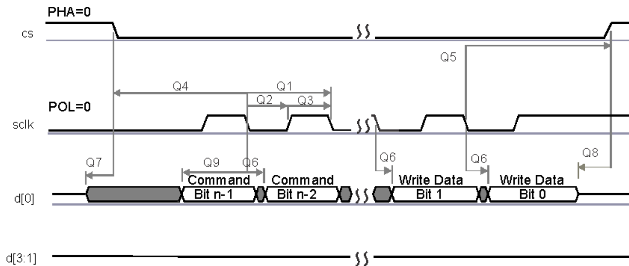
图 6-51. QSPI 开关特性
