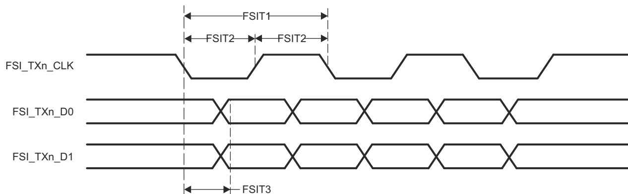
图 6-25. FSI 开关特性 - FSI 模式
