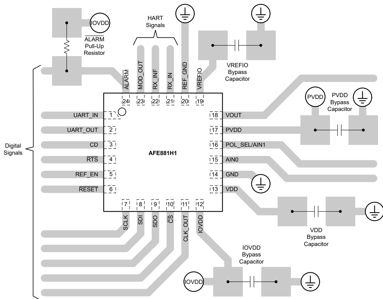
图 8-12. Layout Example
