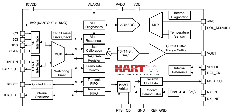
功能方框图
