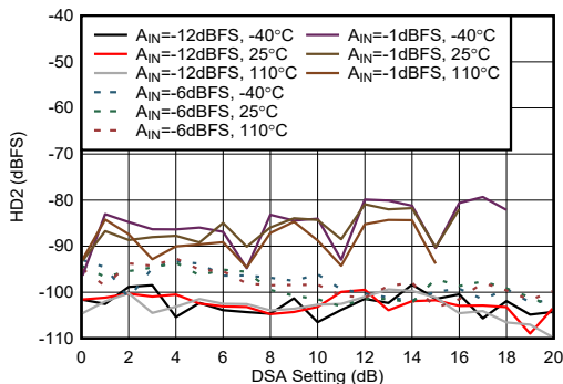
图 4-426. 8.1 GHz 条件下 RX HD2 与 DSA 设置间的关系
