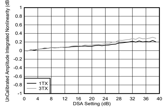
图 4-189. 8.1GHz 条件下 TX DSA 未校准振幅积分非线性
