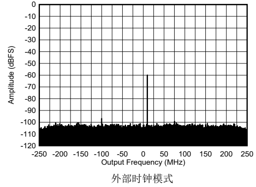
图 4-435. 8.1GHz 条件下 RX 单频输出 FFT，-60dBFS
