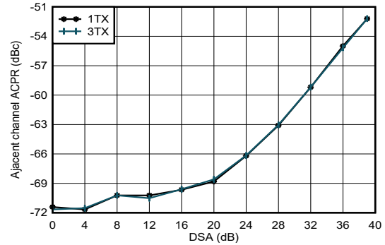
图 4-69. 1.8GHz 条件下 TX 20MHz LTE ACPR 与 DSA 间的关系
