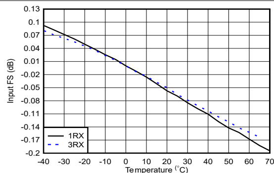
图 4-276. 800MHz 条件下 RX 输入满量程与温度和通道间的关系
