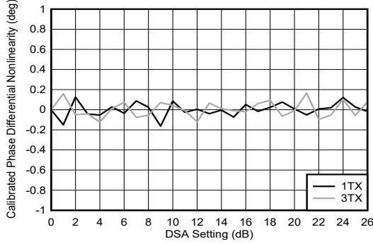
图 4-239. TX DSA 校准相位微分非线性
