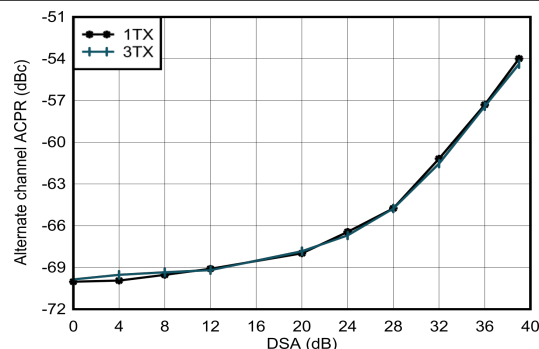
图 4-32. 0.85GHz 条件下 TX 20MHz LTE alt-ACPR 与数字电平间的关系
