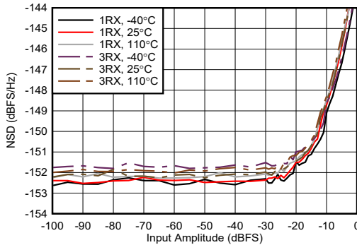
图 4-450. 9.6GHz 条件下 RX NSD 与数字振幅间的关系
