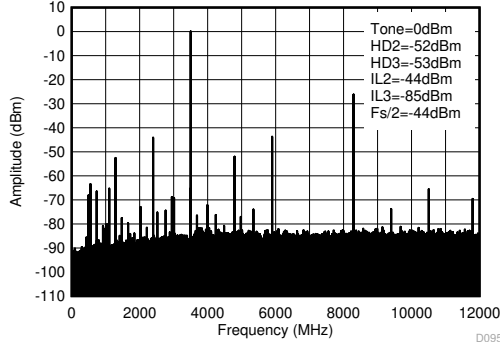
图 4-144. 3.5GHz (0 - f_{\text{DAC}} ) 条件下的 TX 单频 (-1dBFS) 输出频谱
