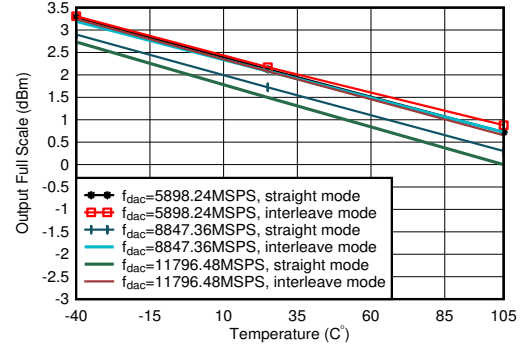
图 4-43. 1.8GHz 条件下 TX 输出功率与温度间的关系
