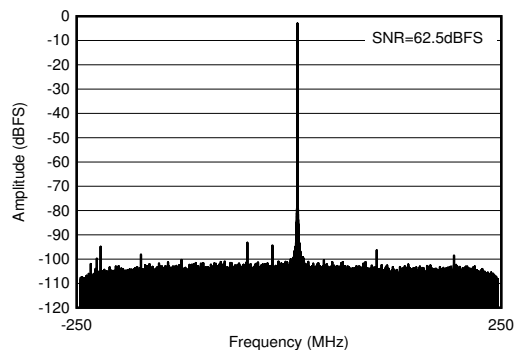
图 4-366. 2.6GHz 条件下的 RX 输出 FFT
