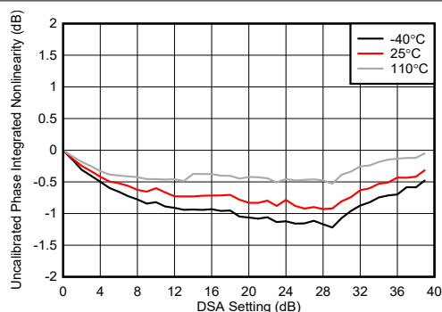
图 4-199. 8.11GHz 条件下 TX DSA 未校准相位积分非线性
