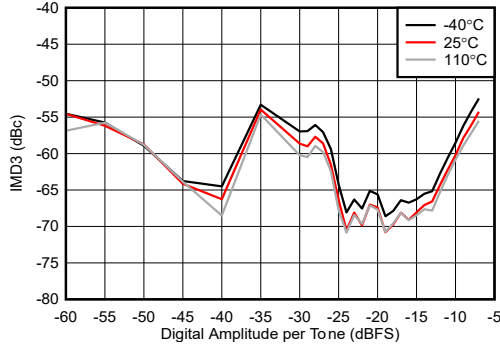
图 4-212. 8.11GHz 条件下 TX IMD3 与数字振幅间的关系
