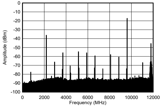
图 4-263. 9.61GHz 和 -12dBFS (宽带) 条件下 TX 单频频谱
