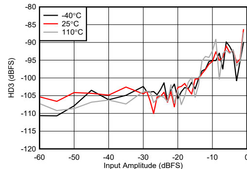
图 4-427. 8.1GHz 条件下 RX HD3 与数字振幅间的关系
