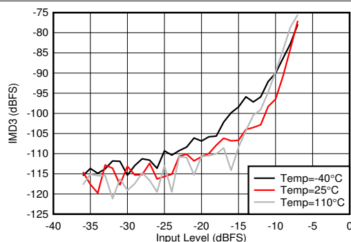
图 4-372. 2.6GHz 条件下 RX IMD3 与输入电平和温度间的关系
