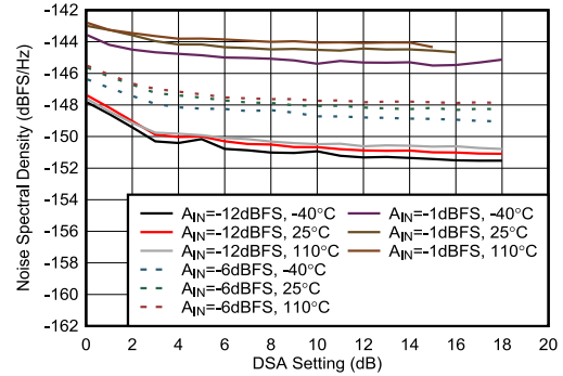
图 4-423. 8.1 GHz 条件下 RX NSD 与 DSA 设置间的关系
