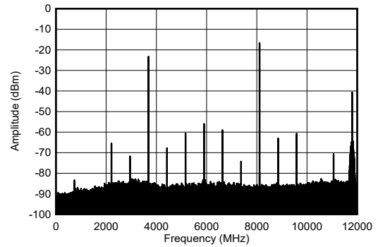
图 4-203. 8.1GHz 条件下 TX 单频输出频谱
