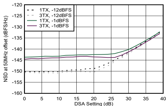
50MHz 偏移
