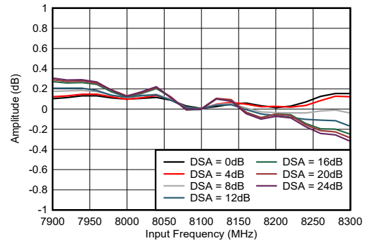
图 4-413. RX 振幅与频率和 DSA 设置间的关系
