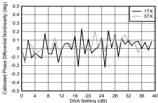
图 4-194. 8.11GHz 条件下 TX DSA 校准相位微分非线性
