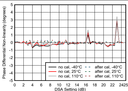
图 4-416. 8.11GHz 条件下 RX 相位微分非线性
