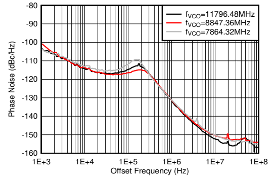
图 4-469. f_{\text{OUT}} = 2610\text{MHz} 时相位噪声与偏移频率和 f_{\text{VCO}} 间的关系
