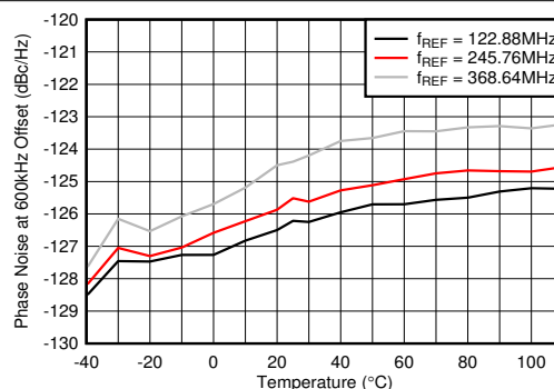
图 4-487. f_{OUT} = 2.6\text{GHz} 时 10GHz VCO 相位噪声 (600kHz 条件下) 与温度和 f_{REF} 间的关系
