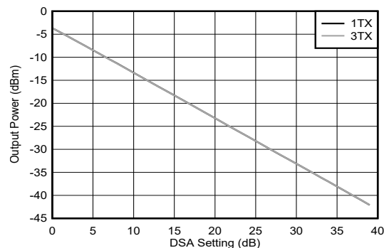
图 4-183. 8.1 GHz 条件下 TX 输出功率与 DSA 设置间的关系
