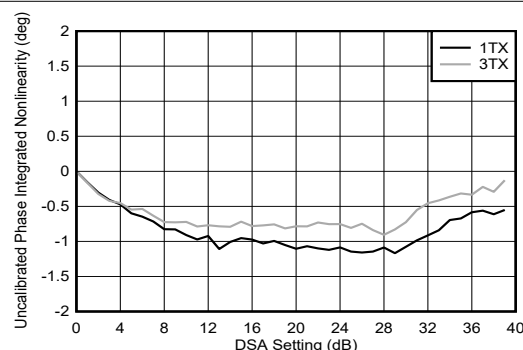
图 4-197. 8.11GHz 条件下 TX DSA 未校准相位积分非线性
