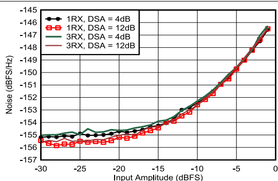
图 4-320. 1.75GHz 条件下 RX 噪声频谱密度与输入振幅和通道间的关系
