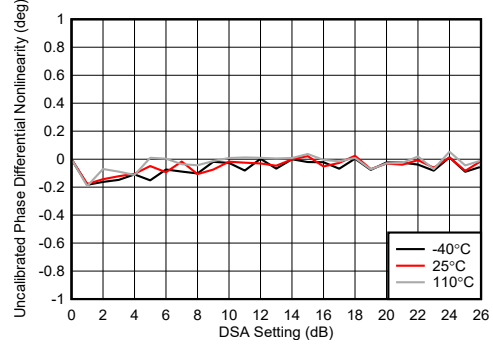
图 4-240. TX DSA 未校准相位微分非线性
