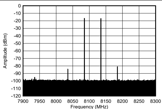
图 4-208. 8.11GHz 条件下 TX 双频输出频谱
