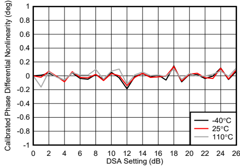
图 4-241. TX DSA 校准相位微分非线性
