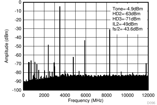
图 4-145. 3.5GHz (0 - f_{\text{DAC}} ) 条件下的 TX 单频 (-6dBFS) 输出频谱
