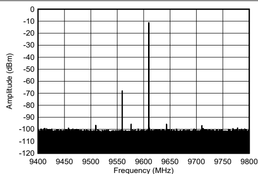
图 4-260. 9.61GHz 和 -1dBFS (1.2 GHz 带宽) 条件下 TX 单频频谱
