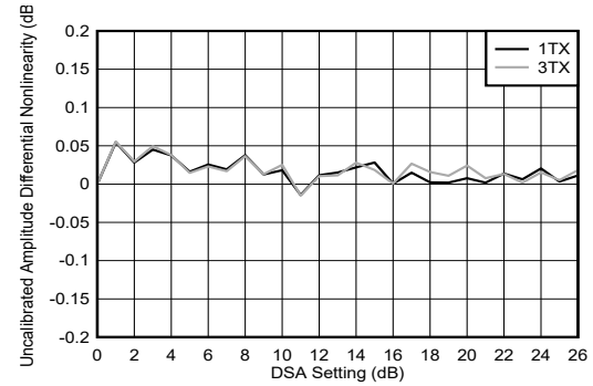
图 4-230. TX DSA 未校准振幅微分非线性
