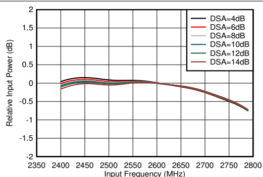
图 4-363. RX 带内增益平坦度， f_{\text{IN}} = 2600\text{MHz}
