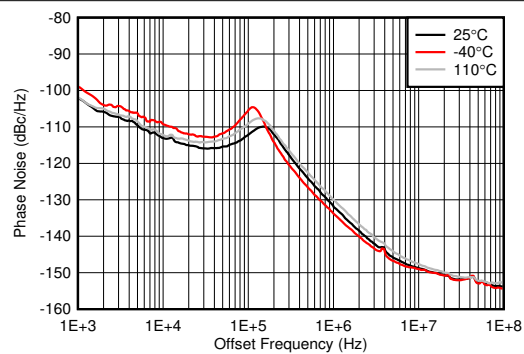
图 4-498. f_{OUT} = 1910\text{MHz} 时 8GHz VCO 相位噪声与偏移频率和温度间的关系
