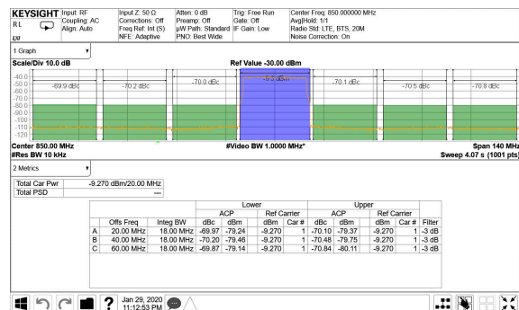
图 4-30. 0.85GHz 条件下的 TX 20MHz LTE 输出频谱
