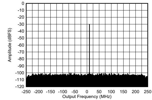
图 4-460. 9.61GHz 条件下 RX 单频输出 FFT
