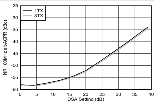
图 4-271. 9.61GHz 条件下 TX NR100MHz alt-ACPR 与 DSA 设置间的关系
