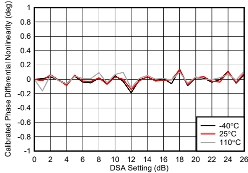
图 4-243. TX DSA 校准相位积分非线性
