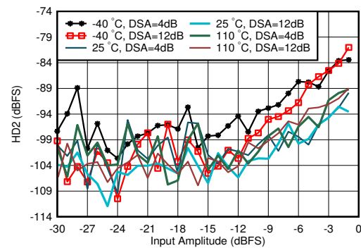
图 4-325. 1.9GHz 条件下 RX HD2 与 DSA 设置和温度间的关系
