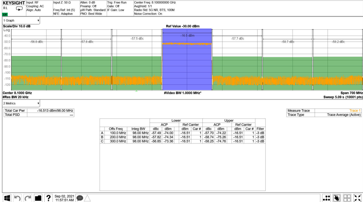
图 4-223. 8.1GHz 条件下 TX 100MHz NR 输出频谱
