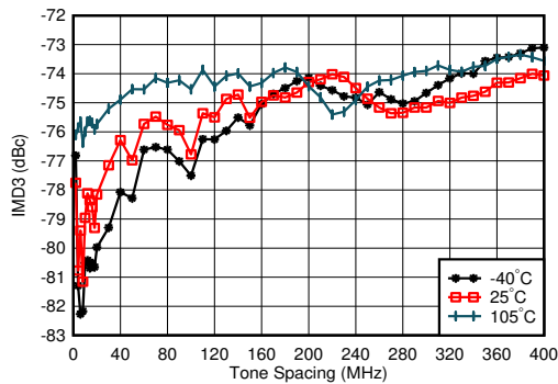
f_{\text{DAC}} = 11796.48\text{MSPS} , 直接模式, f_{\text{CENTER}} = 0.85\text{GHz} , 在 0.8GHz 条件下匹配, 单频幅度为 -13dBFS, 最差通道
