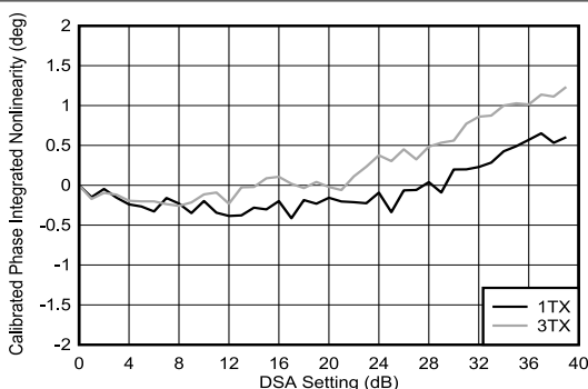
图 4-198. 8.11GHz 条件下 TX DSA 校准相位积分非线性
