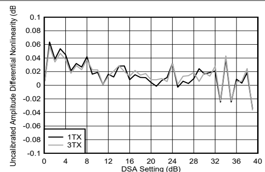
图 4-185. 8.1GHz 条件下 TX DSA 未校准振幅微分非线性
