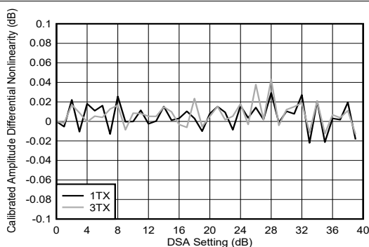
图 4-186. 8.1GHz 条件下 TX DSA 校准振幅微分非线性
