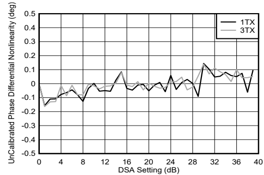
图 4-193. 8.1GHz 条件下 TX DSA 未校准相位微分非线性
