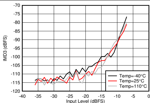
图 4-371. 2.6GHz 条件下 RX IMD3 与输入电平和温度间的关系
