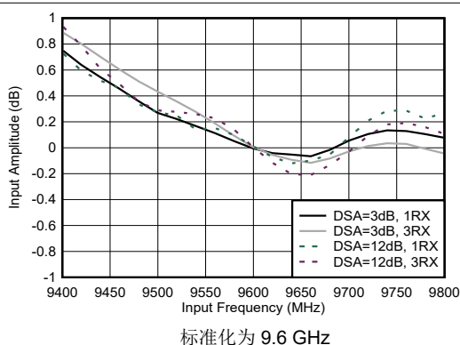
图 4-440. RX 输入振幅与频率间的关系
