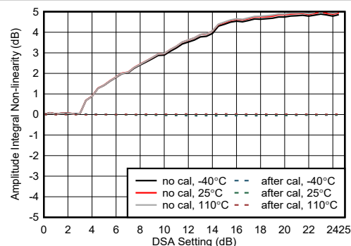
图 4-443. 9.6GHz 条件下 RX 振幅积分非线性
