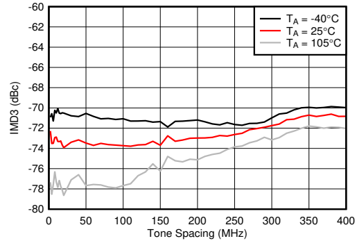
f_{\text{DAC}} = 8847.36\text{MSPS} , 直接模式, f_{\text{CENTER}} = 2.6\text{GHz} , 在 2.6GHz 条件下匹配, 单频幅度为 -13dBFS, 最差通道。
