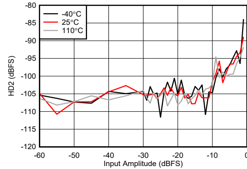
图 4-425. 8.1GHz 条件下 RX HD2 与数字振幅间的关系
