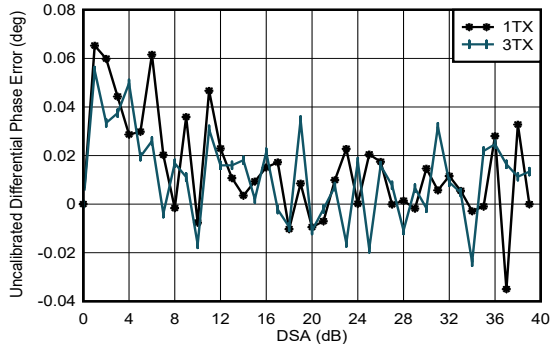
图 4-122. 3.5GHz 条件下 TX 未校准差分相位误差与 DSA 设置和通道间的关系
