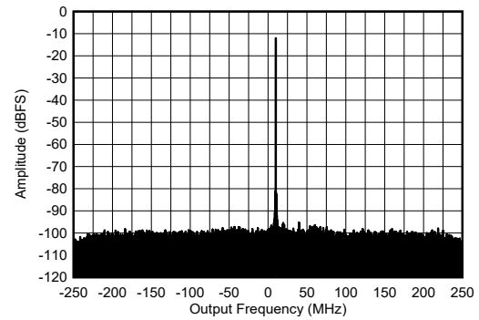
图 4-459. 9.61GHz 条件下 RX 单频输出 FFT
