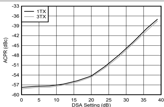
图 4-220. 8.11GHz 条件下 TX NR100MHz ACPR 与 DSA 设置间的关系
