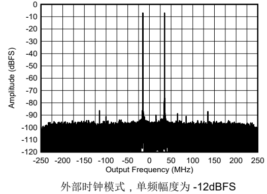
图 4-437. 8.1GHz 条件下 RX 双频输出 FFT
