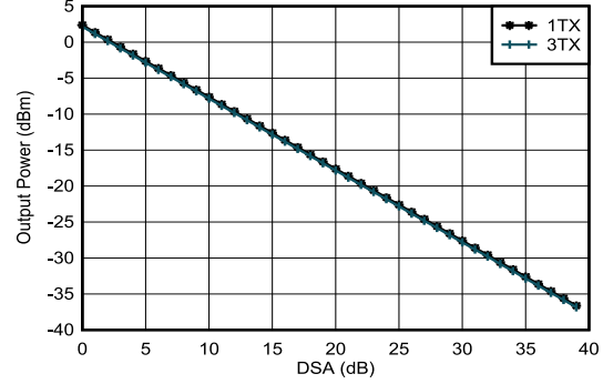
图 4-77. 2.6GHz 条件下 TX 输出功率与 DSA 设置和通道间的关系
