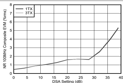
图 4-272. 9.61GHz 条件下 TX NR100MHz EVM 与 DSA 设置间的关系
