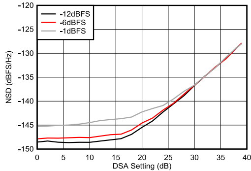
图 4-255. 9.61 GHz 条件下 TX NSD 与 DSA 设置间的关系
