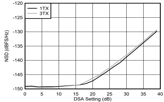
图 4-256. 9.61 GHz 条件下 TX NSD 与 DSA 设置间的关系
