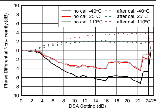
图 4-417. 8.11GHz 条件下 RX 相位微分非线性
