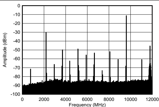
图 4-259. 9.61GHz 和 -1dBFS (宽带) 条件下 TX 单频频谱
