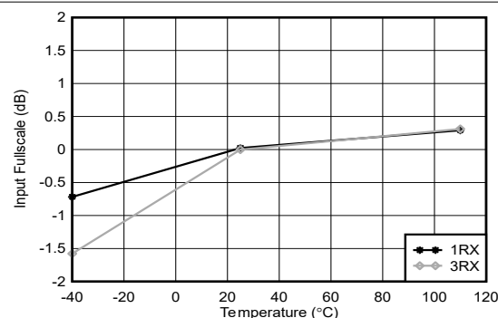
图 4-364. 2.6GHz 条件下 RX 输入满量程与温度和通道间的关系
