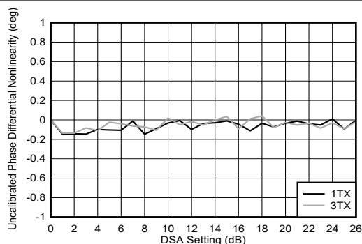
图 4-238. TX DSA 未校准相位微分非线性
