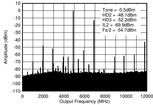
图 4-179. 4.9GHz (0 - f_{\text{DAC}} ) 条件下的 TX 单频 (-12dBFS) 输出频谱
