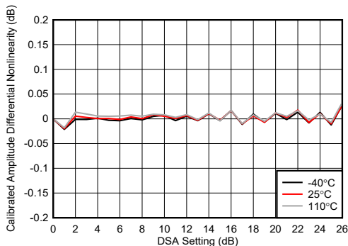
图 4-233. TX DSA 校准振幅微分非线性
