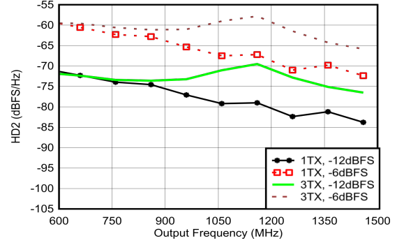
图 4-36. 0.85GHz 条件下 TX HD2 与数字振幅和输出频率间的关系
