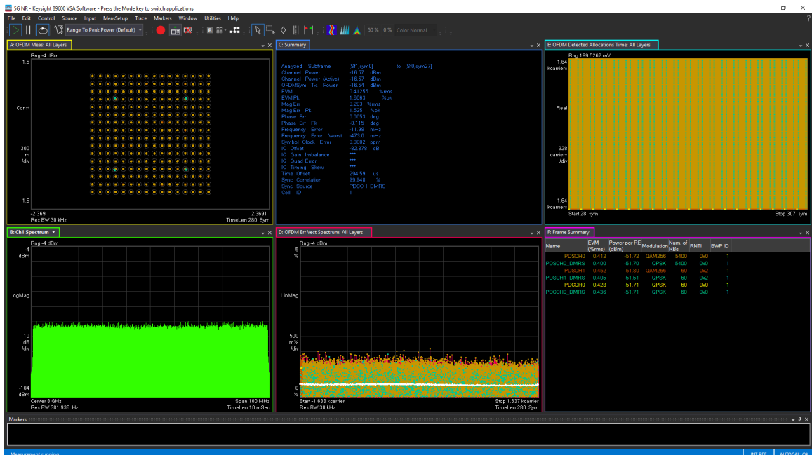
图 4-224. 8.1GHz 条件下 TX 100MHz NR EVM
