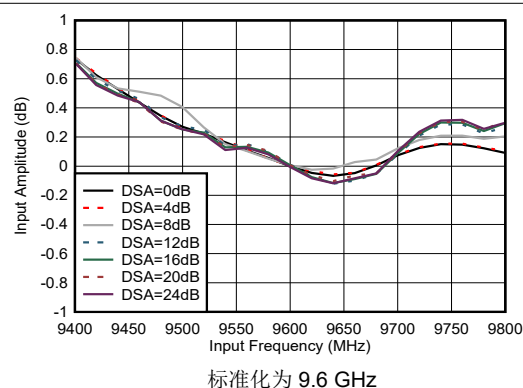
图 4-441. 9.6GHz 条件下 RX 输入振幅与频率间的关系
