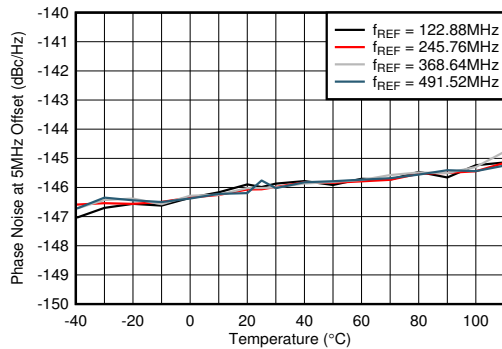
图 4-480. f_{OUT} = 2.6\text{GHz} 时 12GHz VCO 相位噪声 (5MHz 偏移条件下) 与温度和 f_{REF} 间的关系
