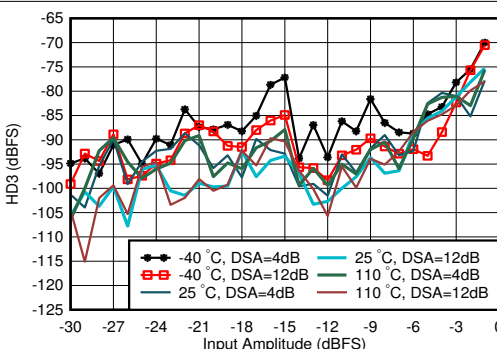
图 4-299. 0.8GHz 条件下 RX HD3 与 DSA 设置和温度间的关系
