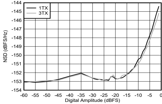
图 4-253. 9.61GHz 条件下 TX NSD 与数字振幅间的关系
