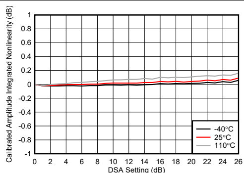
图 4-237. TX DSA 校准振幅积分非线性
