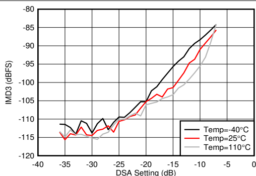
图 4-348. 3.6GHz 条件下 RX IMD3 与输入电平和温度间的关系
