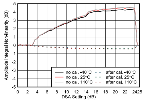
图 4-415. 8.11GHz 条件下 RX 振幅积分非线性
