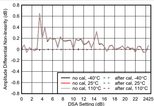
图 4-442. 9.6GHz 条件下 RX 振幅微分非线性
