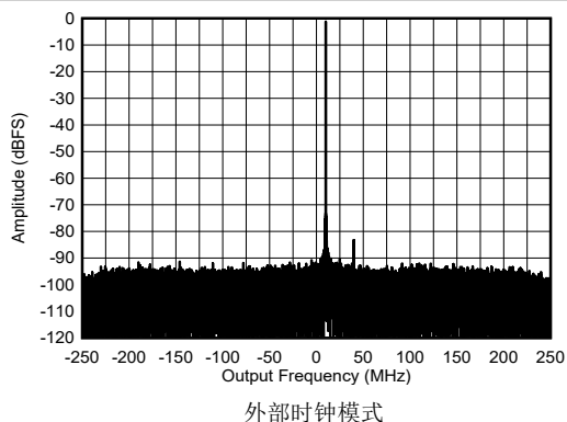
图 4-430. 8.11GHz 条件下 RX 单频输出 FFT, -1dBFS
