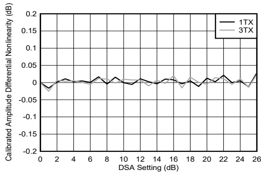
图 4-231. TX DSA 校准振幅微分非线性
