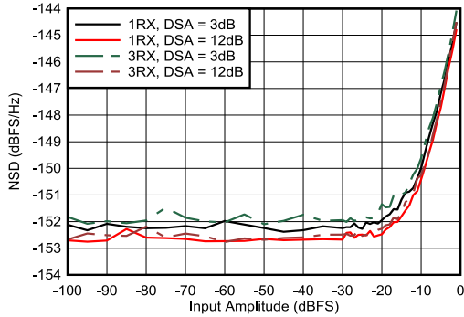
图 4-422. 8.1GHz 条件下 RX NSD 与数字振幅间的关系
