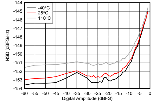
图 4-254. 9.61GHz 条件下 TX NSD 与数字振幅间的关系
