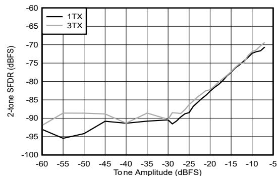
图 4-258. 9.61GHz 条件下 TX 双频 SFDR 与数字振幅间的关系
