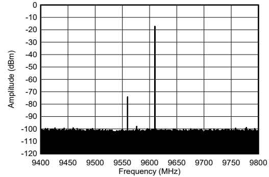
图 4-264. 9.61GHz 和 -12dBFS (1.2GHz 带宽) 条件下 TX 单频频谱
