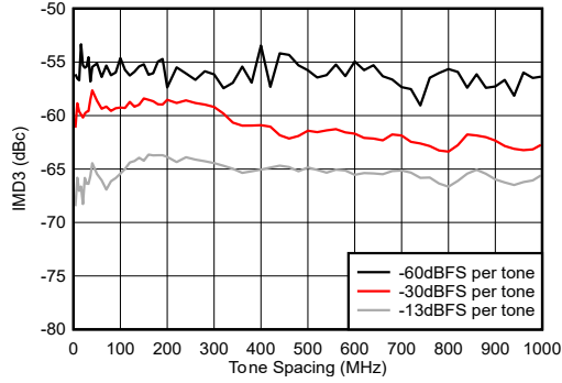
图 4-251. 9.61GHz 条件下 TX IMD3 与频率间隔间的关系
