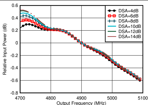
图 4-383. RX 带内增益平坦度， f_{\text{IN}} = 4900\text{MHz}
