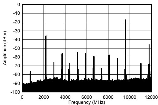
图 4-265. 9.61GHz 和 -7dBFS (宽带) 条件下 TX 双频频谱
