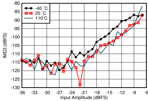
图 4-399. 4.9GHz 条件下 RX IMD3 与输入电平和温度间的关系
