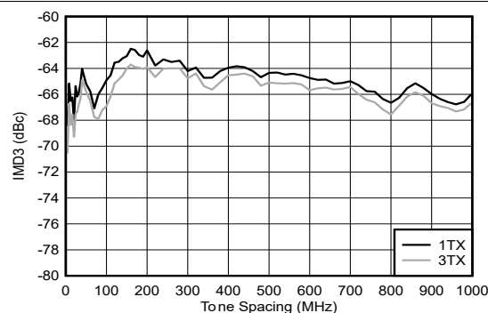
图 4-250. 9.61GHz 条件下 TX IMD3 与频率间隔间的关系
