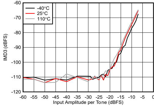
图 4-446. 9.6GHz 条件下 RX IMD3 与数字振幅间的关系
