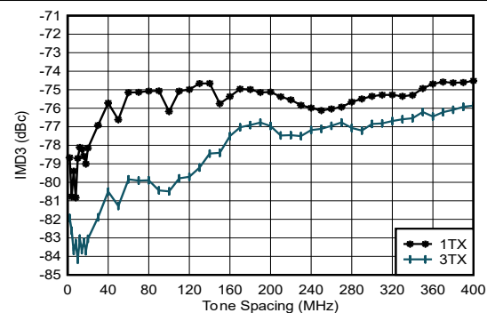
图 4-20. 0.85GHz 条件下 TX IMD3 与频率间隔和通道间的关系
