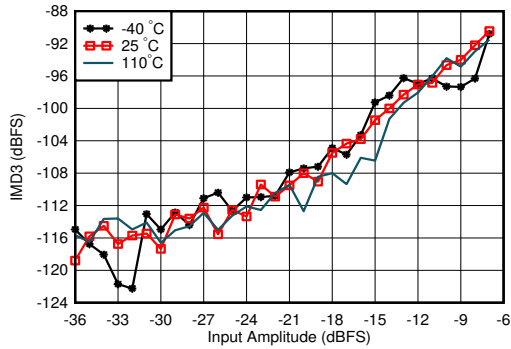
图 4-322. 1.75GHz 条件下 RX IMD3 与输入电平和温度间的关系
