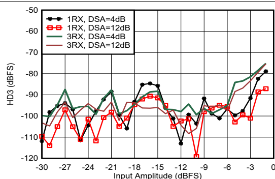
图 4-328. 1.9GHz 条件下 RX HD3 与 DSA 设置和通道间的关系
