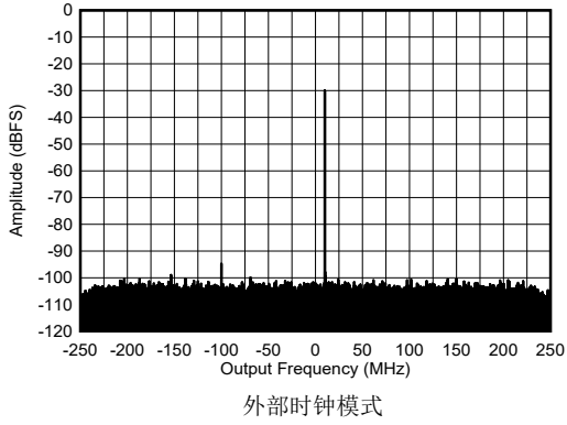
图 4-434. 8.1GHz 条件下 RX 单频输出 FFT，-30dBFS
