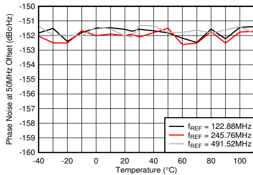
图 4-492. f_{OUT} = 2.6\text{GHz} 时 10GHz VCO 相位噪声 (50MHz 条件下) 与温度和 f_{REF} 间的关系
