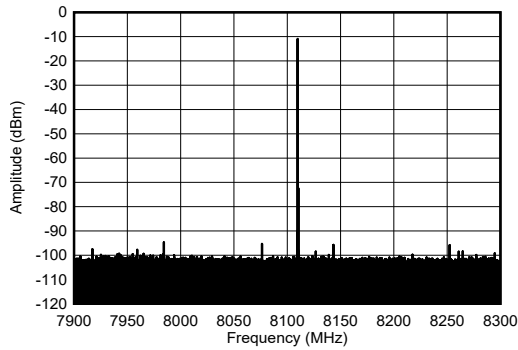
图 4-202. 8.1GHz 条件下 TX 单频输出频谱
