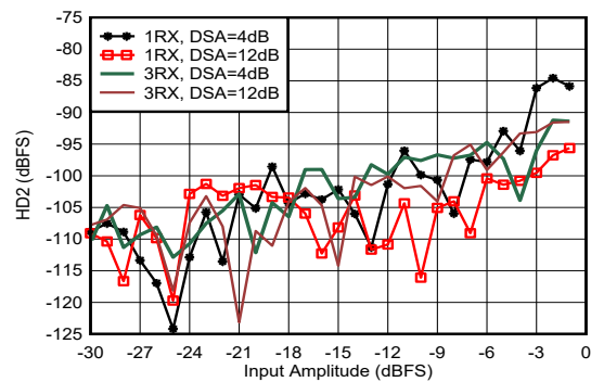
图 4-324. 1.9GHz 条件下 RX HD2 与 DSA 设置和通道间的关系
