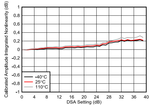
图 4-192. 8.1GHz 条件下 TX DSA 校准振幅积分非线性
