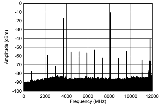
图 4-201. 8.1GHz 条件下 TX 单频输出频谱
