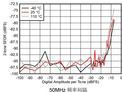
图 4-429. 8.11GHz 条件下 RX 双频 SFDR 与数字振幅间的关系
