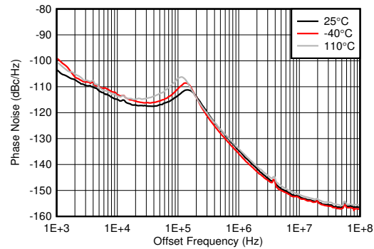
图 4-468. 12GHz 条件下 PLL 和外部时钟的相位噪声与偏移频率间的关系
