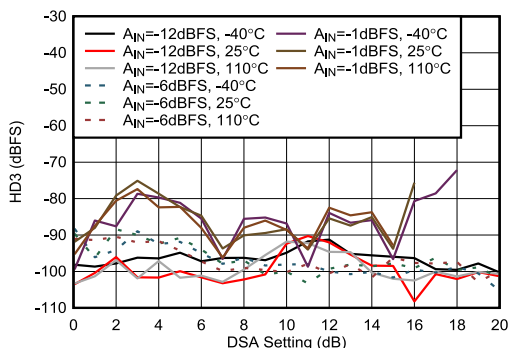
图 4-428. 8.11 GHz 条件下 RX HD3 与 DSA 设置间的关系
