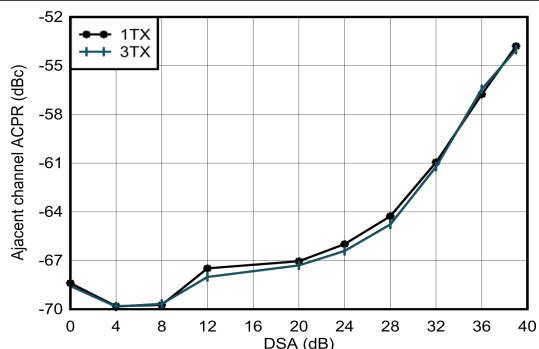
图 4-31. 0.85GHz 条件下 TX 20MHz LTE ACPR 与数字电平间的关系
