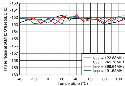
图 4-481. f_{OUT} = 2.6\text{GHz} 时 12GHz VCO 相位噪声 (50MHz 偏移条件下) 与温度和 f_{REF} 间的关系
