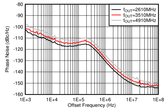
图 4-483. 25°C 条件下 10GHz VCO 相位噪声与偏移频率和 f_{OUT} 间的关系
