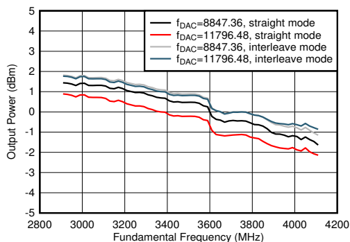
图 4-116. TX 输出功率与频率间的关系
