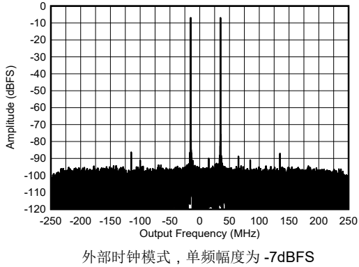
图 4-436. 8.1GHz 条件下 RX 双频输出 FFT
