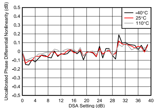
图 4-195. 8.11GHz 条件下 TX DSA 未校准相位微分非线性
