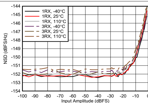
图 4-421. 8.11GHz 条件下 RX NSD 与数字振幅间的关系
