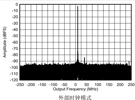
图 4-431. 8.11GHz 条件下 RX 单频输出 FFT, -3dBFS
