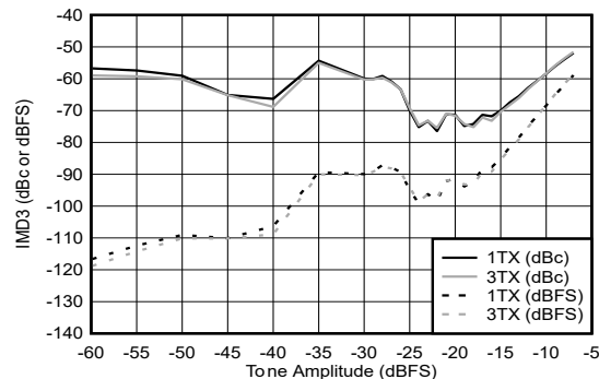
图 4-246. 9.61GHz 条件下 TX IMD3 与数字振幅间的关系
