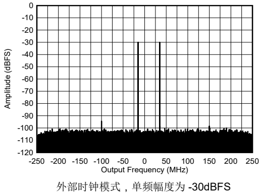
图 4-438. 8.1GHz 条件下 RX 双频输出 FFT
