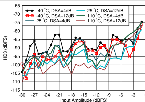
图 4-329. 1.9GHz 条件下 RX HD3 与 DSA 设置和温度间的关系
