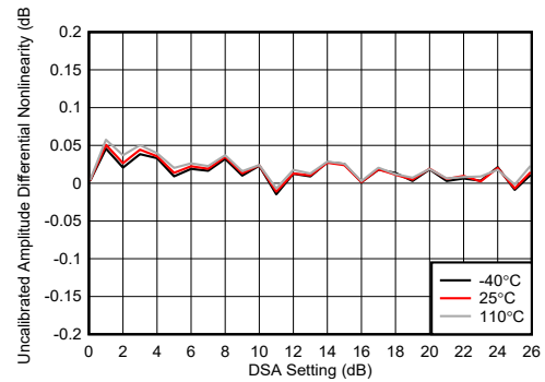
图 4-232. TX DSA 未校准振幅微分非线性
