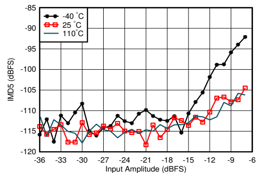
图 4-294. 0.8GHz 条件下 Rx IMD5 与输入电平和温度间的关系
