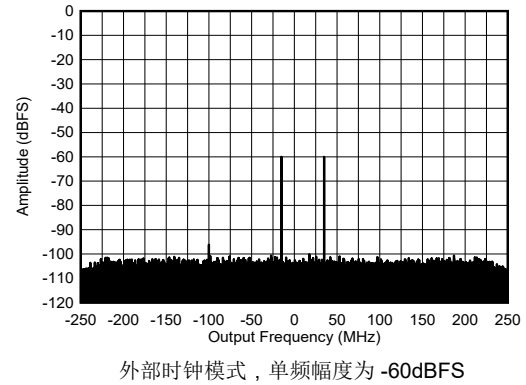
图 4-439. 8.1GHz 条件下 RX 双频输出 FFT
