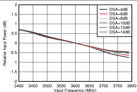
图 4-336. RX 带内增益平坦度， f_{\text{IN}} = 3600\text{MHz}
