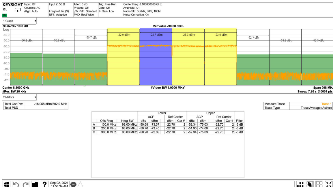
图 4-225. 8.1GHz 条件下 TX 4x100MHz NR 输出频谱
