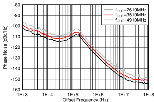
图 4-494. 25°C 条件下 9GHz VCO 相位噪声与偏移频率和 f_{OUT} 间的关系
