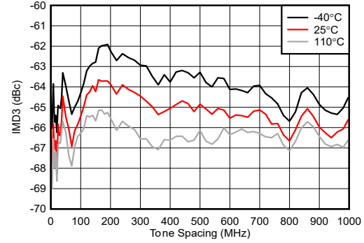
图 4-252. 9.61GHz 条件下 TX IMD3 与频率间隔间的关系
