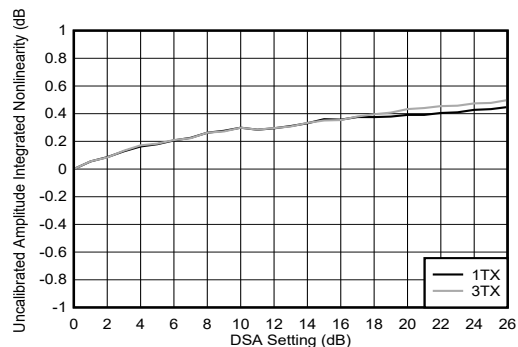
图 4-234. TX DSA 未校准振幅积分非线性
