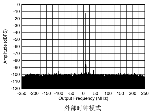
图 4-433. 8.11GHz 条件下 RX 单频输出 FFT, -12dBFS
