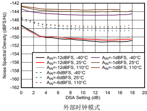
图 4-424. 8.1 GHz 条件下 RX NSD 与 DSA 设置间的关系
