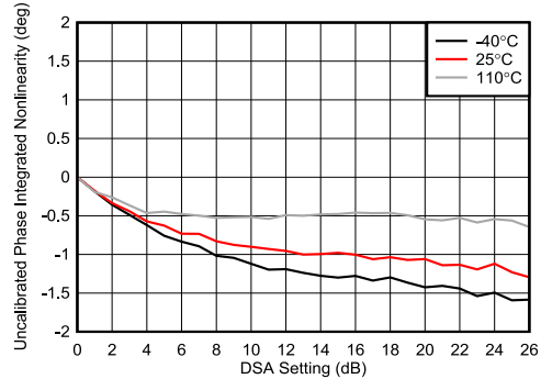
图 4-244. TX DSA 未校准相位积分非线性
