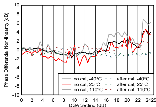
图 4-445. 9.6GHz 条件下 RX 相位微分非线性
