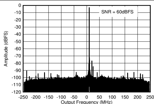
图 4-394. 4.9GHz 条件下的 RX 输出 FFT
