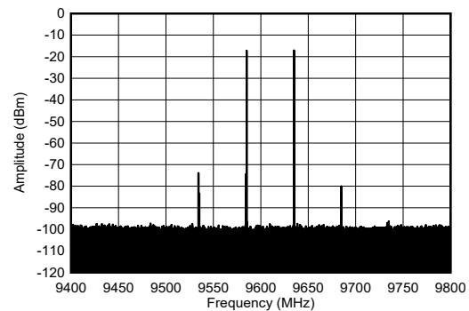
图 4-266. 9.61GHz 和 -7dBFS (1.2 GHz 带宽) 条件下 TX 双频频谱
