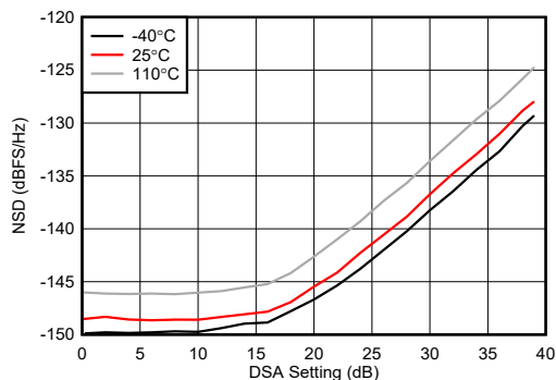
图 4-257. 9.61 GHz 条件下 TX NSD 与 DSA 设置间的关系
