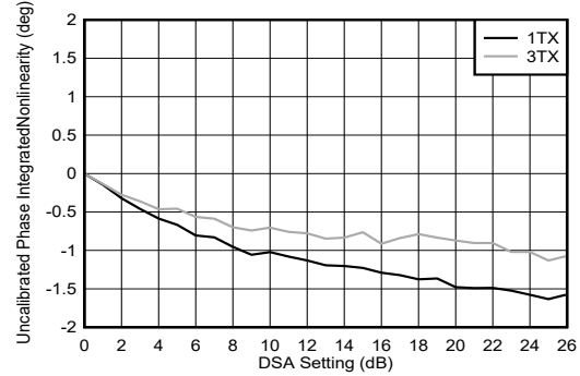
图 4-242. TX DSA 未校准相位积分非线性
