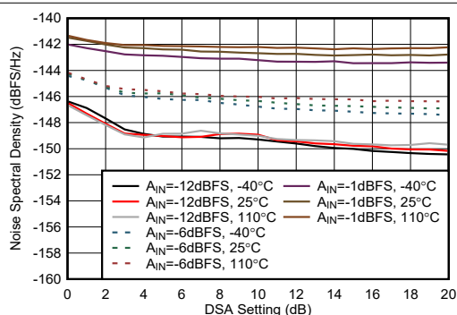
图 4-452. 9.6 GHz 条件下 RX NSD 与 DSA 设置间的关系
