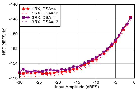
图 4-369. 2.6GHz 条件下 RX 噪声频谱密度与输入振幅和通道间的关系
