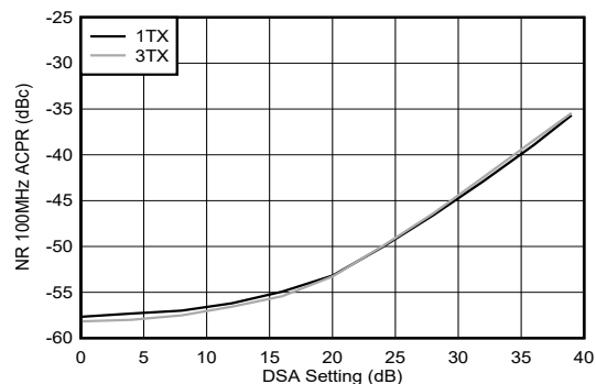
图 4-270. 9.61GHz 条件下 TX NR100MHz ACPR 与 DSA 设置间的关系
