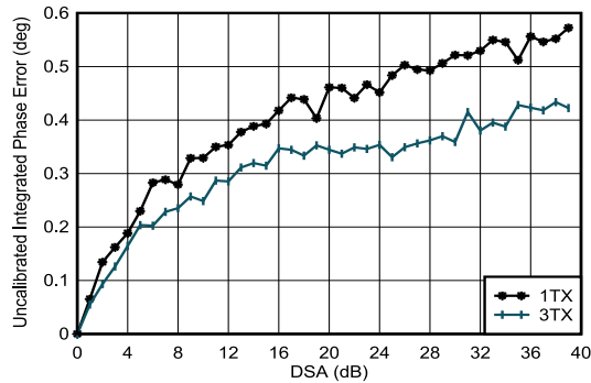
图 4-124. 3.5GHz 条件下 TX 未校准积分相位误差与 DSA 设置和通道间的关系
