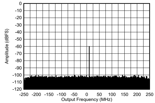
图 4-461. 9.61GHz 条件下 RX 单频输出 FFT
