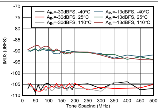
图 4-420. 8.11 GHz 条件下 RX IMD3 与频率间隔间的关系
