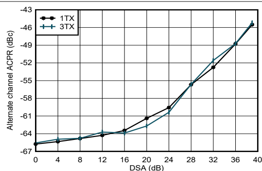
图 4-221. 8.11GHz 条件下 TX NR100MHz alt-ACPR 与 DSA 设置间的关系
