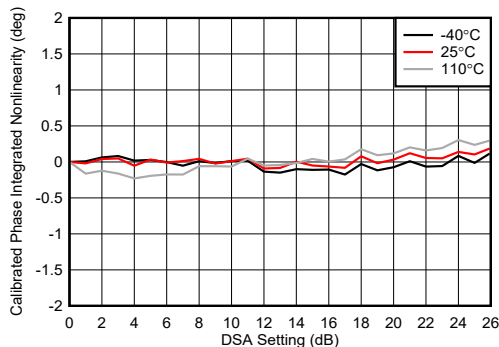
图 4-245. TX DSA 校准振幅积分非线性
