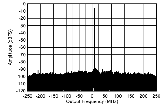
图 4-458. 9.61GHz 条件下 RX 单频输出 FFT
