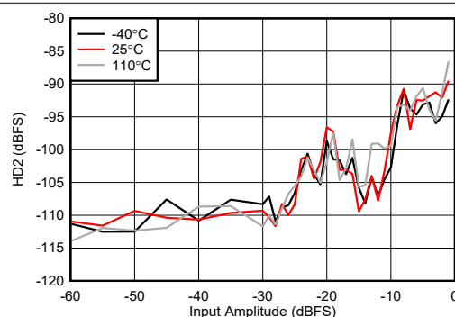
图 4-453. 9.6GHz 条件下 RX HD2 与数字电平间的关系
