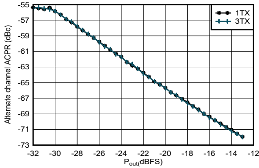
图 4-68. 1.8425GHz 条件下 TX 20MHz LTE alt-ACPR 与数字电平间的关系
