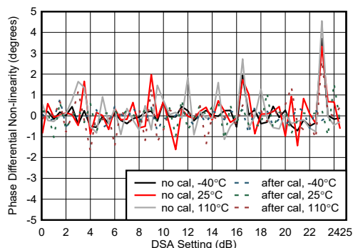
图 4-444. 9.6GHz 条件下 RX 相位微分非线性
