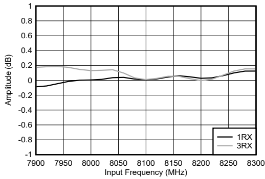
图 4-412. RX 振幅与频率和通道间的关系
