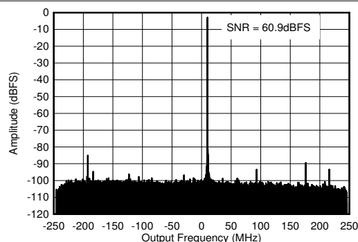
图 4-317. 1.75GHz 条件下的 RX 输出 FFT
