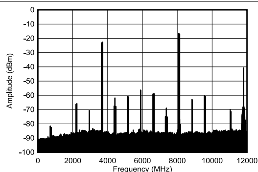
图 4-207. 8.11GHz 条件下 TX 双频输出频谱
