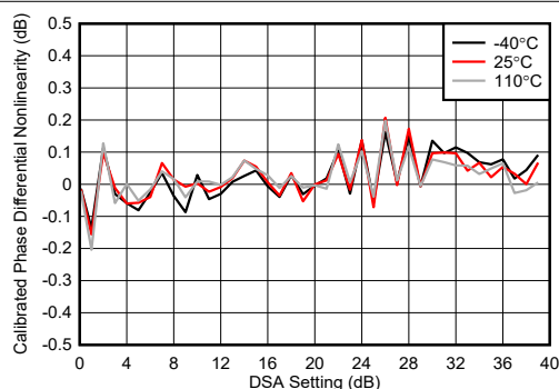
图 4-196. 8.11GHz 条件下 TX DSA 校准相位微分非线性
