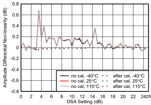
图 4-414. 8.11GHz 条件下 RX 振幅微分非线性
