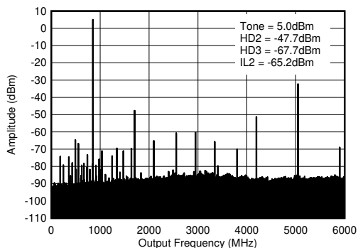
图 4-41. 0.85GHz ( 0-f_{\text{DAC}} ) 条件下的 TX 单频 ( -1\text{dBFS} ) 输出频谱
