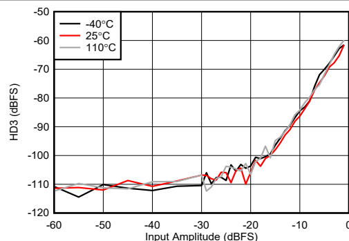
图 4-455. 9.6GHz 条件下 RX HD3 与数字电平间的关系
