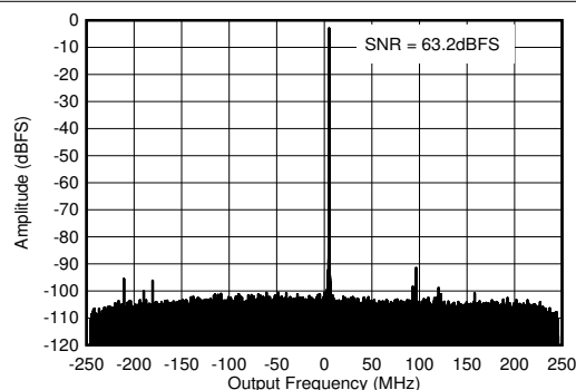
图 4-286. 0.8GHz 条件下的 RX 输出 FFT
