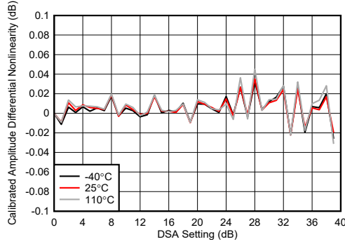
图 4-188. 8.1GHz 条件下 TX DSA 校准振幅微分非线性
