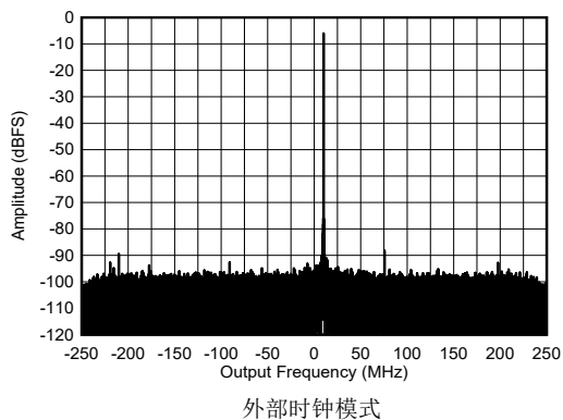
图 4-432. 8.11GHz 条件下 RX 单频输出 FFT, -6dBFS
