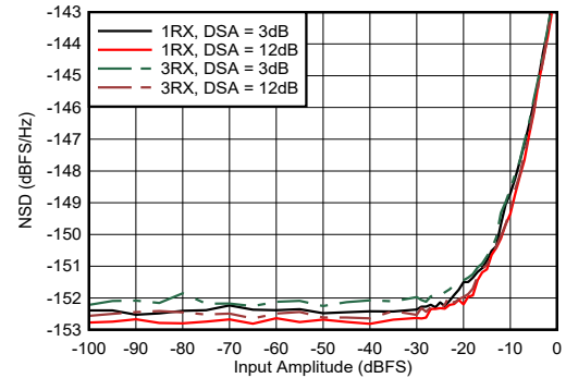
图 4-451. 9.6GHz 条件下 RX NSD 与数字振幅间的关系
