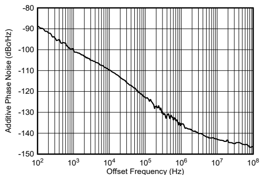
图 4-269. 9.61GHz 条件下 TX 附加相位噪声与偏移频率间的关系
