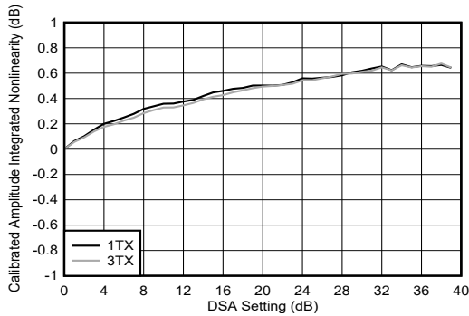
图 4-190. 8.1GHz 条件下 TX DSA 校准振幅积分非线性
