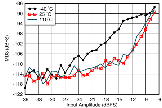
图 4-292. 0.8GHz 条件下 RX IMD3 与输入电平和温度间的关系
