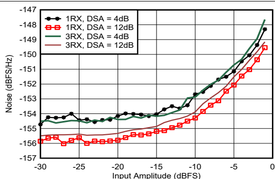
图 4-289. 0.8GHz 条件下 RX 噪声频谱密度与输入振幅和通道间的关系
