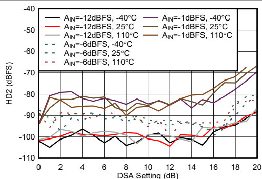
图 4-454. 9.6 GHz 条件下 RX HD2 与 DSA 设置间的关系
