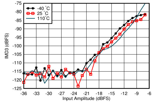
图 4-400. 4.9GHz 条件下 RX IMD3 与输入电平和温度间的关系
