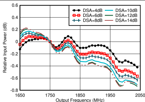
图 4-306. RX 带内增益平坦度， f_{\text{IN}} = 1750\text{MHz}
