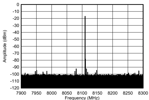
图 4-206. 8.11GHz 条件下 TX 单频输出频谱
