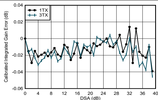
图 4-119. 3.5GHz 条件下 TX 校准差分增益误差与 DSA 设置和通道间的关系
