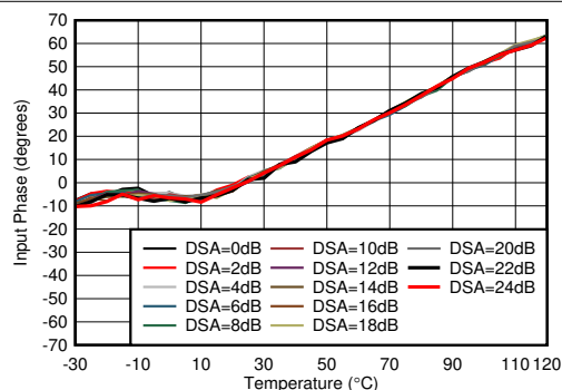
图 4-337. 3.6GHz 条件下 RX 输入相位与温度间的关系
