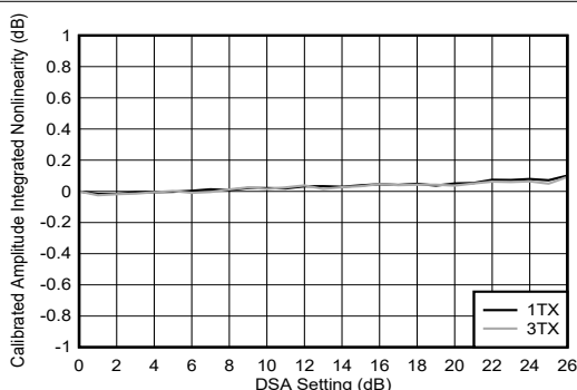
图 4-235. TX DSA 校准振幅积分非线性
