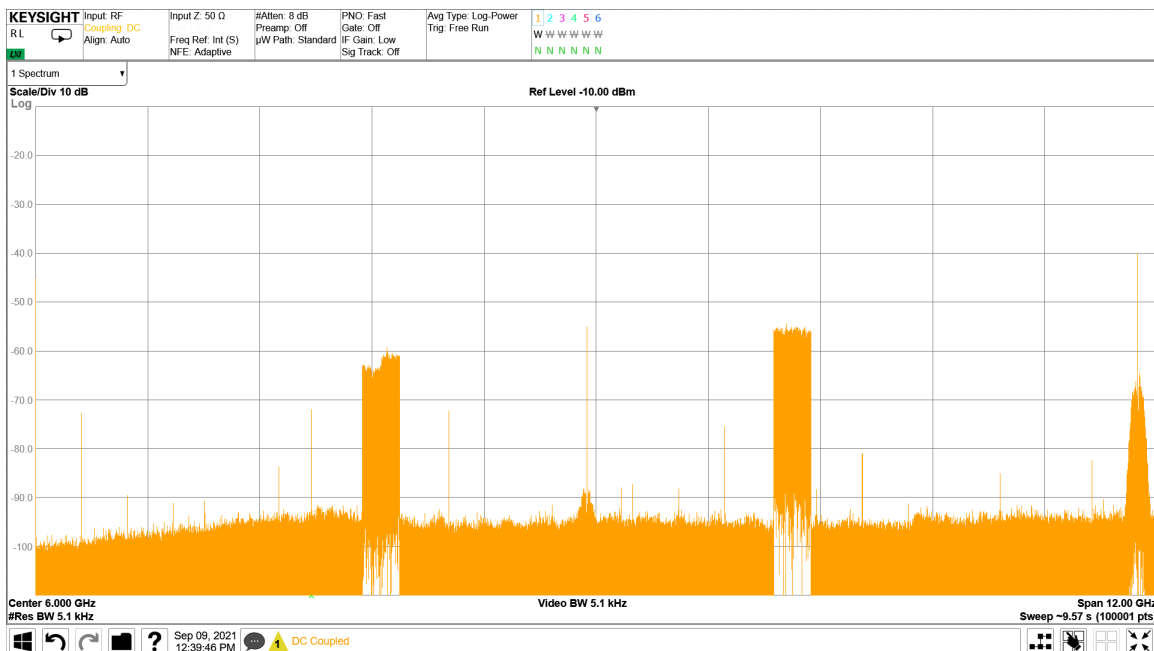
图 4-226. 8.1GHz 条件下 TX 4x100MHz NR 输出频谱
