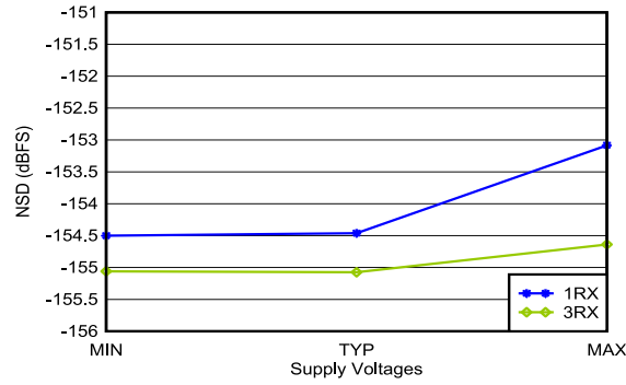
图 4-411. 4.9GHz 条件下 RX 噪声频谱密度与电源和通道间的关系
