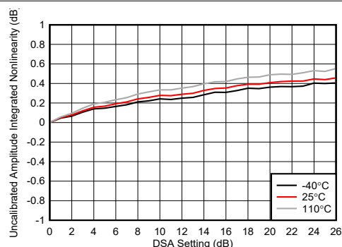
图 4-236. TX DSA 未校准振幅积分非线性
