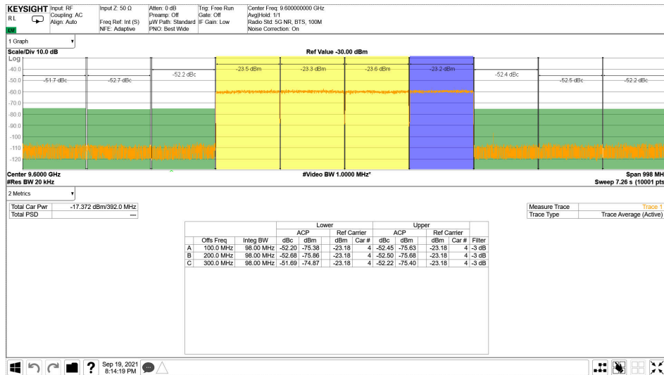
图 4-273. 9.61GHz 条件下 TX NR100MHz 输出频谱
