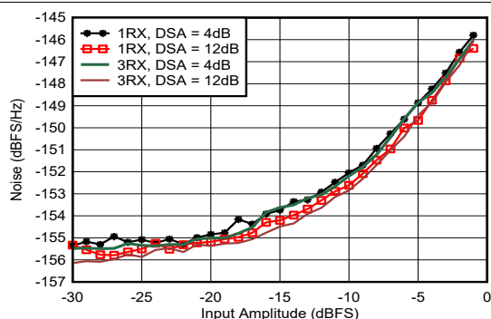
图 4-397. 4.9GHz 条件下 RX 噪声频谱密度与输入振幅和通道间的关系
