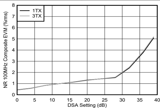
图 4-222. 8.11GHz 条件下 TX NR100MHz EVM 与 DSA 设置间的关系
