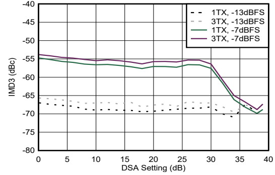
图 4-213. 8.11 GHz 条件下 TX IMD3 与 DSA 设置间的关系
