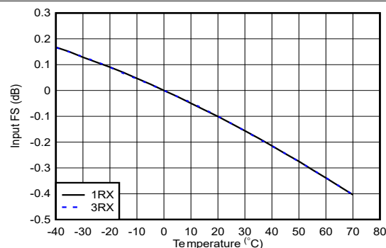
图 4-307. 1.75GHz 条件下 RX 输入满量程与温度和通道间的关系
