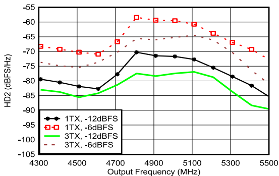
在 4.9GHz 条件下匹配, f_{\text{DAC}} = 11.79648\text{GSPS} , 交错模式, 标准化为谐波频率下的输出功率
