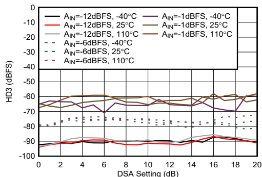
图 4-456. 9.6 GHz 条件下 RX HD3 与 DSA 设置间的关系
