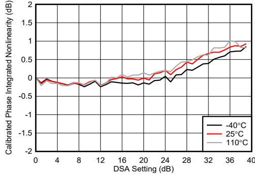
图 4-200. 8.1GHz 条件下 TX DSA 校准相位积分非线性
