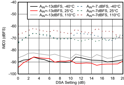
图 4-448. 9.6 GHz 条件下 RX IMD3 与 DSA 设置间的关系
