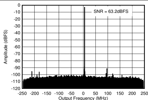
图 5-289. 0.8GHz 条件下的 RX 输出 FFT
