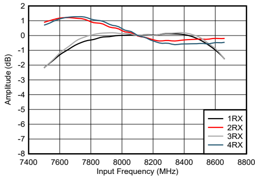
图 5-415. RX 振幅与频率和通道间的关系
