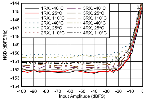
图 5-425. 8.1GHz 条件下 RX NSD 与数字振幅间的关系
