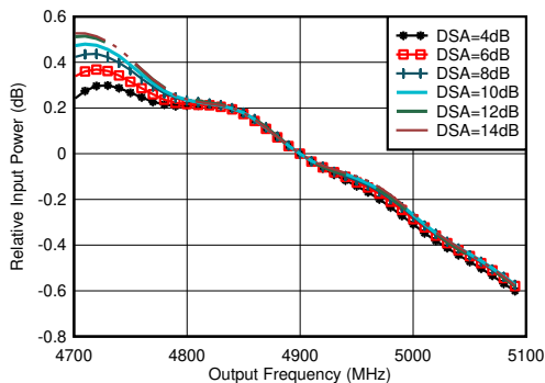
图 5-386. RX 带内增益平坦度， f_{\text{IN}} = 4900\text{MHz}
