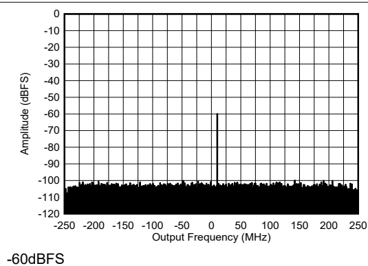
图 5-467. 9.61GHz 条件下 RX 单音输出 FFT
