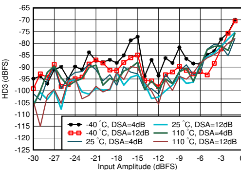
图 5-302. 0.8GHz 条件下 RX HD3 与 DSA 设置和温度间的关系
