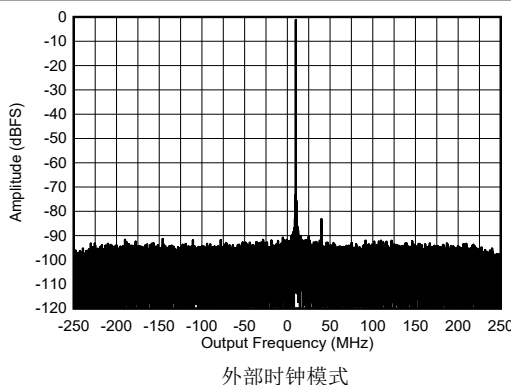
图 5-434. 8.1GHz 条件下 RX 单音输出 FFT，-1dBFS
