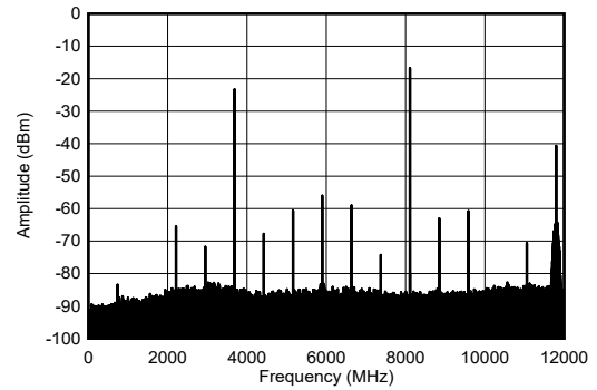
图 5-205. 8.1GHz 条件下 TX 单音输出频谱
