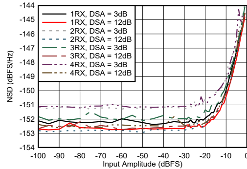
图 5-426. 8.1GHz 条件下 RX NSD 与数字振幅间的关系
