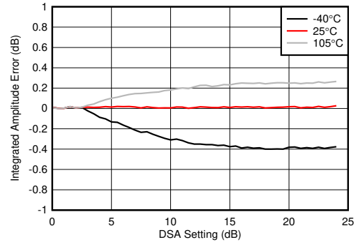
图 5-362. 3.6GHz 条件下 RX 校准差分振幅误差与 DSA 设置间的关系
