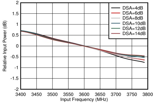
图 5-359. RX 带内增益平坦度， f_{\text{IN}} = 3600\text{MHz}
