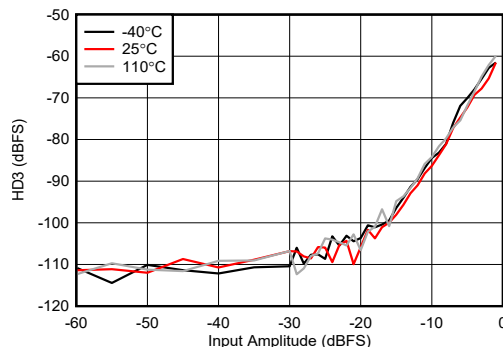
图 5-459. 9.6GHz 条件下 RX HD3 与数字电平间的关系
