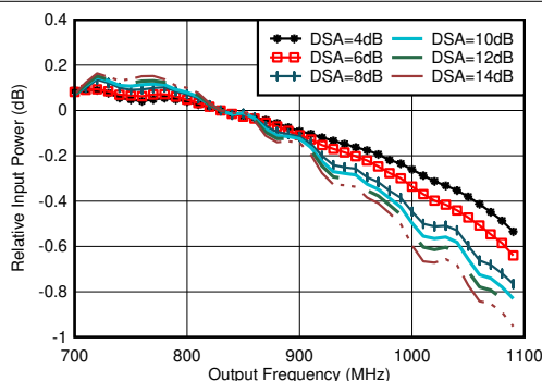
图 5-278. 通道 1RX 的 RX 带内增益平坦度， f_{\text{IN}} = 830\text{MHz}
