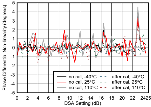
图 5-448. 9.6GHz 条件下 RX 相位微分非线性
