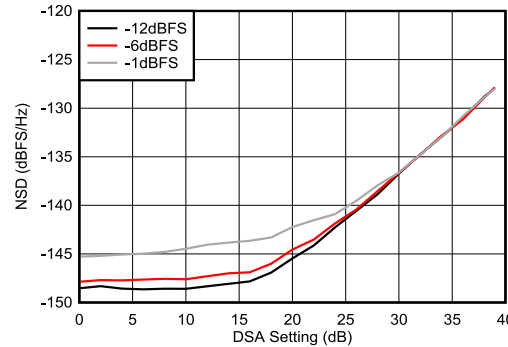
图 5-258. 9.61 GHz 条件下 TX NSD 与 DSA 设置间的关系
