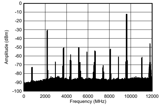
图 5-266. 9.61GHz 和 -12dBFS (宽带) 条件下 TX 单音频谱
