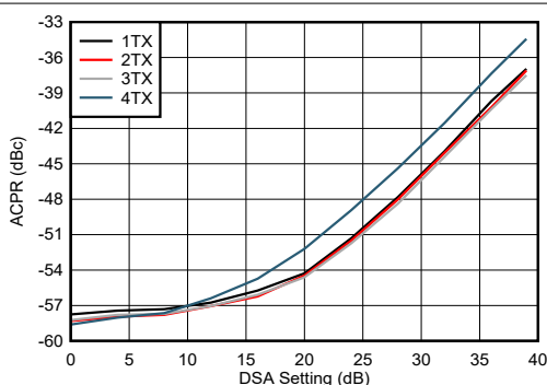
图 5-222. 8.11GHz 条件下 TX NR100MHz ACPR 与 DSA 设置间的关系
