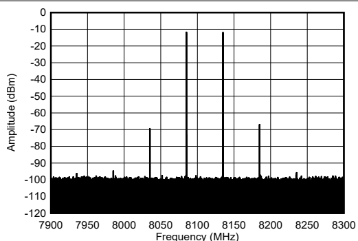
图 5-208. 8.11GHz 条件下 TX 单音输出频谱
