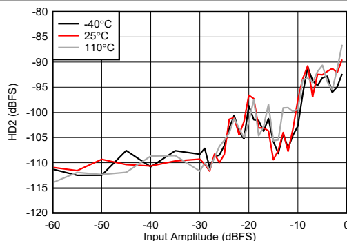
图 5-457. 9.6GHz 条件下 RX HD2 与数字电平间的关系
