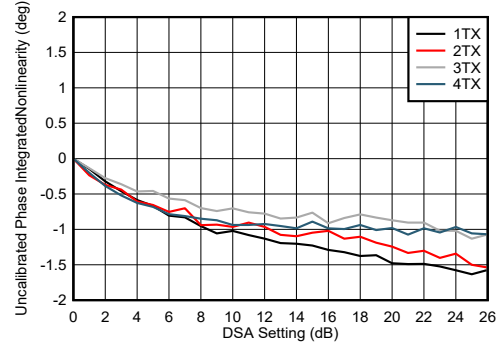
图 5-244. TX DSA 未校准相位积分非线性
