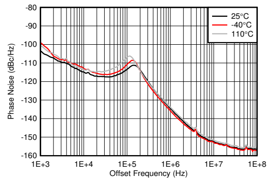
图 5-472. 12GHz 条件下 PLL 和外部时钟的相位噪声与偏移频率间的关系
