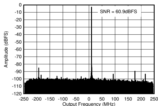
图 5-320. 1.75GHz 条件下的 RX 输出 FFT
