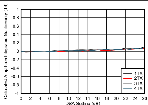
图 5-237. TX DSA 校准振幅积分非线性
