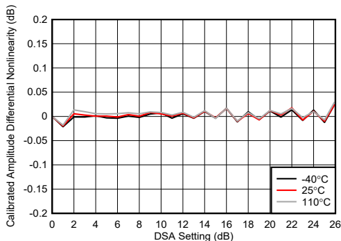
图 5-235. TX DSA 校准振幅微分非线性
