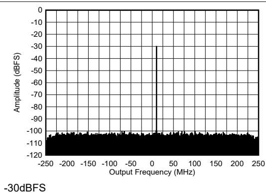
图 5-466. 9.61GHz 条件下 RX 单音输出 FFT
