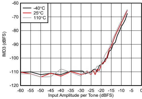
图 5-450. 9.6GHz 条件下 RX IMD3 与数字振幅间的关系
