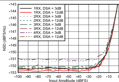
图 5-455. 9.6GHz 条件下 RX NSD 与数字振幅间的关系
