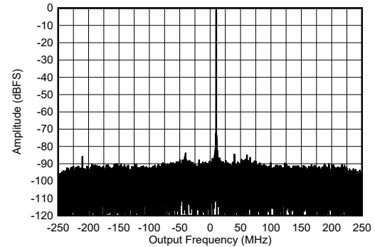
图 5-461. 9.61GHz 条件下 RX 单音输出 FFT
