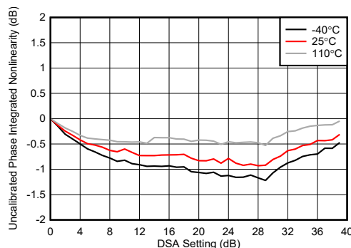
图 5-201. 8.11GHz 条件下 TX DSA 未校准相位积分非线性
