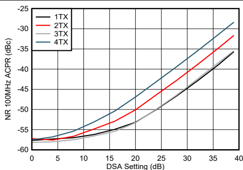
图 5-273. 9.61GHz 条件下 TX NR100MHz ACPR 与 DSA 设置间的关系
