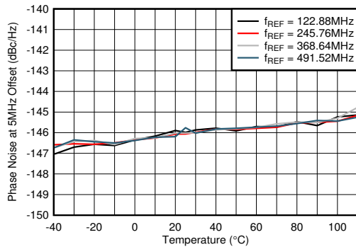
图 5-484. f_{OUT} = 2.6\text{GHz} 时 12GHz VCO 相位噪声 (5MHz 偏移条件下) 与温度和 f_{REF} 间的关系
