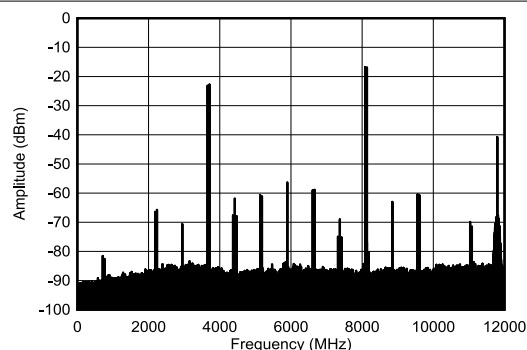
图 5-209. 8.11GHz 条件下 TX 双音输出频谱
