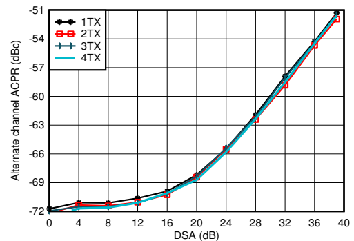
图 5-107. 2.6GHz 条件下 TX 20MHz LTE alt-ACPR 与 DSA 间的关系
