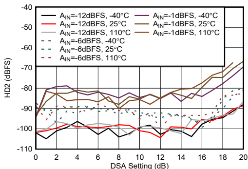
图 5-458. 9.6 GHz 条件下 RX HD2 与 DSA 设置间的关系
