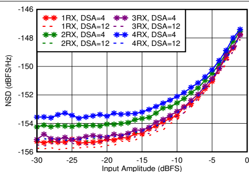
图 5-345. 2.6GHz 条件下 RX 噪声频谱密度与输入振幅和通道间的关系
