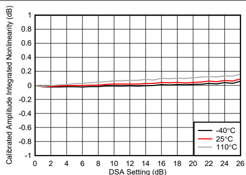
图 5-239. TX DSA 校准振幅积分非线性
