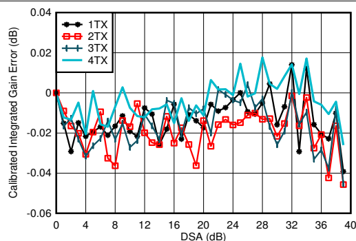
图 5-121. 3.5GHz 条件下 TX 校准差分增益误差与 DSA 设置和通道间的关系
