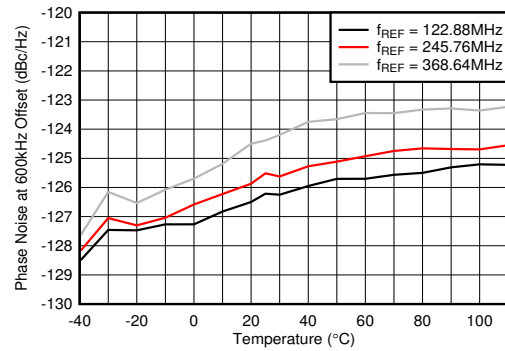
图 5-491. f_{OUT} = 2.6\text{GHz} 时 10GHz VCO 相位噪声 (600kHz 条件下) 与温度和 f_{REF} 间的关系
