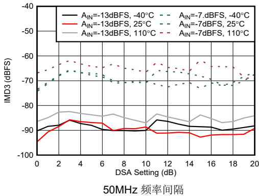
图 5-452. 9.6 GHz 条件下 RX IMD3 与 DSA 设置间的关系
