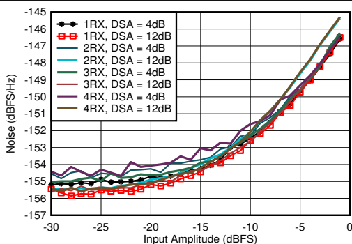
图 5-323. 1.75GHz 条件下 RX 噪声频谱密度与输入振幅和通道间的关系
