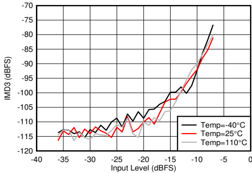
图 5-347. 2.6GHz 条件下 RX IMD3 与输入电平和温度间的关系
