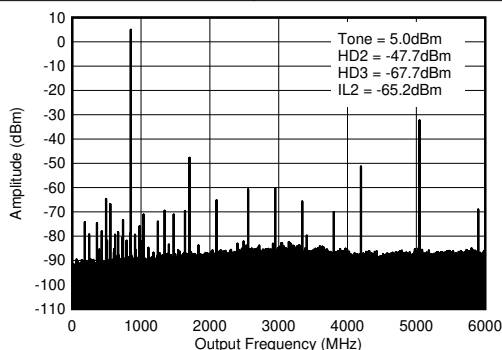
图 5-41. 0.85GHz ( 0-f_{\text{DAC}} ) 条件下的 TX 单频 (-12dBFS) 输出频谱
