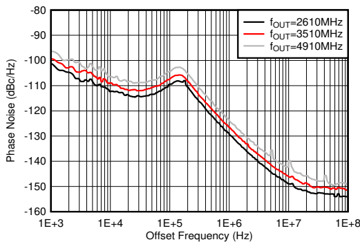
图 5-498. 25°C 条件下 9GHz VCO 相位噪声与偏移频率和 f_{OUT} 间的关系
