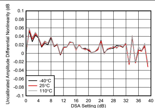
图 5-189. 8.11GHz 条件下 TX DSA 未校准振幅微分非线性
