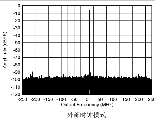
图 5-436. 8.1GHz 条件下 RX 单音输出 FFT，-6dBFS
