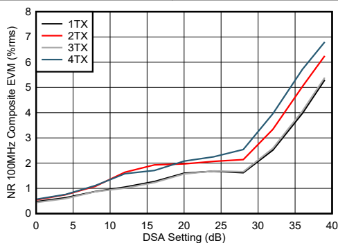
图 5-275. 9.61GHz 条件下 TX NR100MHz EVM 与 DSA 设置间的关系
