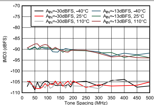
图 5-424. 8.1GHz 条件下 RX IMD3 与频率间隔间的关系
