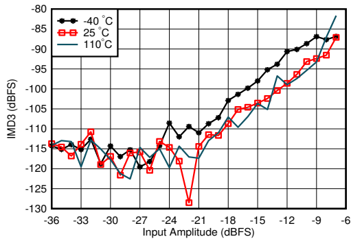
图 5-402. 4.9GHz 条件下 RX IMD3 与输入电平和温度间的关系
