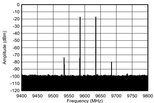
图 5-271. 9.61GHz 和 -12dBFS (400MHz 带宽) 条件下 TX 双音频谱
