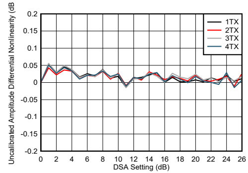
图 5-232. TX DSA 未校准振幅微分非线性
