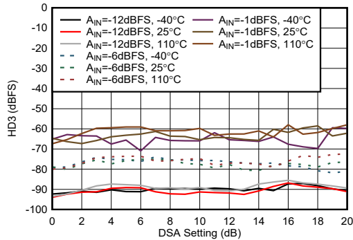
图 5-460. 9.6 GHz 条件下 RX HD3 与 DSA 设置间的关系
