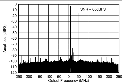
图 5-397. 4.9GHz 条件下的 RX 输出 FFT
