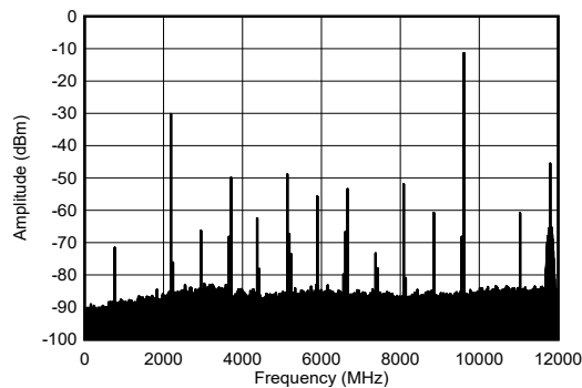
图 5-262. 9.61GHz 和 -1dBFS (宽带) 条件下 TX 单音频谱
