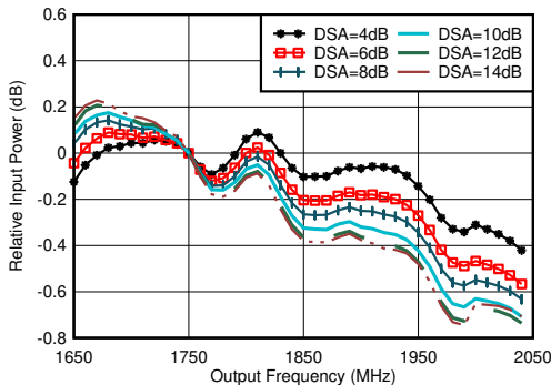
图 5-309. RX 带内增益平坦度， f_{\text{IN}} = 1750\text{MHz}
