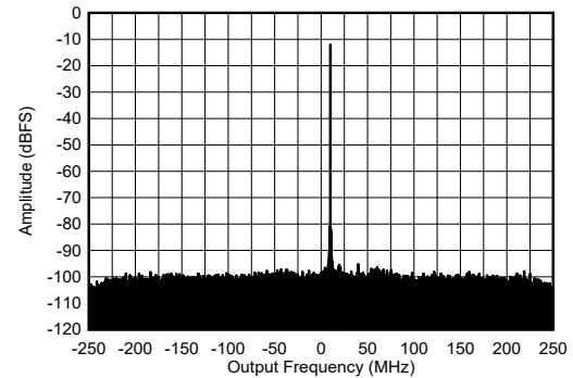
图 5-463. 9.61GHz 条件下 RX 单音输出 FFT
