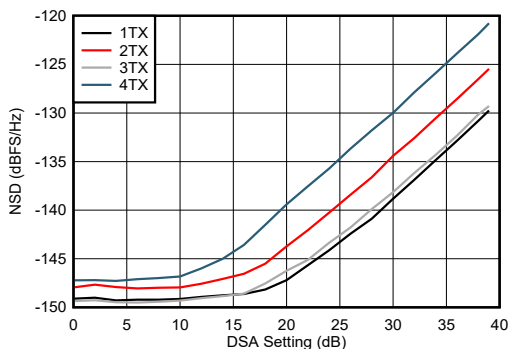
图 5-259. 9.61 GHz 条件下 TX NSD 与 DSA 设置间的关系
