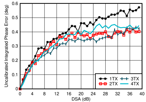
图 5-126. 3.5GHz 条件下 TX 未校准积分相位误差与 DSA 设置和通道间的关系
