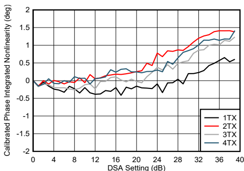
图 5-200. 8.11GHz 条件下 TX DSA 校准相位积分非线性
