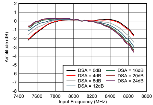
图 5-416. RX 振幅与频率和 DSA 设置间的关系
