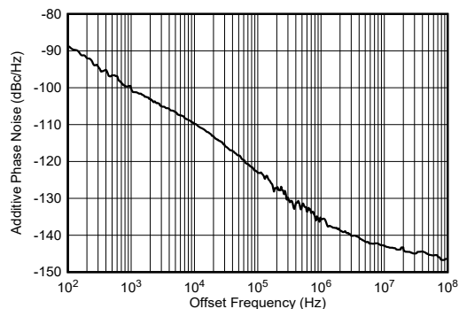
图 5-272. 9.61GHz 条件下 TX 附加相位噪声与偏移频率间的关系
