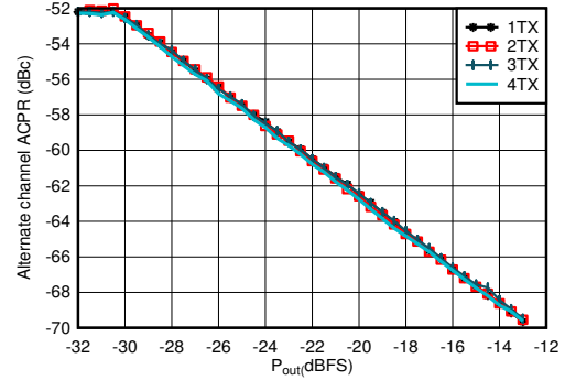
图 5-34. 0.85GHz 条件下 TX 20MHz LTE alt-ACPR 与数字电平间的关系
