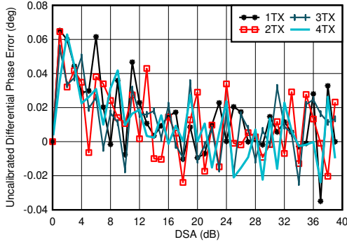
图 5-124. 3.5GHz 条件下 TX 未校准差分相位误差与 DSA 设置和通道间的关系
