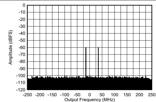
图 5-469. 9.61GHz 条件下 RX 双音输出 FFT
