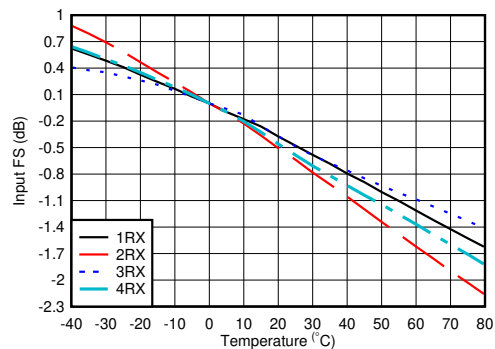
图 5-387. 4.9GHz 条件下 RX 输入满量程与温度和通道间的关系
