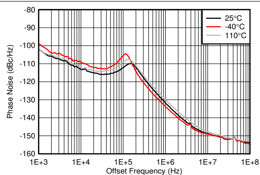
图 5-502. f_{OUT} = 1910\text{MHz} 时 8GHz VCO 相位噪声与偏移频率和温度间的关系
