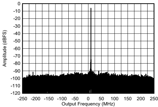
图 5-462. 9.61GHz 条件下 RX 单音输出 FFT
