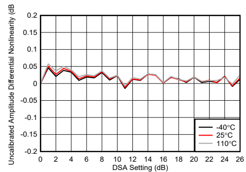
图 5-234. TX DSA 未校准振幅微分非线性
