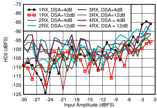
图 5-327. 1.9GHz 条件下 RX HD2 与 DSA 设置和通道间的关系
