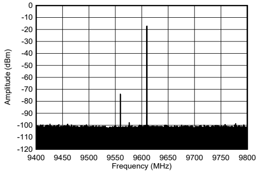
图 5-265. 9.61GHz 和 -6dBFS (400MHz 带宽) 条件下 TX 单音频谱
