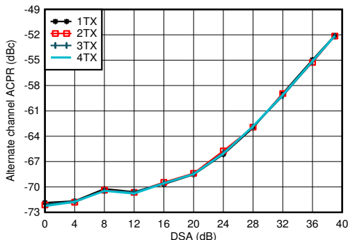
图 5-70. 1.8425GHz 条件下 TX 20MHz LTE alt-ACPR 与数字电平间的关系
