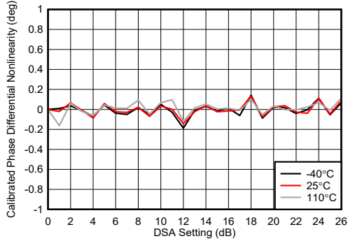
图 5-243. TX DSA 校准相位微分非线性
