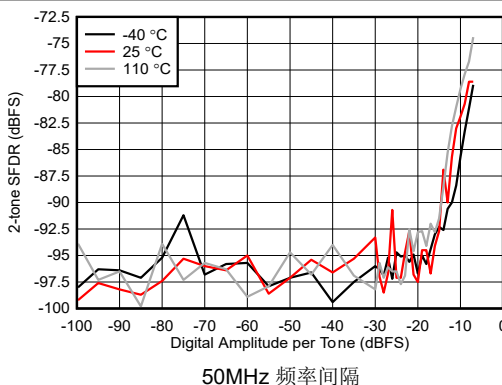
图 5-433. 8.1GHz 条件下 RX 双音 SFDR 与数字振幅间的关系
