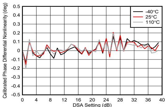
图 5-198. 8.11GHz 条件下 TX DSA 校准相位微分非线性
