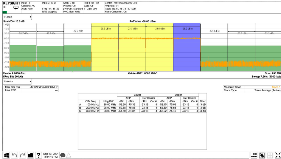
图 5-276. 9.61GHz 条件下 TX NR100MHz 输出频谱
