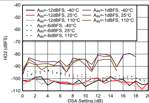
图 5-430. 8.1GHz 条件下 RX HD2 与 DSA 设置间的关系
