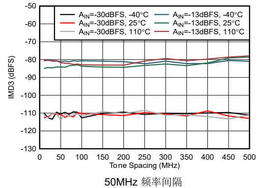
图 5-453. 9.6 GHz 条件下 RX IMD3 与频率间隔间的关系
