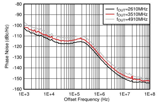
图 5-487. 25°C 条件下 10GHz VCO 相位噪声与偏移频率和 f_{OUT} 间的关系
