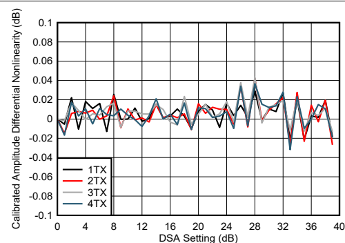
图 5-188. 8.11GHz 条件下 TX DSA 校准振幅微分非线性
