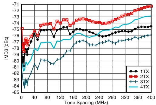
图 5-22. 0.85GHz 条件下 TX IMD3 与频率间隔和通道间的关系
