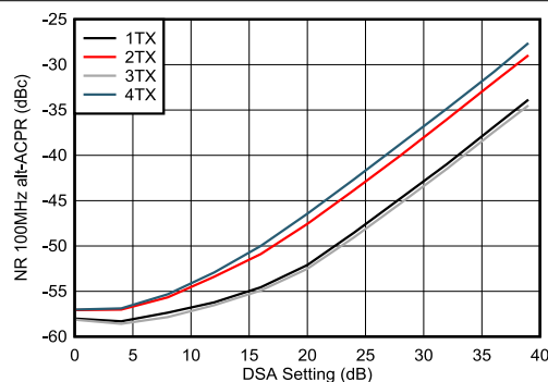
图 5-274. 9.61GHz 条件下 TX NR100MHz alt-ACPR 与 DSA 设置间的关系
