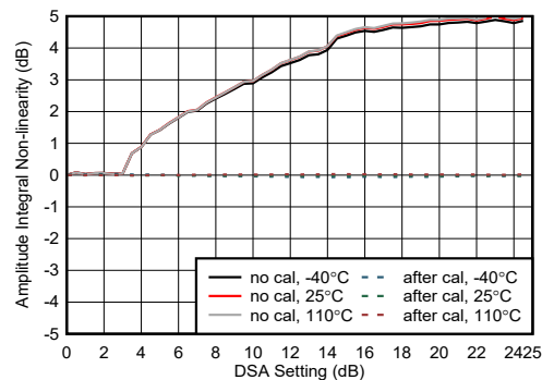
图 5-447. 9.6GHz 条件下 RX 振幅积分非线性
