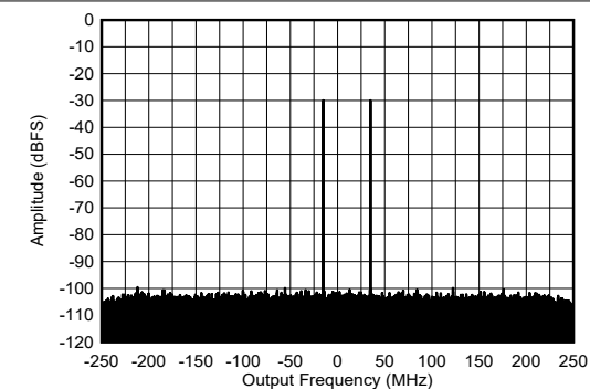
图 5-468. 9.61GHz 条件下 RX 双音输出 FFT
