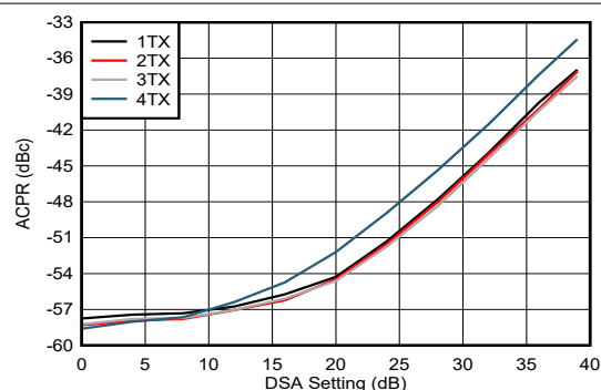
图 5-223. 8.11GHz 条件下 TX NR100MHz alt-ACPR 与 DSA 设置间的关系
