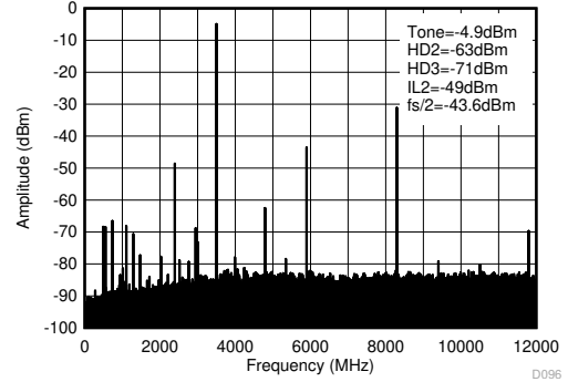
图 5-147. 3.5GHz (0 - f_{\text{DAC}} ) 条件下的 TX 单频 (-6dBFS) 输出频谱
