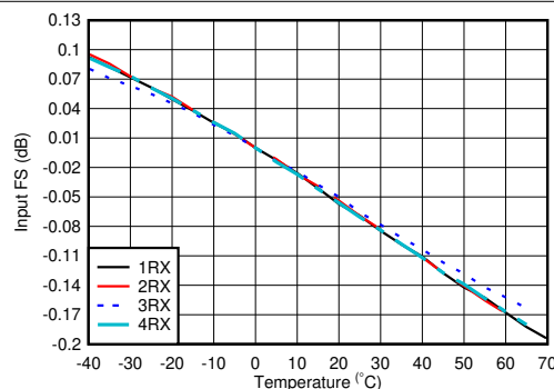
图 5-279. 800MHz 条件下 RX 输入满量程与温度和通道间的关系
