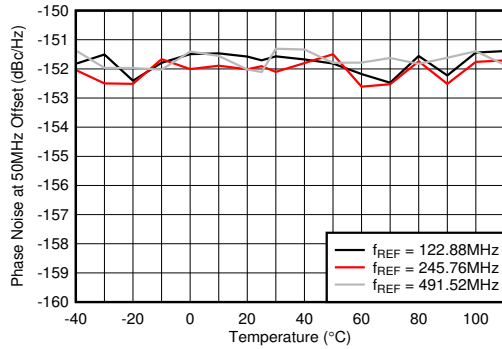
图 5-496. f_{OUT} = 2.6\text{GHz} 时 10GHz VCO 相位噪声 (50MHz 条件下) 与温度和 f_{REF} 间的关系
