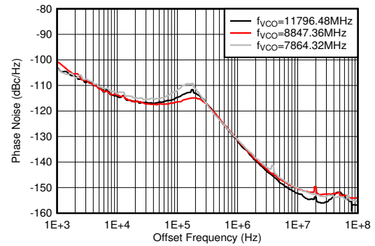
图 5-473. f_{\text{OUT}} = 2610\text{MHz} 时相位噪声与偏移频率和 f_{\text{VCO}} 间的关系
