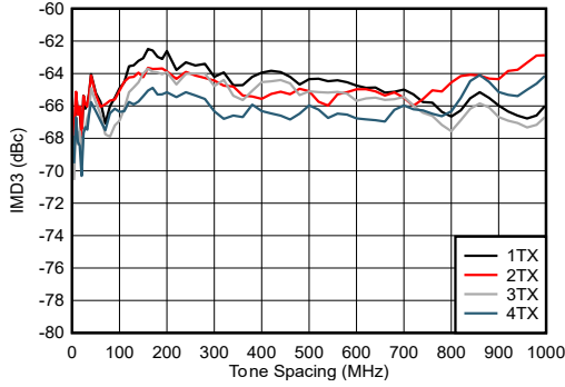
图 5-253. 9.61GHz 条件下 TX IMD3 与频率间隔间的关系
