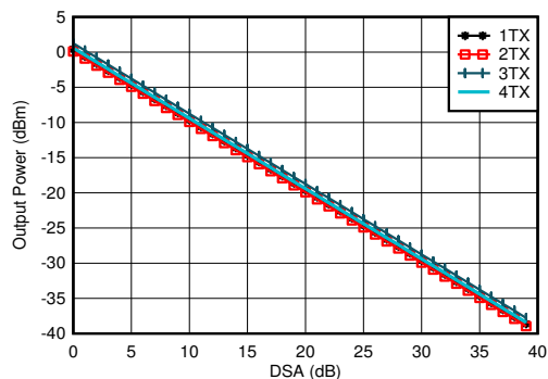
图 5-119. 3.5GHz 条件下 TX 输出功率与 DSA 设置间的关系
