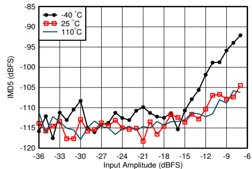
图 5-297. 0.8GHz 条件下 Rx IMD5 与输入电平和温度间的关系
