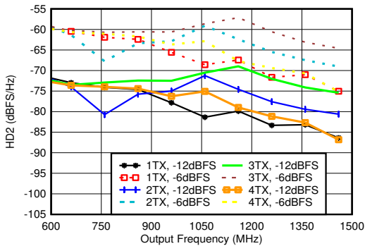
图 5-37. 0.85GHz 条件下 TX HD2 与数字振幅和输出频率间的关系
