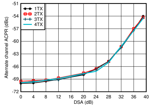
图 5-34. 0.85GHz 条件下 TX 20MHz LTE alt-ACPR 与数字电平间的关系
