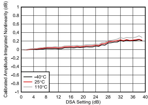
图 5-194. 8.1GHz 条件下 TX DSA 校准振幅积分非线性
