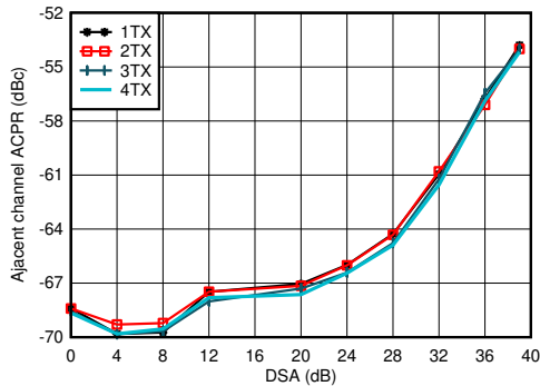
图 5-33. 0.85GHz 条件下 TX 20MHz LTE ACPR 与数字电平间的关系
