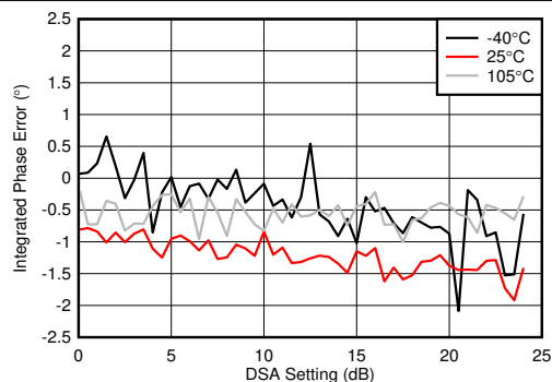
图 5-366. 3.6GHz 条件下 RX 校准差分相位误差与 DSA 设置间的关系
