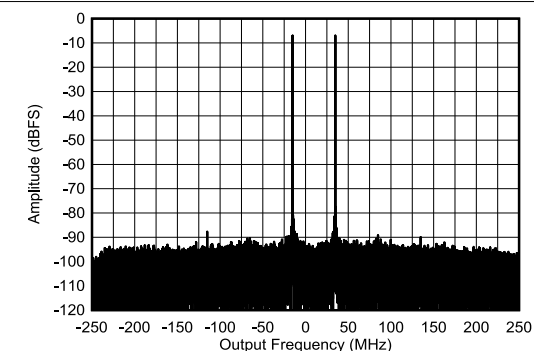
图 5-466. 9.61GHz 条件下 RX 单音输出 FFT
