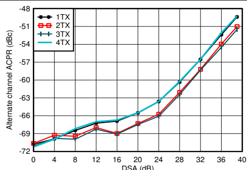
图 5-176. 4.9GHz 条件下 TX 20MHz LTE alt-ACPR 与数字电平间的关系
