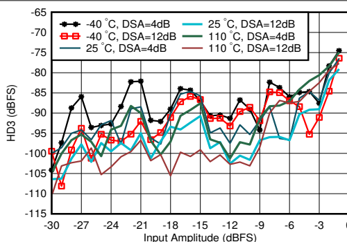
图 5-332. 1.9GHz 条件下 RX HD3 与 DSA 设置和温度间的关系
