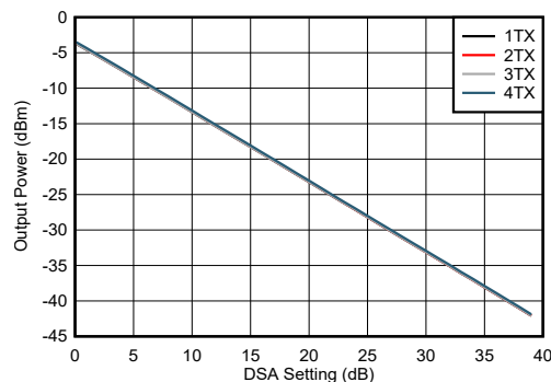
图 5-185. 8.11 GHz 条件下 TX 输出功率与 DSA 设置间的关系
