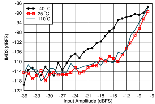
图 5-295. 0.8GHz 条件下 RX IMD3 与输入电平和温度间的关系
