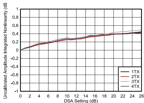
图 5-236. TX DSA 未校准振幅积分非线性
