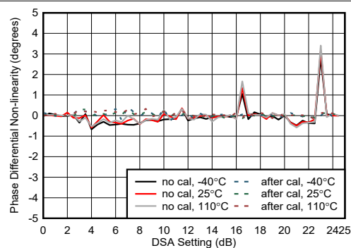
图 5-420. 8.1GHz 条件下 RX 相位微分非线性
