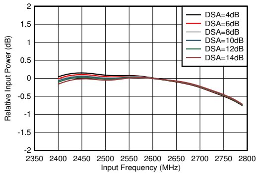
图 5-339. RX 带内增益平坦度， f_{\text{IN}} = 2600\text{MHz}
