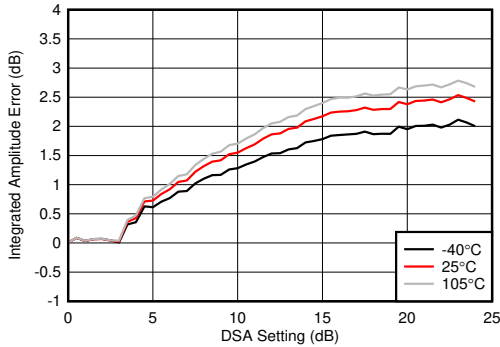
图 5-361. 3.6GHz 条件下 RX 未校准差分振幅误差与 DSA 设置间的关系
