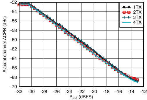
图 5-33. 0.85GHz 条件下 TX 20MHz LTE ACPR 与数字电平间的关系
