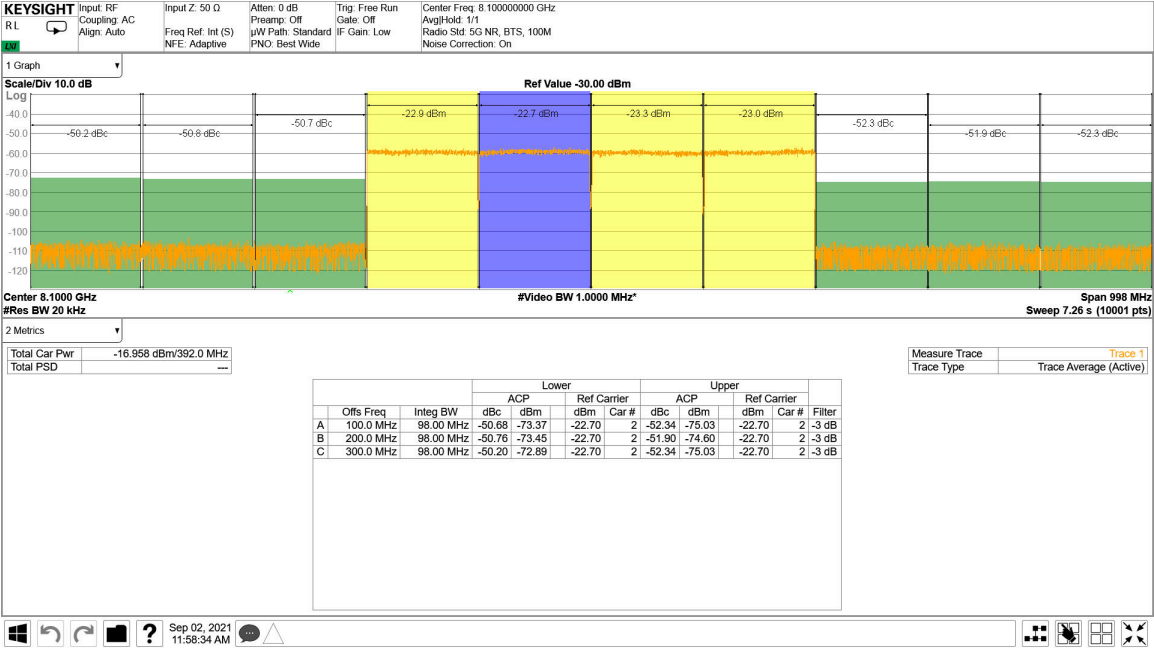
图 5-227. 8.11GHz 条件下 TX 4x100MHz NR 输出频谱
