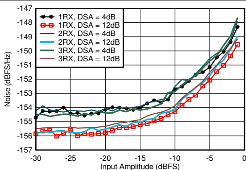
图 5-292. 0.8GHz 条件下 RX 噪声频谱密度与输入振幅和通道间的关系
