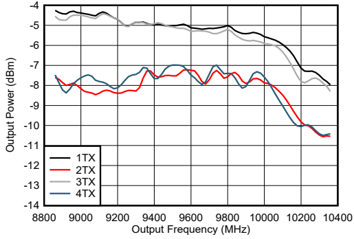
图 5-229. 9.61GHz 条件下 TX 输出功率与频率间的关系
