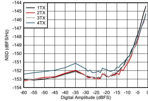
图 5-256. 9.61GHz 条件下 TX NSD 与数字振幅间的关系
