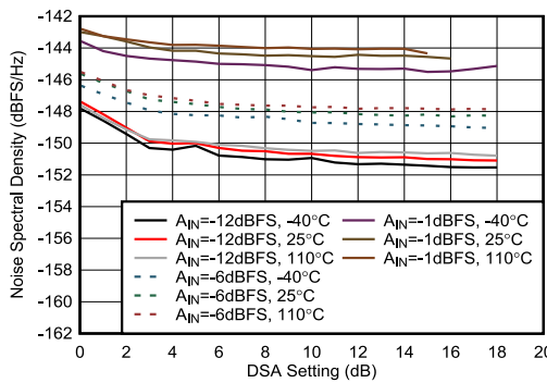
图 5-427. 8.1GHz 条件下 RX NSD 与 DSA 设置间的关系
