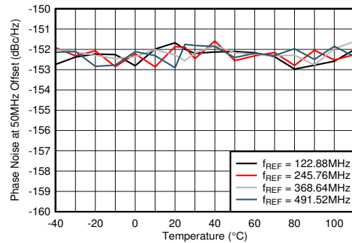
图 5-485. f_{OUT} = 2.6\text{GHz} 时 12GHz VCO 相位噪声 (50MHz 偏移条件下) 与温度和 f_{REF} 间的关系
