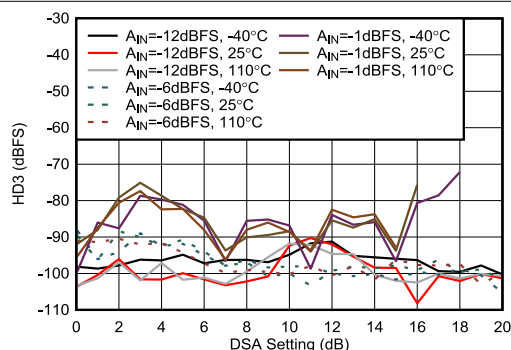
图 5-432. 8.1 GHz 条件下 RX HD3 与 DSA 设置间的关系
