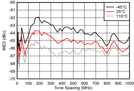
图 5-255. 9.61GHz 条件下 TX IMD3 与频率间隔间的关系
