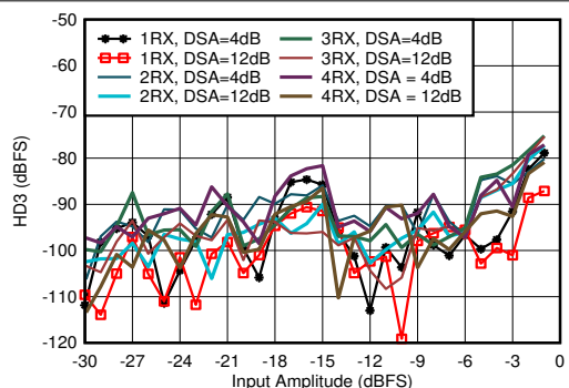
图 5-331. 1.9GHz 条件下 RX HD3 与 DSA 设置和通道间的关系
