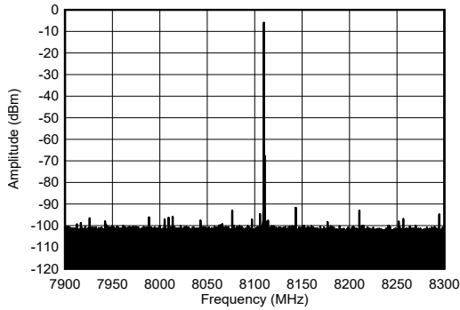
图 5-204. 8.1GHz 条件下 TX 单音输出频谱
