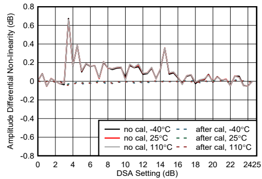
图 5-418. 8.11GHz 条件下 RX 振幅微分非线性
