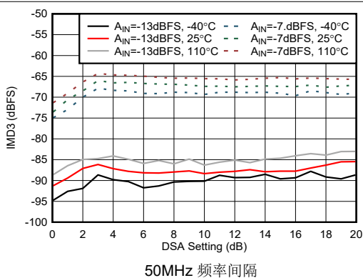
图 5-423. 8.1GHz 条件下 RX IMD3 与 DSA 设置间的关系
