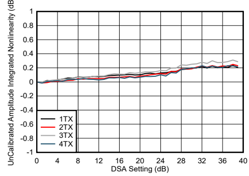
图 5-191. 8.1GHz 条件下 TX DSA 未校准振幅积分非线性
