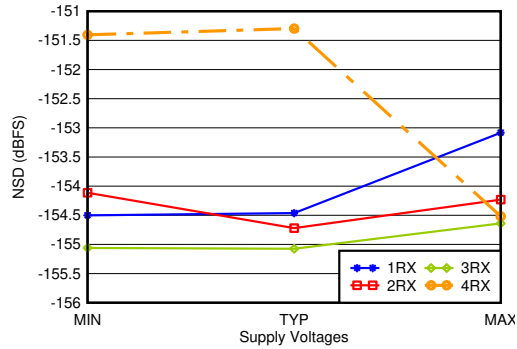
图 5-414. 4.9GHz 条件下 RX 噪声频谱密度与电源和通道间的关系
