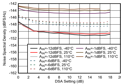
图 5-426. 8.1GHz 条件下 RX NSD 与数字振幅间的关系
