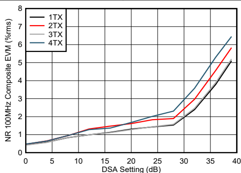
图 5-224. 8.11GHz 条件下 TX NR100MHz EVM 与 DSA 设置间的关系
