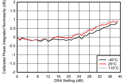
图 5-202. 8.1GHz 条件下 TX DSA 校准相位积分非线性
