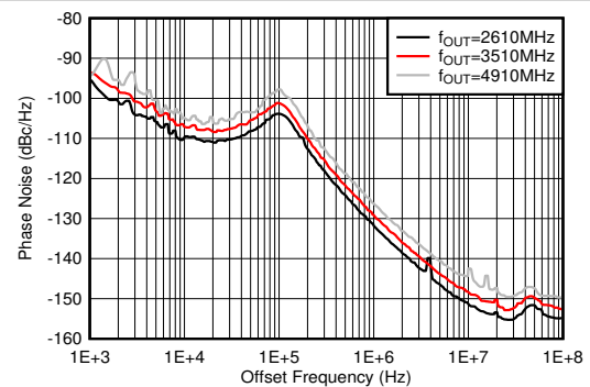
图 5-475. 25°C 条件下 12GHz VCO 相位噪声与偏移频率和 f_{\text{OUT}} 间的关系
