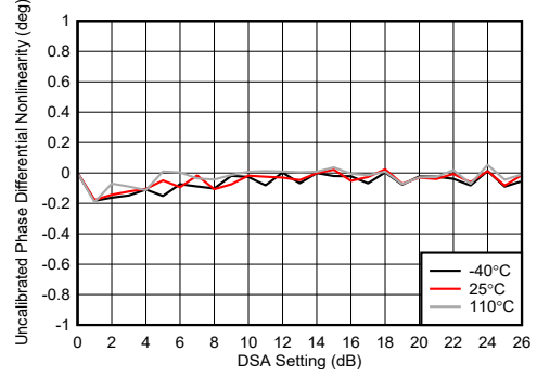
图 5-242. TX DSA 未校准相位微分非线性
