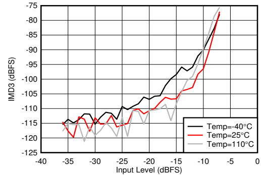
图 5-348. 2.6GHz 条件下 RX IMD3 与输入电平和温度间的关系
