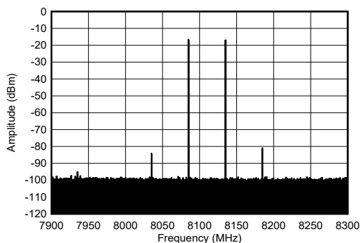
图 5-210. 8.11GHz 条件下 TX 双音输出频谱
