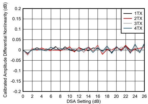
图 5-233. TX DSA 校准振幅微分非线性
