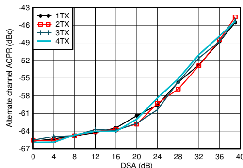
图 5-111. 2.6GHz 条件下 TX 100MHz NR alt-ACPR 与 DSA 间的关系
