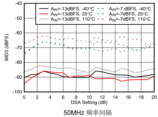
图 5-451. 9.6 GHz 条件下 RX IMD3 与 DSA 设置间的关系
