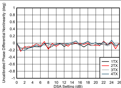
图 5-240. TX DSA 未校准相位微分非线性
