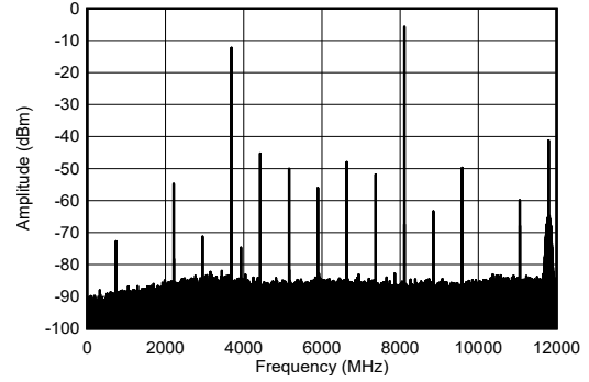
图 5-203. 8.1GHz 条件下 TX 单音输出频谱
