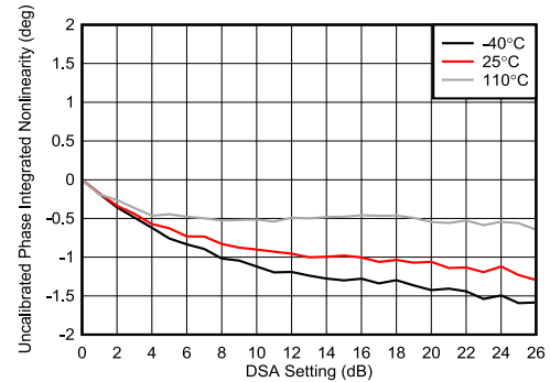
图 5-246. TX DSA 未校准相位积分非线性
