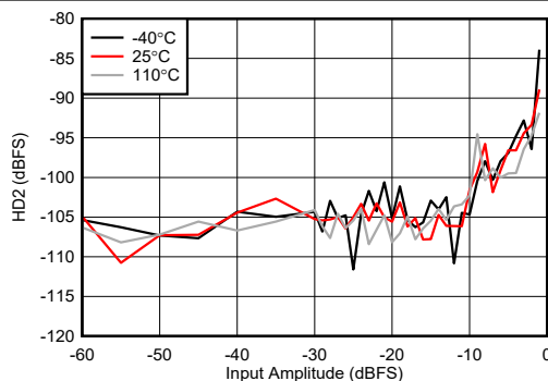
图 5-429. 8.1GHz 条件下 RX HD2 与数字振幅间的关系
