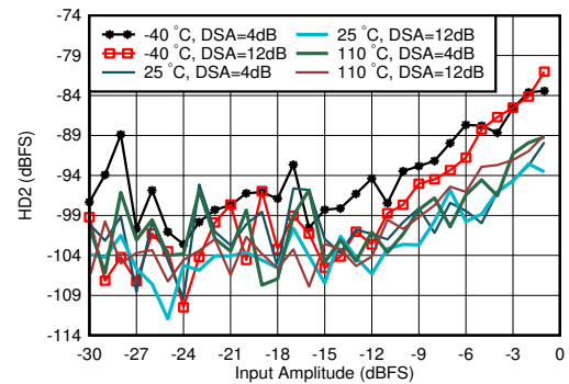
图 5-328. 1.9GHz 条件下 RX HD2 与 DSA 设置和温度间的关系
