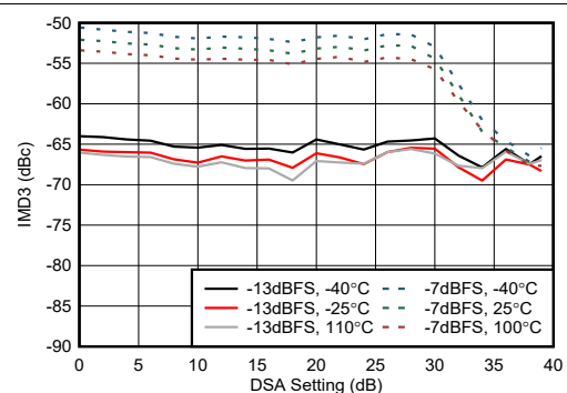
图 5-250. 9.61 GHz 条件下 TX IMD3 与 DSA 设置间的关系
