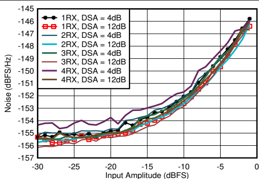
图 5-400. 4.9GHz 条件下 RX 噪声频谱密度与输入振幅和通道间的关系
