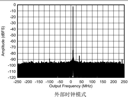
图 5-435. 8.1GHz 条件下 RX 单音输出 FFT，-3dBFS
