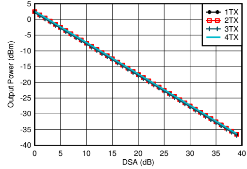
图 5-79. 2.6GHz 条件下 TX 输出功率与 DSA 设置和通道间的关系
