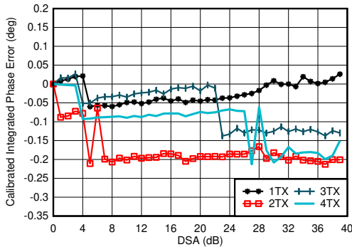
图 5-13. 0.85GHz 条件下 TX 校准差分相位误差与 DSA 设置和通道间的关系
