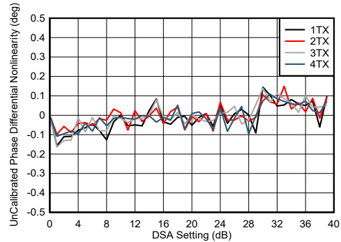
图 5-195. 8.1GHz 条件下 TX DSA 未校准相位微分非线性
