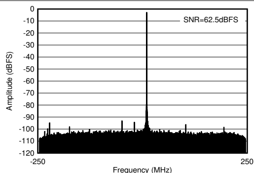
图 5-342. 2.6GHz 条件下的 RX 输出 FFT
