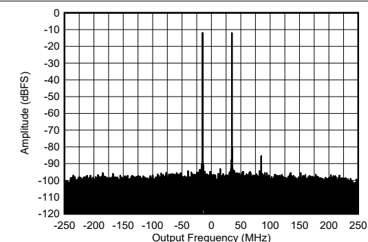
图 5-467. 9.61GHz 条件下 RX 单音输出 FFT
