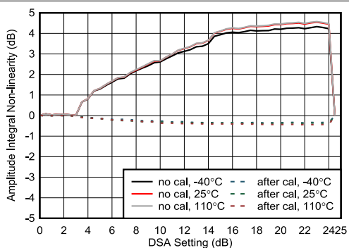
图 5-419. 8.1GHz 条件下 RX 振幅积分非线性
