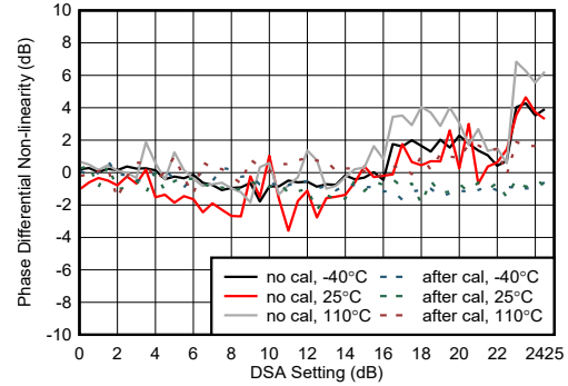
图 5-449. 9.6GHz 条件下 RX 相位微分非线性
