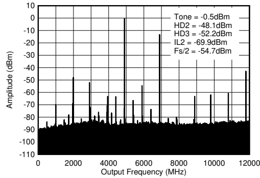
图 5-181. 4.9GHz (0 - f_{\text{DAC}} ) 条件下的 TX 单频 (-12dBFS) 输出频谱
