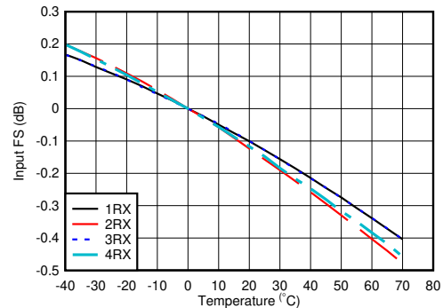
图 5-310. 1.75GHz 条件下 RX 输入满量程与温度和通道间的关系
