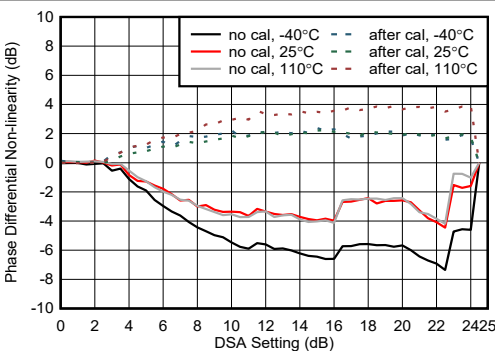
图 5-421. 8.1GHz 条件下 RX 相位微分非线性
