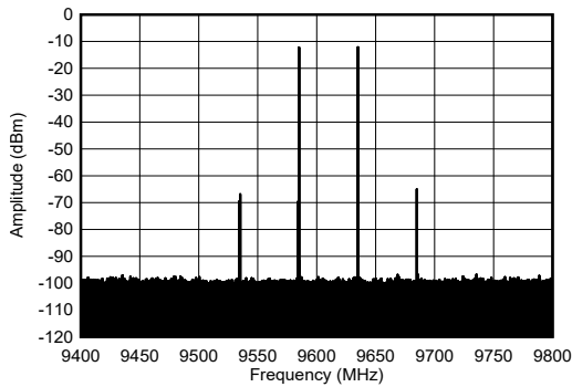
图 5-267. 9.61GHz 和 -12dBFS (400MHz 带宽) 条件下 TX 单音频谱
