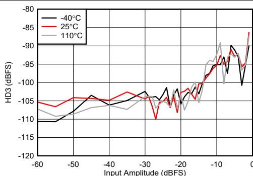
图 5-431. 8.1GHz 条件下 RX HD3 与数字振幅间的关系
