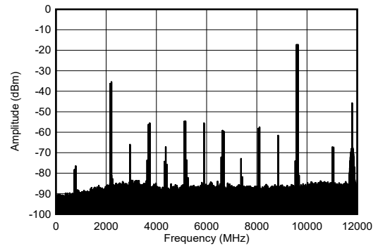
图 5-270. 9.61GHz 和 -12dBFS (宽带) 条件下 TX 双音频谱
