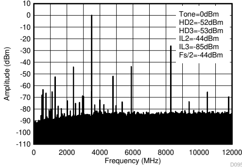
图 5-146. 3.5GHz (0 - f_{\text{DAC}} ) 条件下的 TX 单频 (-1dBFS) 输出频谱
