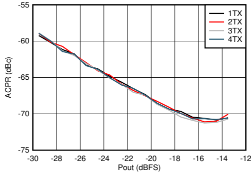
图 5-104. 2.6GHz 条件下 TX 20MHz LTE ACPR 与数字电平间的关系
