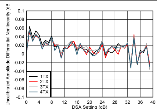
图 5-187. 8.11GHz 条件下 TX DSA 未校准振幅微分非线性
