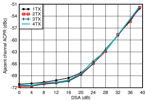
图 5-106. 2.6GHz 条件下 TX 20MHz LTE ACPR 与 DSA 间的关系
