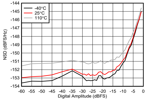
图 5-257. 9.61GHz 条件下 TX NSD 与数字振幅间的关系
