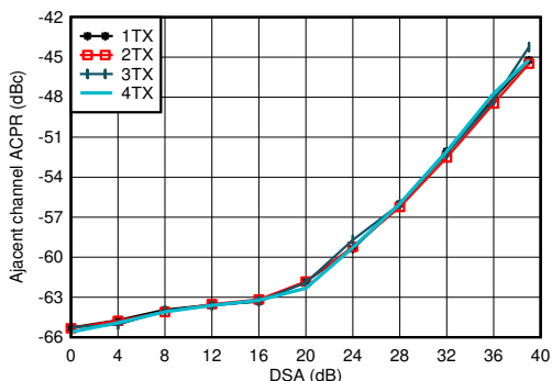
图 5-110. 2.6GHz 条件下 TX 100MHz NR ACPR 与 DSA 间的关系
