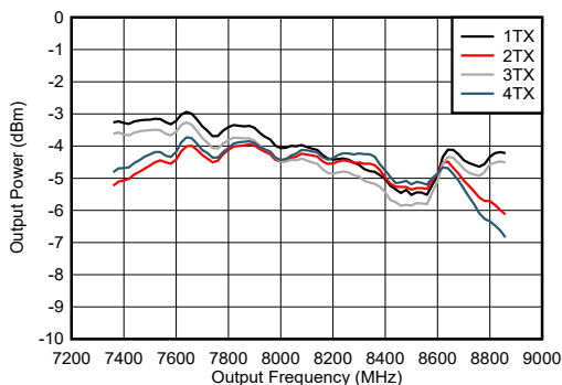
图 5-184. 8.11GHz 条件下 TX 输出功率与频率间的关系
