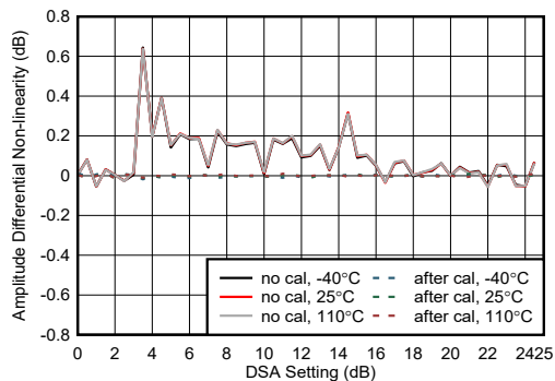
图 5-446. 9.6GHz 条件下 RX 振幅微分非线性
