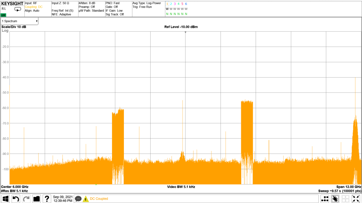
图 5-228. 8.11GHz 条件下 TX 4x100MHz NR 输出频谱
