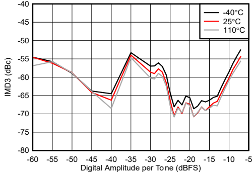
图 5-214. 8.11GHz 条件下 TX IMD3 与数字振幅间的关系
