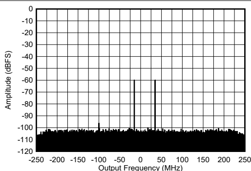
图 5-443. 8.1GHz 条件下 RX 双音输出 FFT
