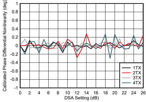
图 5-241. TX DSA 校准相位微分非线性
