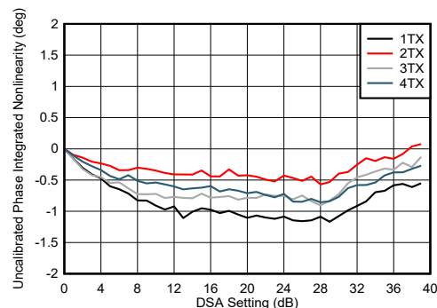
图 5-199. 8.11GHz 条件下 TX DSA 未校准相位积分非线性
