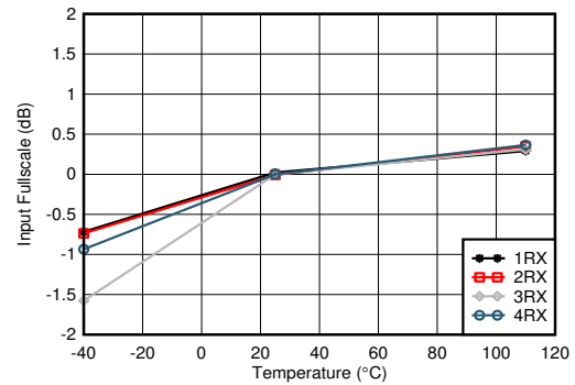
图 5-340. 2.6GHz 条件下 RX 输入满量程与温度和通道间的关系
