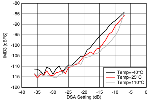
图 5-371. 3.6GHz 条件下 RX IMD3 与输入电平和温度间的关系
