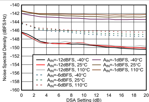
图 5-456. 9.6 GHz 条件下 RX NSD 与 DSA 设置间的关系
