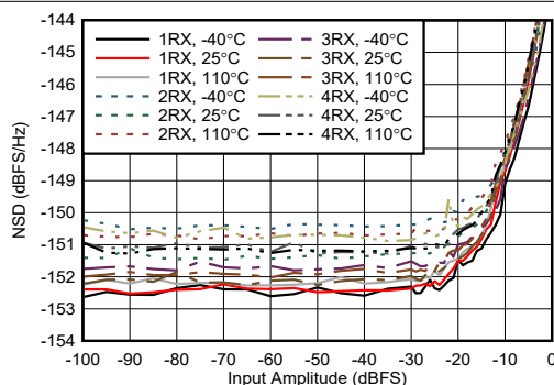
图 5-454. 9.6GHz 条件下 RX NSD 与数字振幅间的关系
