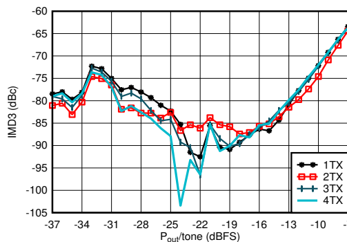
图 5-28. 0.85GHz 条件下 TX IMD3 与数字电平间的关系
