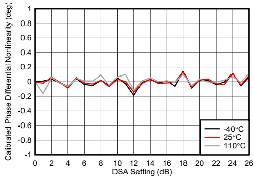
图 5-245. TX DSA 校准相位积分非线性
