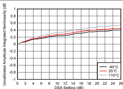
图 5-238. TX DSA 未校准振幅积分非线性
