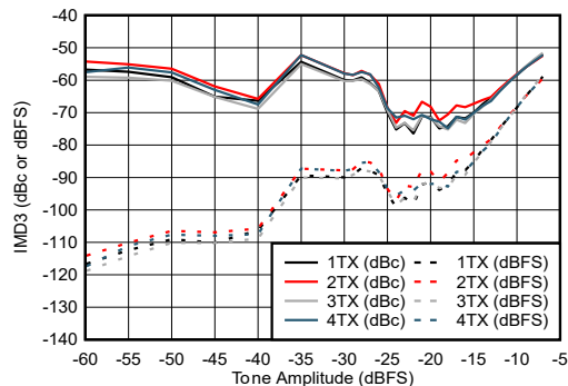
图 5-248. 9.61GHz 条件下 TX IMD3 与数字振幅间的关系
