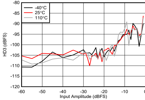
图 4-438. 8.1GHz 条件下 RX HD3 与数字振幅间的关系
