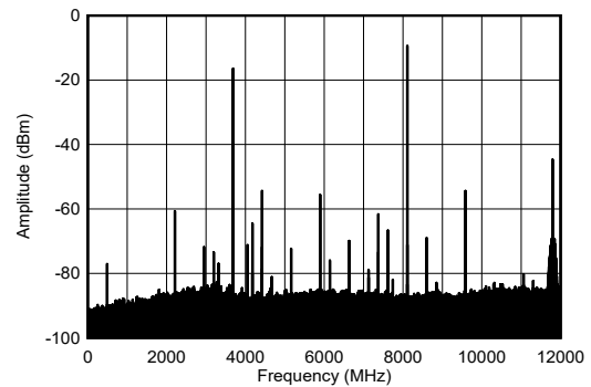
图 4-203. 8.1GHz 条件下 TX 单音输出频谱
