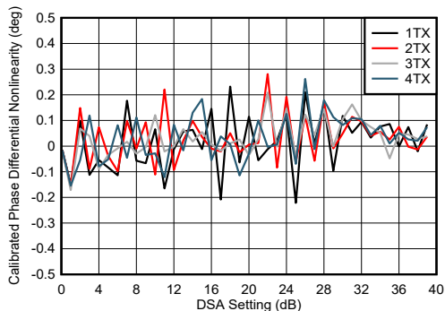
图 4-196. 8.11GHz 条件下 TX DSA 已校准相位微分非线性
