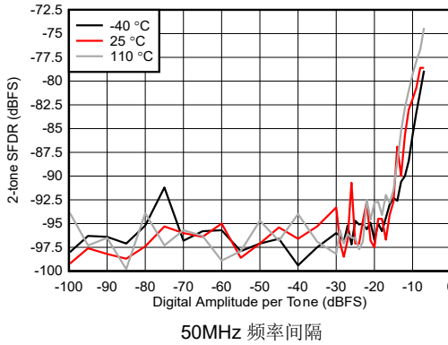
图 4-440. 8.1GHz 条件下 RX 双音 SFDR 与数字振幅间的关系
