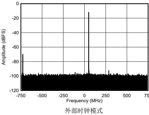
图 4-442. 8.1GHz 条件下 RX 单频输出 FFT, -12dBFS
