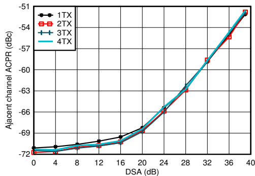
图 4-108. 2.6GHz 条件下 TX 20MHz LTE ACPR 与 DSA 间的关系
