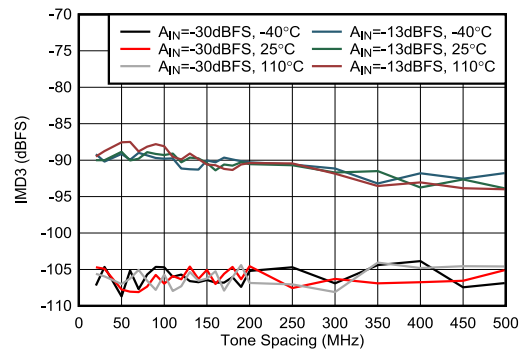
图 4-431. 8.1GHz 条件下 RX IMD3 与频率间隔间的关系
