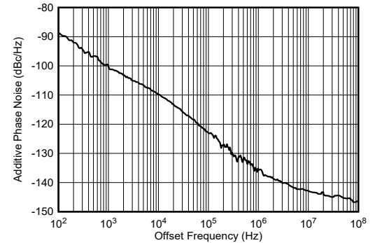
图 4-280. 9.61GHz 条件下 TX 附加相位噪声与偏移频率间的关系
