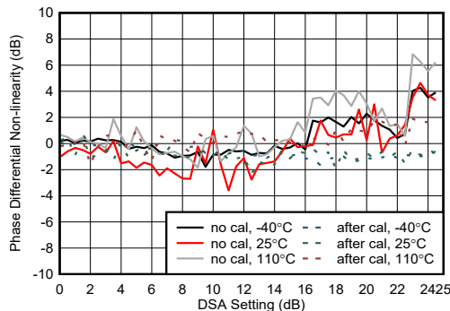
图 4-454. 9.6GHz 条件下 RX 相位积分非线性
