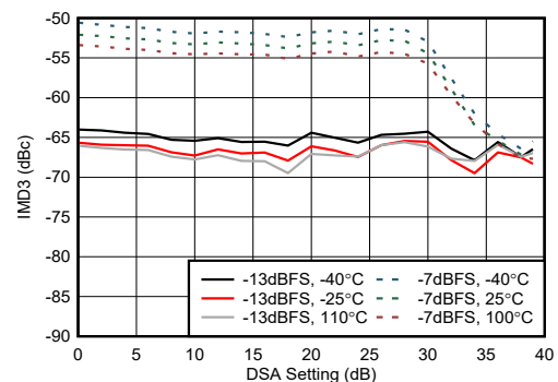
图 4-254. 9.6GHz 条件下 TX IMD3 与 DSA 设置间的关系
