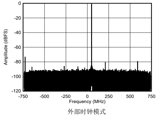
图 4-441. 8.1GHz 条件下 RX 单频输出 FFT, -1dBFS
