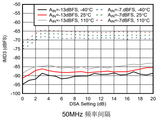
图 4-430. 8.1GHz 条件下 RX IMD3 与 DSA 设置间的关系
