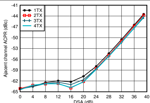
图 4-175. 4.9GHz 条件下 TX 20MHz LTE ACPR 与数字电平间的关系
