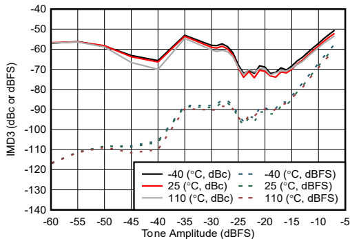
图 4-253. 9.6GHz 条件下 TX IMD3 与数字振幅间的关系
