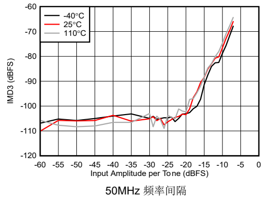
图 4-429. 8.1GHz 条件下 RX IMD3 与输入振幅间的关系
