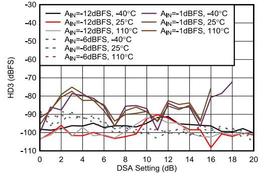
图 4-439. 8.1GHz 条件下 RX HD3 与 DSA 设置间的关系
