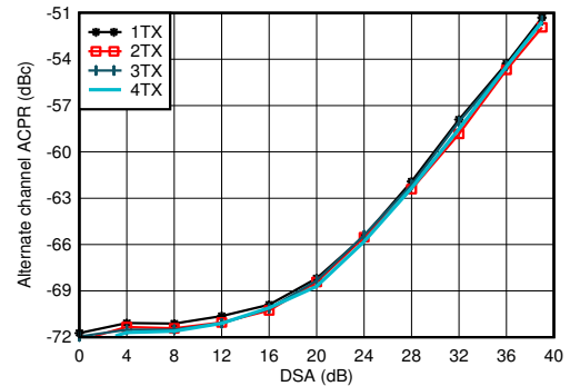
图 4-105. 2.6GHz 条件下 TX 20MHz LTE alt-ACPR 与数字电平间的关系
