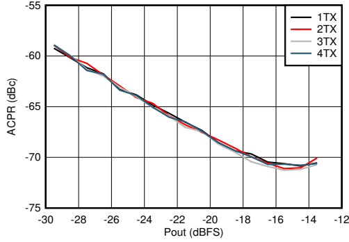
图 4-104. 2.6GHz 条件下 TX 20MHz LTE ACPR 与数字电平间的关系
