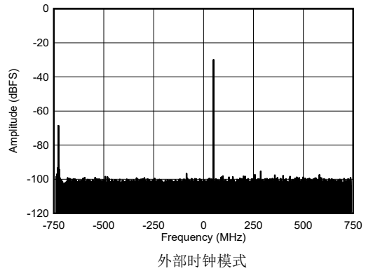
图 4-443. 8.1GHz 条件下 RX 单频输出 FFT, -30dBFS
