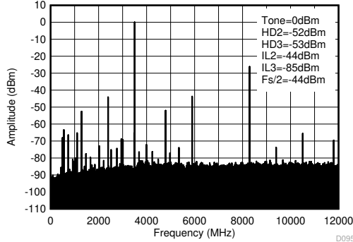
图 4-146. 3.5GHz (0 - f_{\text{DAC}} ) 条件下的 TX 单音 (-1dBFS) 输出频谱
