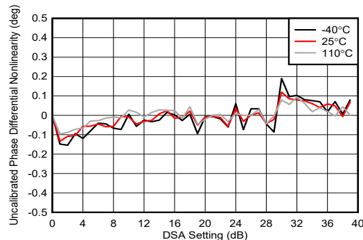
图 4-197. 8.11GHz 条件下 TX DSA 未校准相位微分非线性
