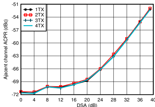
图 4-71. 1.8GHz 条件下 TX 20MHz LTE ACPR 与 DSA 间的关系
