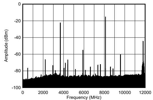
图 4-205. 8.1GHz 条件下 TX 单音输出频谱
