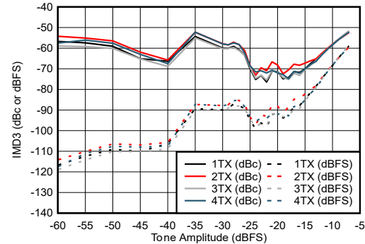
图 4-252. 9.6GHz 条件下 TX IMD3 与数字振幅间的关系
