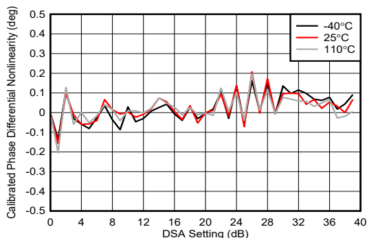
图 4-198. 8.11GHz 条件下 TX DSA 已校准相位微分非线性
