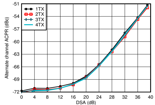
图 4-107. 2.6GHz 条件下 TX 20MHz LTE alt-ACPR 与 DSA 间的关系
