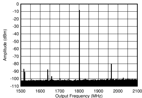
图 4-367. 1.8GHz ( \pm 300\text{MHz} ) 条件下的 TX 单音 (-1dBFS) 输出频谱
