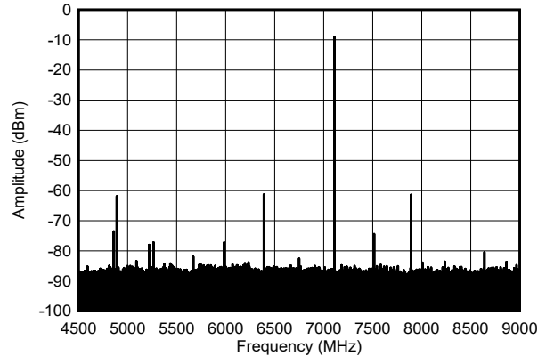
图 4-577. 7.1GHz、-1dBFS (奈奎斯特) 条件下的单音输出频谱
