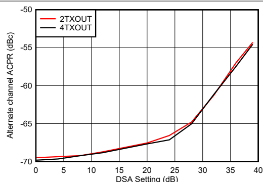
图 4-332. 0.85GHz 条件下 TX 20MHz LTE alt2-ACPR 与数字电平间的关系
