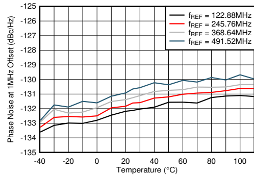
图 4-601. f_{\text{OUT}} = 2.6\text{GHz} 时 12GHz VCO 相位噪声 (1MHz 偏移条件下) 与温度和 f_{\text{REF}} 间的关系
