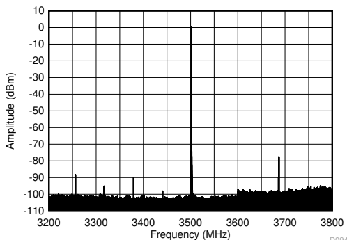
图 4-486. 3.5GHz ( \pm 300\text{MHz} ) 条件下的 TX 单音 ( -1\text{dBFS} ) 输出频谱
