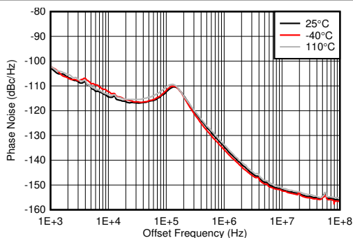
图 4-614. f_{\text{OUT}} = 2.6\text{GHz} 时 10GHz VCO 相位噪声 (5MHz 条件下) 与温度和 f_{\text{REF}} 间的关系
