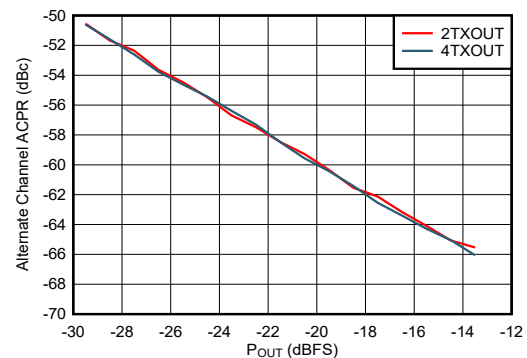
图 4-405. 2.6GHz 条件下 TX 20MHz LTE alt2-ACPR 与数字电平间的关系
