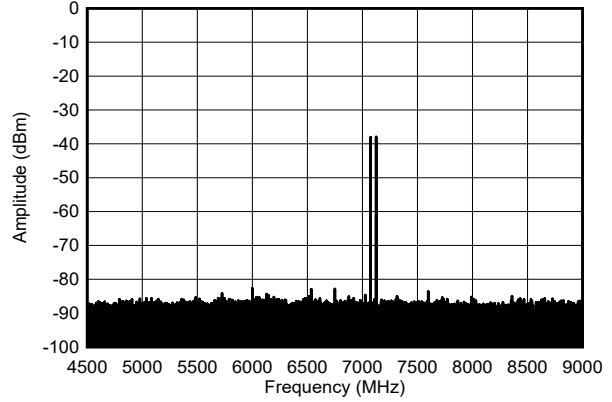
图 4-587. 7.1GHz、单音幅值为 -30dBFS (奈奎斯特) 条件下的双音输出频谱
