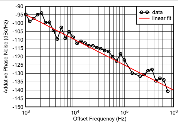
图 4-591. 9.61GHz 条件下的 RX 附加相位噪声
