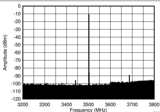
图 4-488. 3.5GHz ( \pm 300\text{MHz} ) 条件下的 TX 单音 ( -6\text{dBFS} ) 输出频谱
