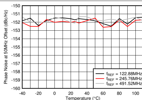
图 4-615. f_{\text{OUT}} = 2.6\text{GHz} 时 10GHz VCO 相位噪声 (50MHz 条件下) 与温度和 f_{\text{REF}} 间的关系
