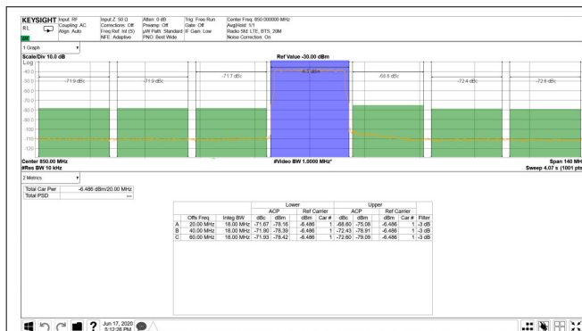
图 4-329. 0.85GHz 条件下 TX 20MHz LTE 输出频谱
