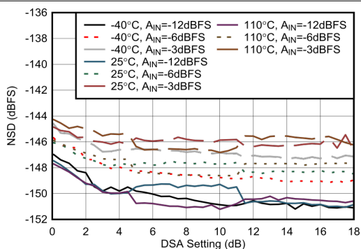
图 4-220. 6.851 GHz 条件下 RX NSD 与 DSA 设置间的关系
