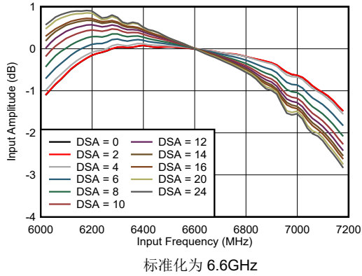
图 4-202. RX 带内增益平坦度
