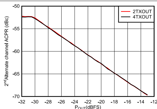
图 4-330. 0.85GHz 条件下 TX 20MHz LTE ACPR 与数字电平间的关系
