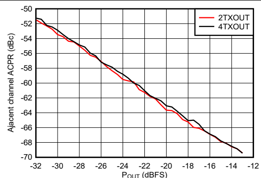
图 4-527. 4.9GHz 条件下 TX 20MHz LTE ACPR 与数字电平间的关系
