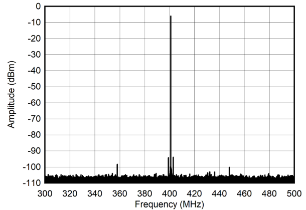
图 4-274. 400MHz 和 -12dBFS (±100MHz) 条件下的单音频谱
