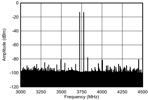
图 4-492. 3.75GHz、单音幅值为 -7dBFS ( \pm 600\text{MHz} ) 条件下的 TX 双音输出频谱
