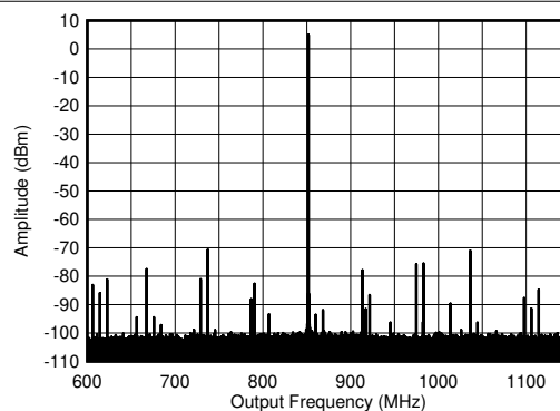
图 4-350. 0.85GHz ( \pm 300\text{MHz} ) 条件下的 TX 单频 (-6dBFS) 输出频谱
