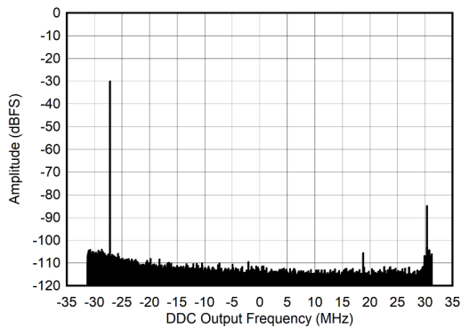
图 4-11. 5MHz 条件下的 RX 输出 FFT
