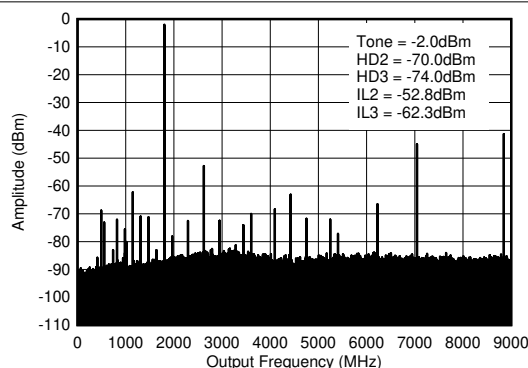
图 4-362. 1.8GHz ( 0-f_{\text{DAC}} ) 条件下的 TX 单频 (-12dBFS) 输出频谱
