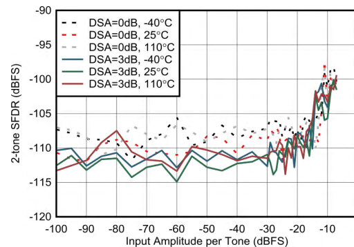
图 4-132. 2.6GHz 条件下 RX 带内 SFDR ( \pm 300\text{MHz} ) 与输入幅度和温度间的关系
