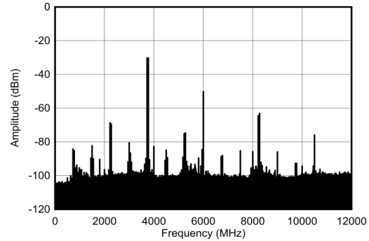
图 4-493. 3.75GHz、单音幅值为 -13dBFS ( 0 - f_{\text{DAC}} ) 条件下的 TX 双音输出频谱
