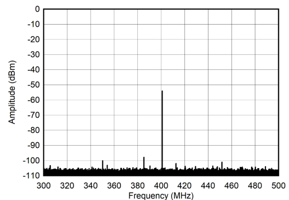
图 4-278. 400MHz 和 -60dBFS (±100MHz) 条件下的单音频谱
