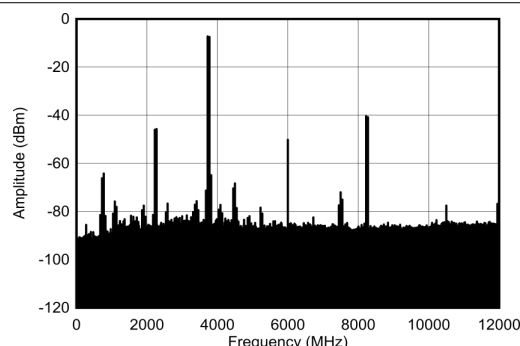
图 4-489. 3.5GHz ( 0 - f_{\text{DAC}} ) 条件下的 TX 单音 ( -12\text{dBFS} ) 输出频谱
