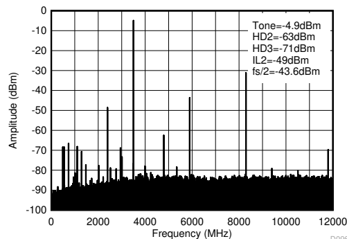
图 4-487. 3.5GHz ( 0 - f_{\text{DAC}} ) 条件下的 TX 单音 ( -6\text{dBFS} ) 输出频谱
