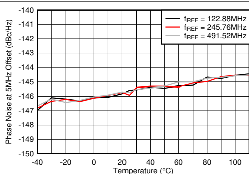
图 4-614. f_{\text{OUT}} = 2.6\text{GHz} 时 10GHz VCO 相位噪声 (5MHz 条件下) 与温度和 f_{\text{REF}} 间的关系
