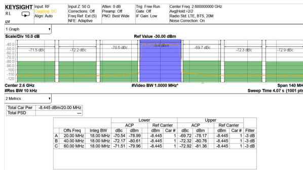
图 4-402. 2.6GHz (频带 41) 条件下的 TX 20MHz LTE 输出频谱
