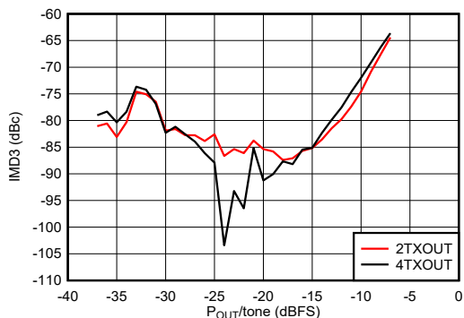
图 4-325. 0.85GHz 条件下 TX IMD3 与数字电平间的关系
