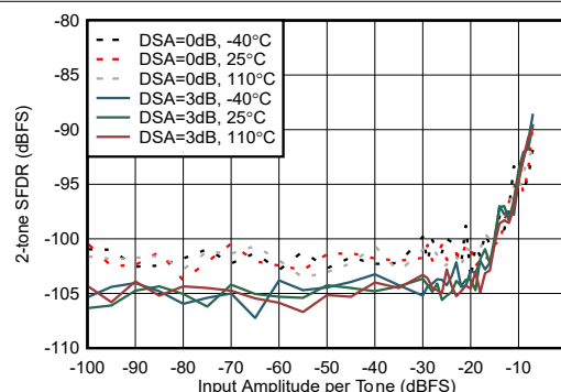
图 4-168. 3.7GHz 条件下 RX 双频 SFDR 与输入幅度和 DSA 设置间的关系
