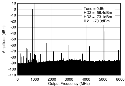
图 4-341. 0.85GHz ( 0-f_{\text{DAC}} ) 条件下的 TX 单频 (-12dBFS) 输出频谱
