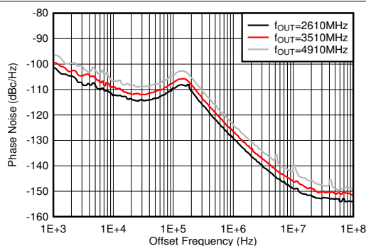
图 4-617. 25^\circ\text{C} 条件下 9GHz VCO 相位噪声与偏移频率和 f_{\text{OUT}} 间的关系
