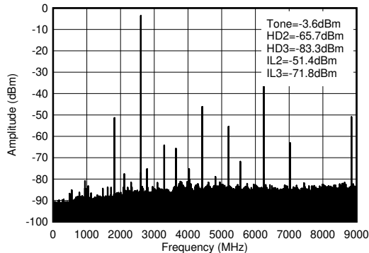
图 4-416. 2.6GHz ( 0-f_{\text{DAC}} ) 条件下的 TX 单频 ( -12\text{dBFS} ) 输出频谱
