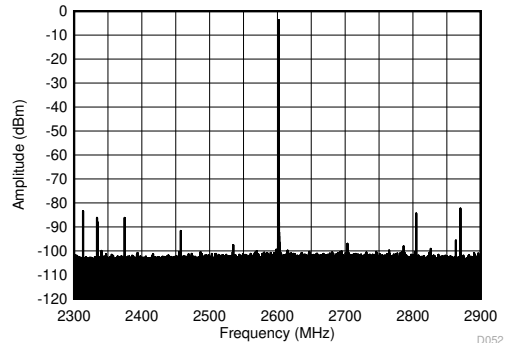
图 4-417. 2.6GHz ( \pm 300\text{MHz} ) 条件下的 TX 单音 ( -12\text{dBFS} ) 输出频谱
