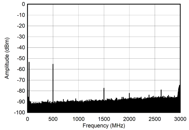
图 4-248. 30MHz 和 -60dBFS (奈奎斯特) 条件下的单音频谱
