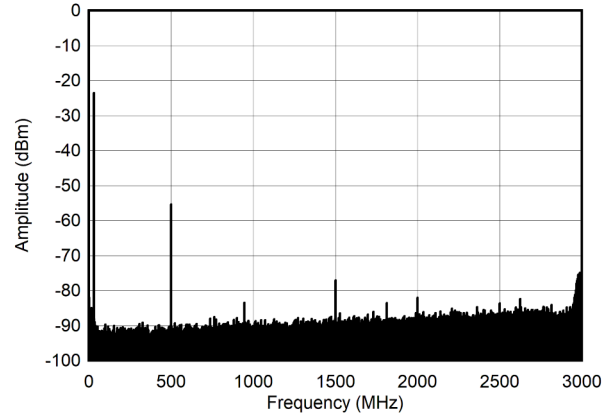
图 4-246. 30MHz 和 -30dBFS (奈奎斯特) 条件下的单音频谱
