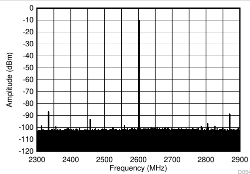
图 4-421. 2.6GHz ( \pm 300\text{MHz} ) 条件下的 TX 单音 (-1dBFS) 输出频谱
