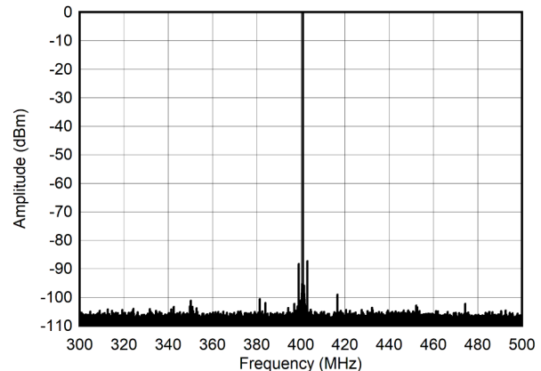
图 4-272. 400MHz 和 -6dBFS ( \pm 100\text{MHz} ) 条件下的单音频谱
