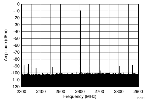
图 4-415. 2.6GHz 条件下双频带内固定杂散与数字振幅间的关系
