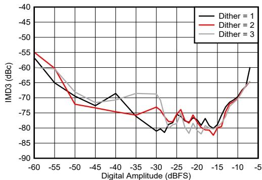
图 4-470. 3.75GHz 条件下 TX IMD3 与数字振幅和抖动间的关系
