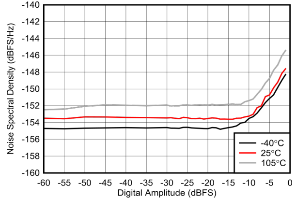
图 4-575. 7.1GHz 条件下 NSD 与数字振幅和温度间的关系
