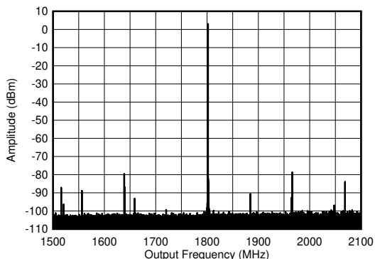
图 4-365. 1.8GHz ( \pm 300\text{MHz} ) 条件下的 TX 单音 (-6dBFS) 输出频谱
