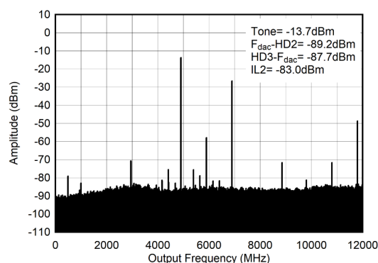
图 4-539. 4.9GHz ( 0-f_{\text{DAC}} ) 条件下的 TX 单频 ( -6\text{dBFS} ) 输出频谱
