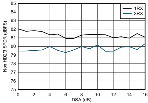
图 4-199. 4.9GHz 条件下 RX 非 HD2/3 与 DSA 设置间的关系
