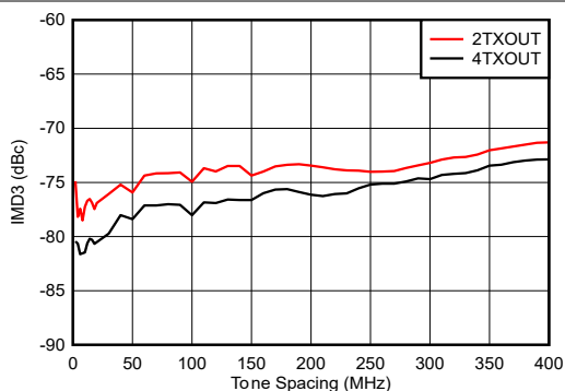
图 4-319. 0.85GHz 条件下 TX IMD3 与频率间隔和通道间的关系
