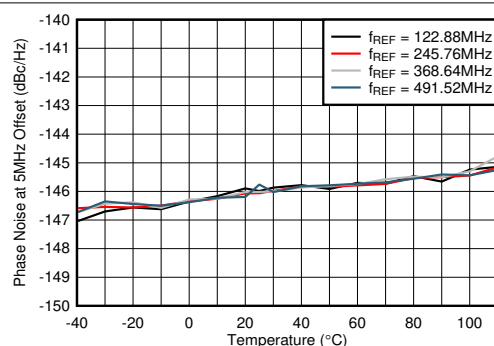
图 4-603. f_{\text{OUT}} = 2.6\text{GHz} 时 12GHz VCO 相位噪声 (5MHz 偏移条件下) 与温度和 f_{\text{REF}} 间的关系
