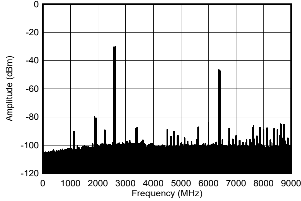
图 4-432. 2.6GHz、单音幅值为 -30dBFS (0 - D_{\text{AC}} ) 条件下的 TX 双音输出频谱
