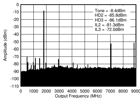
图 4-366. 1.8GHz ( 0-f_{\text{DAC}} ) 条件下的 TX 单频 (-1dBFS) 输出频谱
