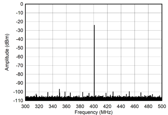
图 4-276. 400MHz 和 -30dBFS (±100MHz) 条件下的单音频谱
