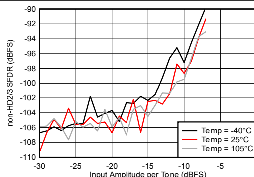
图 4-221. 6.85GHz 条件下 RX 2 子载波 SFDR 与输入振幅间的关系
