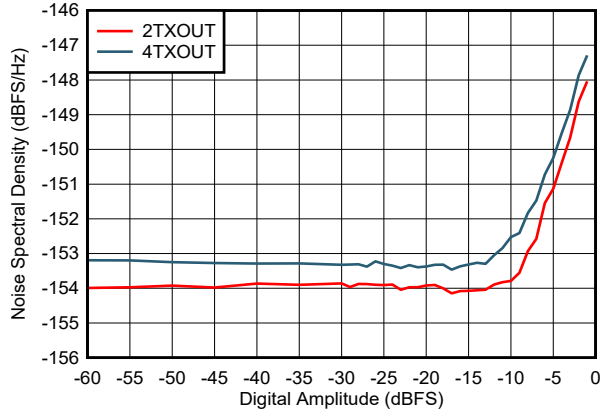
图 4-574. 7.1GHz 条件下 NSD 与数字振幅和通道间的关系
