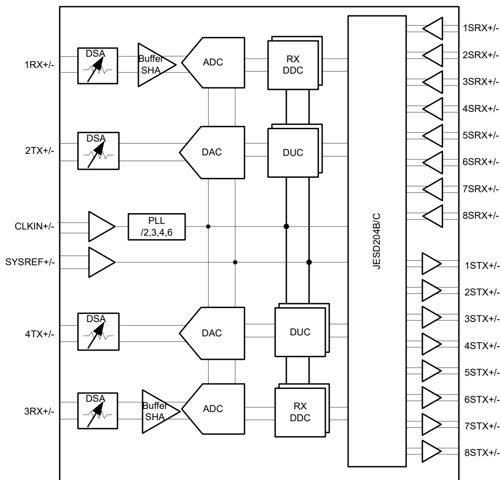
功能方框图
