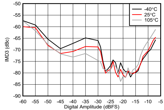
图 4-469. 3.75GHz 条件下 TX IMD3 与数字振幅和温度间的关系
