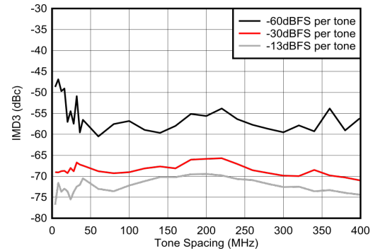
图 4-465. 3.5GHz 条件下 TX IMD3 与 DSA 设置间的关系
