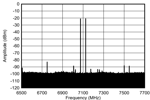
图 4-586. 7.1GHz、单音幅值为 -13dBFS (窄跨) 条件下的双音输出频谱
