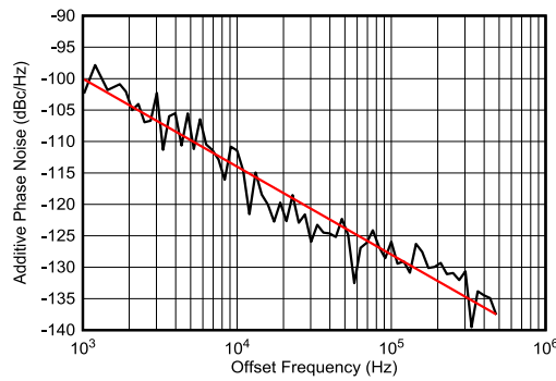
图 4-222. 6.85GHz 频率下的 RX 附加相位噪声
