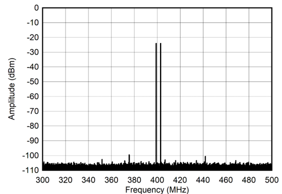
图 4-282. 400MHz 和 -13dBFS ( \pm 100\text{MHz} ) 条件下的双频频谱
