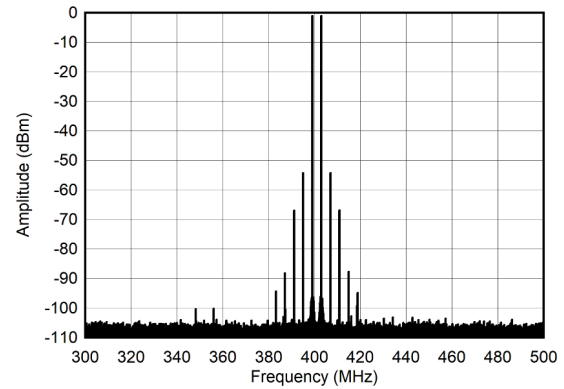
图 4-280. 400MHz 和 -7dBFS ( \pm 100\text{MHz} ) 条件下的双频频谱
