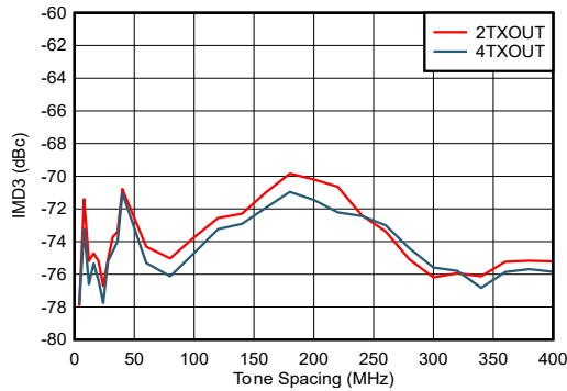
图 4-466. 3.5GHz 条件下 TX IMD3 与数字振幅和通道间的关系
