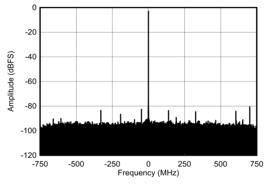
图 4-211. 6.851GHz 和 -3dBFS 条件下的 RX 输出 FFT
