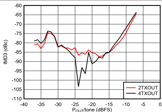
图 4-325. 0.85GHz 条件下 TX IMD3 与数字电平间的关系
