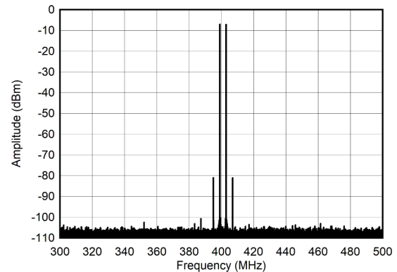
图 4-280. 400MHz 和 -7dBFS ( \pm 100\text{MHz} ) 条件下的双频频谱
