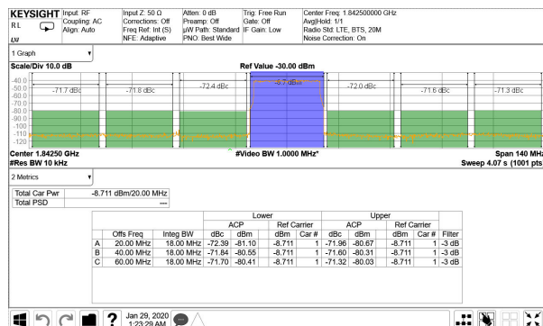
图 4-360. 1.8425GHz 条件下 TX 20MHz LTE 输出频谱
