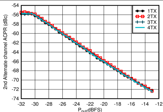
图 4-361. 1.8425GHz 条件下 TX 20MHz LTE ACPR 与数字电平间的关系
