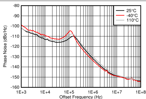
图 4-625. f_{\text{OUT}} = 1910\text{MHz} 时 8GHz VCO 相位噪声与偏移频率和温度间的关系
