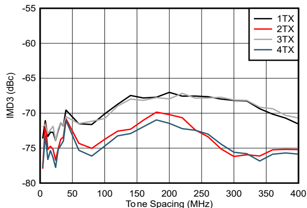
图 4-473. 3.75GHz 条件下 TX IMD3 与频率间隔和通道间的关系
