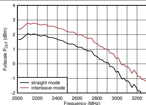
图 4-380. 5898.24MSPS 条件下 TX 满量程与射频频率间的关系
