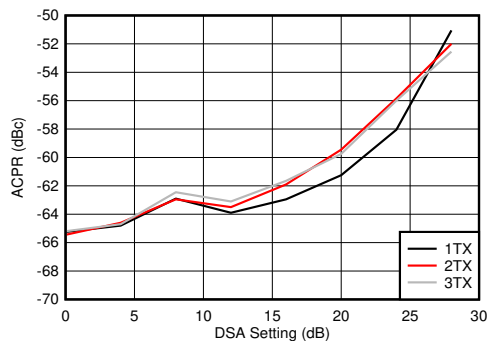
在 0.8GHz 条件下匹配, 单载波 100MHz BW TM1.1 NR
