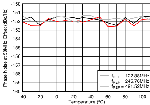
图 4-619. f_{\text{OUT}} = 2.6\text{GHz} 时 10GHz VCO 相位噪声 (50MHz 条件下) 与温度和 f_{\text{REF}} 间的关系
