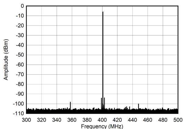
图 4-280. 400MHz 和 -12dBFS (±100MHz) 条件下的单音频谱
