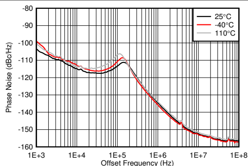
图 4-595. 12GHz 条件下 PLL 和外部时钟的相位噪声与偏移频率间的关系
