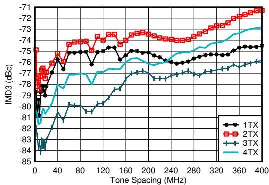
图 4-325. 0.85GHz 条件下 TX IMD3 与频率间隔和通道间的关系
