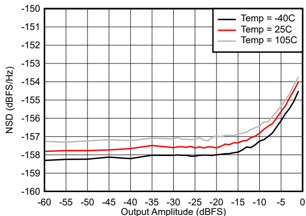
图 4-260. 30MHz 条件下的噪声频谱密度与数字振幅间的关系
