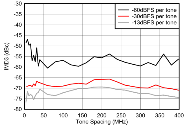
图 4-470. 3.5GHz 条件下 TX IMD3 与 DSA 设置间的关系
