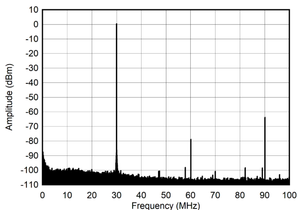
图 4-249. 30MHz 和 -6dBFS (0 - 100MHz) 条件下的单音频谱
