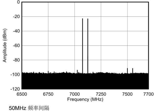
图 4-591. 7.1GHz、单音幅值为 -13dBFS (带内) 条件下的双音输出频谱
