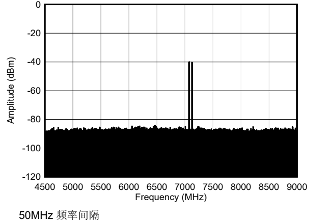
图 4-592. 7.1GHz、单音幅值为 -30dBFS (奈奎斯特) 条件下的双音输出频谱
