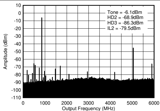
图 4-351. 0.85GHz ( 0-f_{\text{DAC}} ) 条件下的 TX 单频 ( -1\text{dBFS} ) 输出频谱
