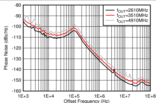
图 4-598. 25^\circ\text{C} 条件下 12GHz VCO 相位噪声与偏移频率和 f_{\text{OUT}} 间的关系
