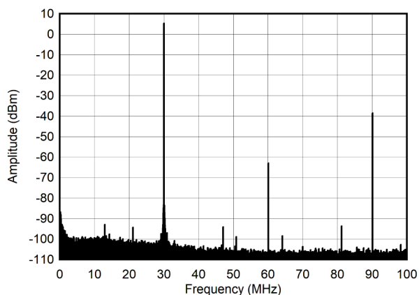
图 4-247. 30MHz 和 -1dBFS (0 - 100MHz) 条件下的单音频谱
