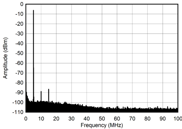
图 4-243. 5MHz 和 -12dBFS (0 - 100MHz) 条件下的单音频谱
