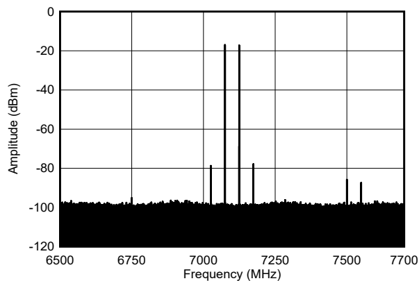
图 4-589. 7.1GHz、单音幅值为 -7dBFS (带内) 条件下的双音输出频谱
