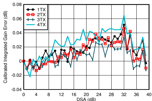
图 4-386. 2.6GHz 条件下 TX 校准差分增益误差与 DSA 设置和通道间的关系
