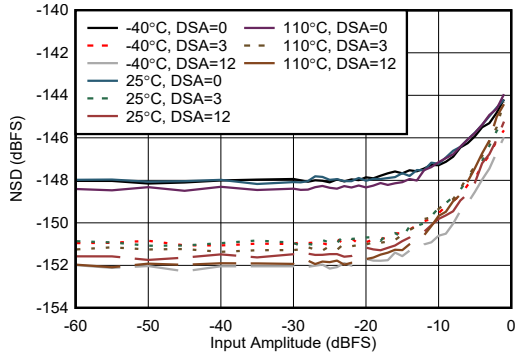
图 4-216. 6.851GHz 条件下 RX NSD 与输入振幅间的关系
