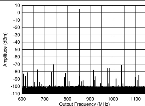
图 4-356. 0.85GHz ( \pm 300\text{MHz} ) 条件下的 TX 单音 (-6dBFS) 输出频谱
