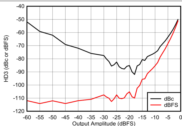
图 4-298. 400MHz 条件下 HD3 与振幅间的关系
