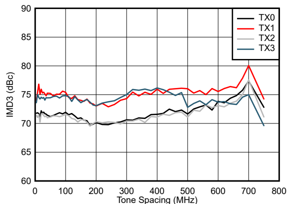
图 4-573. 7.1GHz 条件下 IMD3 与频率间隔和通道间的关系
