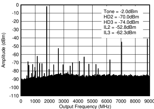
图 4-368. 1.8GHz ( 0-f_{\text{DAC}} ) 条件下的 TX 单频 (-12dBFS) 输出频谱
