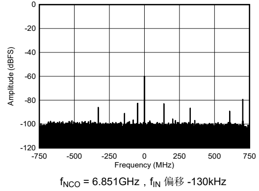
图 4-215. 6.851GHz 和 -60dBFS 条件下的 RX 输出 FFT
