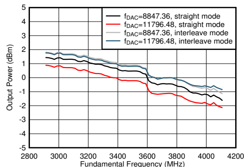
图 4-450. TX 输出功率与频率间的关系
