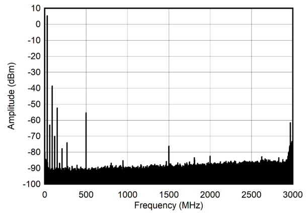
图 4-246. 30MHz 和 -1dBFS (奈奎斯特) 条件下的单音频谱
