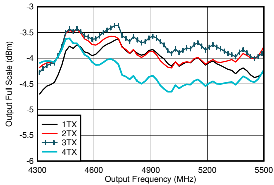
图 4-502. 11796.48MSPS 条件下的 TX 满量程与射频频率和通道间的关系
