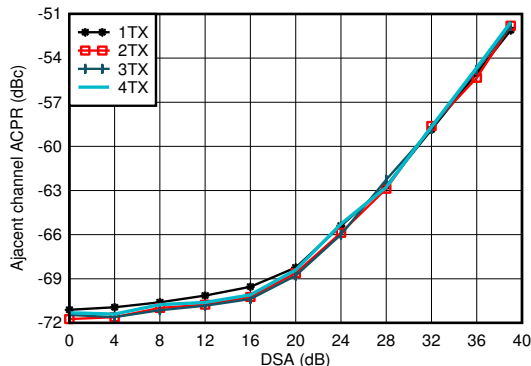
图 4-414. 2.6GHz 条件下 TX 20MHz LTE ACPR 与 DSA 间的关系
