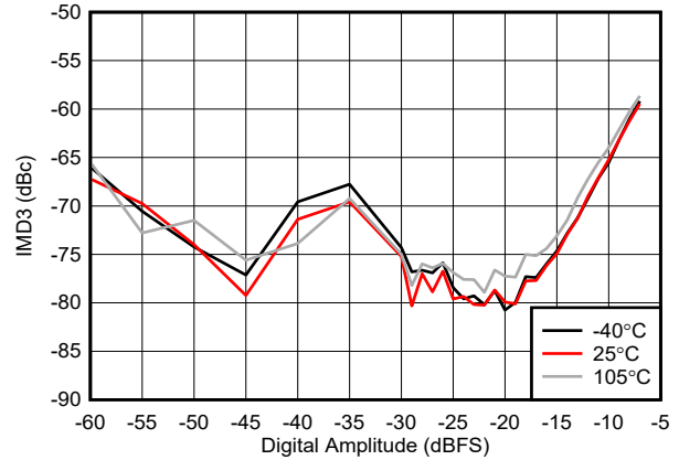
图 4-445. 2.6GHz 条件下 IMD3 与数字振幅和温度间的关系
