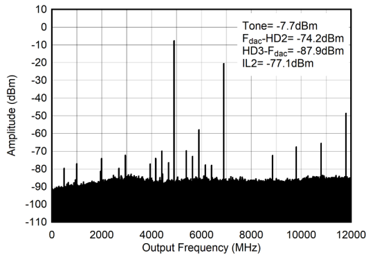
图 4-542. 4.9GHz ( 0-f_{\text{DAC}} ) 条件下的 TX 单频 ( -1\text{dBFS} ) 输出频谱
