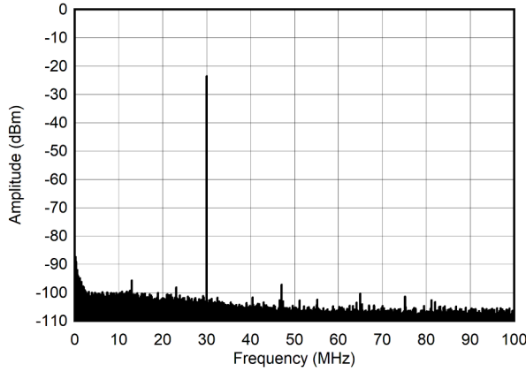
图 4-253. 30MHz 和 -30dBFS (0 - 100MHz) 条件下的单音频谱
