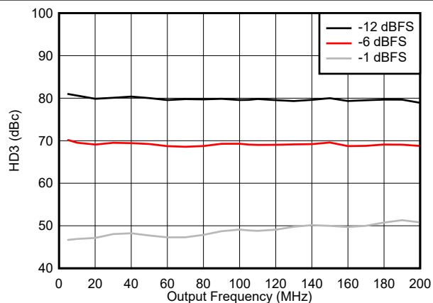
图 4-264. HD3 与频率 (0 - 200MHz) 间的关系
