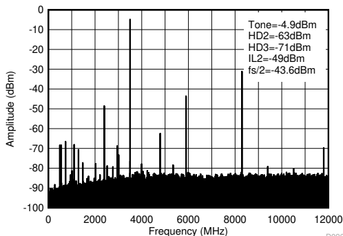
图 4-489. 3.5GHz (0 - f_{\text{DAC}} ) 条件下的 TX 单音 (-1dBFS) 输出频谱
