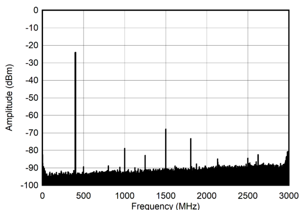
图 4-287. 400MHz 和 -13dBFS (奈奎斯特) 条件下的双频频谱
