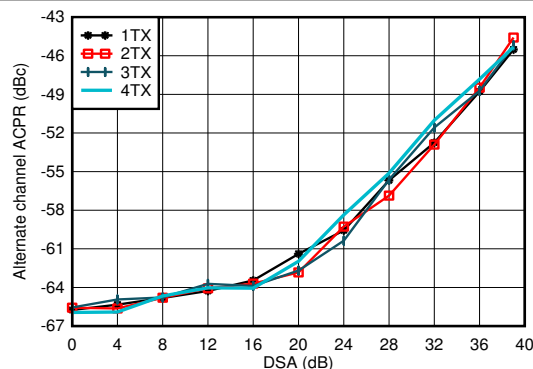
图 4-415. 2.6GHz 条件下 TX 20MHz LTE alt-ACPR 与 DSA 间的关系
