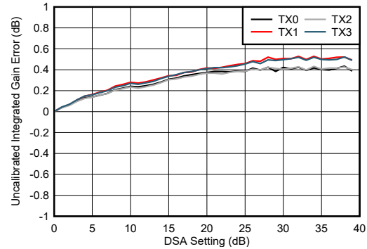
图 4-556. 7.1GHz 条件下未校准积分增益误差与通道间的关系
