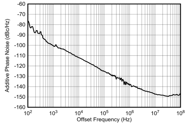
图 4-594. 7.1GHz 条件下的外部时钟附加相位噪声
