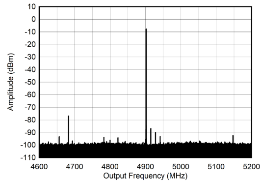
图 4-543. 4.9GHz ( \pm 300\text{MHz} ) 条件下的 TX 单音 ( -1\text{dBFS} ) 输出频谱
