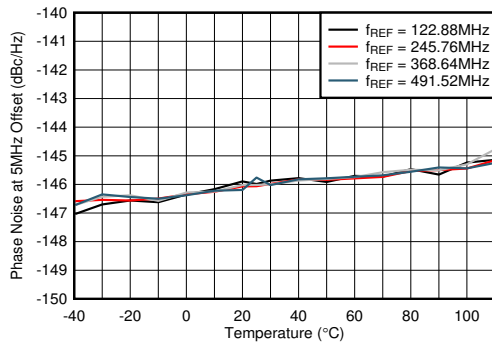
图 4-607. f_{\text{OUT}} = 2.6\text{GHz} 时 12GHz VCO 相位噪声 (5MHz 偏移条件下) 与温度和 f_{\text{REF}} 间的关系
