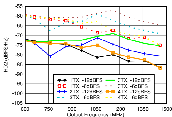
在 0.8GHz 条件下匹配, f_{\text{DAC}} = 5898.24\text{GSPS} , 直接模式
