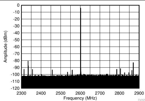
图 4-429. 2.6GHz ( \pm 300\text{MHz} ) 条件下的 TX 单音 (-12dBFS) 输出频谱
