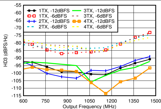
在 0.8 GHz 条件下匹配, f_{\text{DAC}} = 5898.24\text{MSPS} , 直接模式, 标准化为谐波频率下的输出功率
