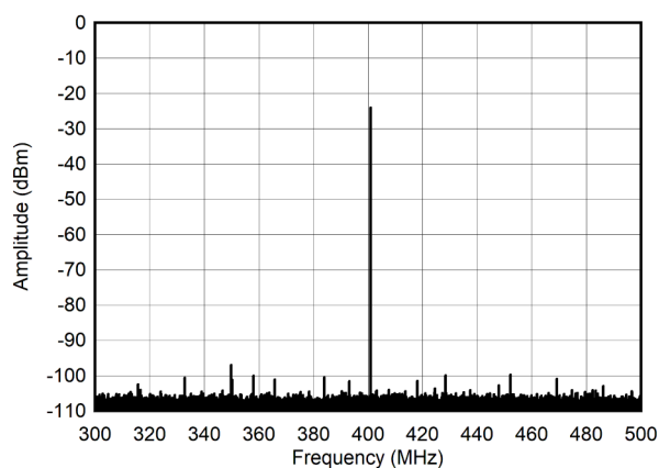
图 4-282. 400MHz 和 -30dBFS (±100MHz) 条件下的单音频谱
