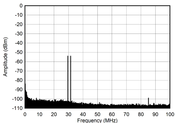
图 4-259. 30MHz 和 -60dBFS (0 - 100MHz) 条件下的双频频谱
