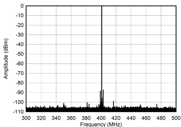
图 4-278. 400MHz 和 -6dBFS (±100MHz) 条件下的单音频谱
