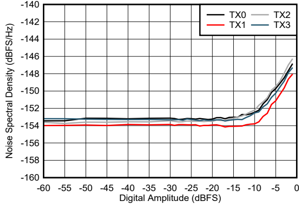
图 4-579. 7.1GHz 条件下 NSD 与数字振幅和通道间的关系
