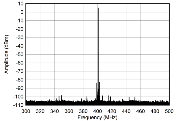
图 4-276. 400MHz 和 -1dBFS ( \pm 100\text{MHz} ) 条件下的单音频谱
