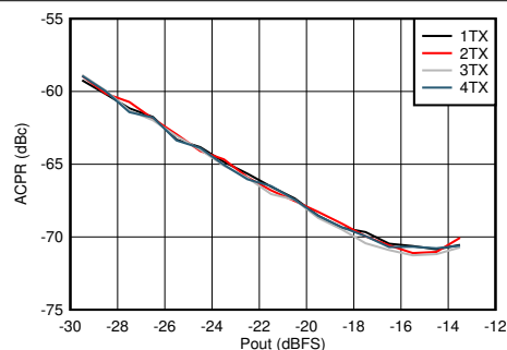
图 4-409. 2.6GHz 条件下 TX 20MHz LTE ACPR 与数字电平间的关系
