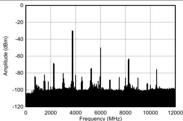
图 4-497. 3.75GHz、单音幅值为 -13dBFS ( 0 - f_{\text{DAC}} ) 条件下的 TX 双音输出频谱
