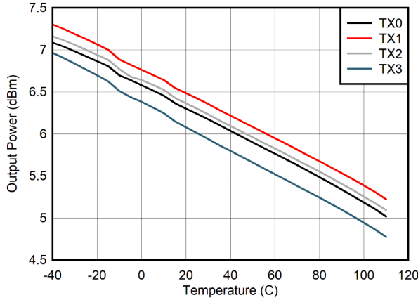
图 4-265. 400MHz 条件下 TX 输出满量程与温度间的关系
