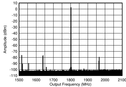
图 4-378. 1.8GHz ( 0-f_{\text{DAC}} ) 条件下的 TX 单频 ( -1\text{dBFS} ) 输出频谱
