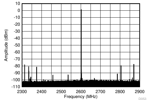
图 4-425. 2.6GHz ( \pm 300\text{MHz} ) 条件下的 TX 单音 (-6dBFS) 输出频谱
