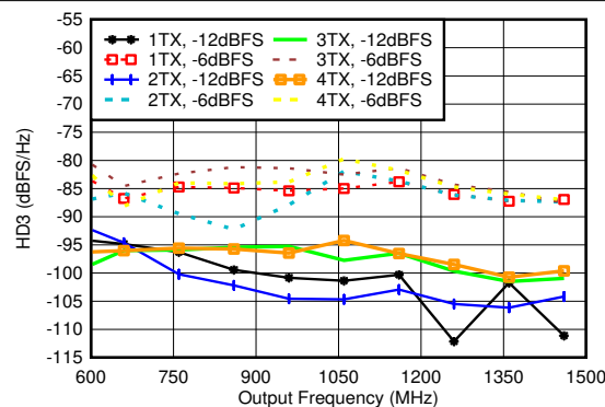
在 0.8 GHz 条件下匹配, f_{\text{DAC}} = 8847.36\text{MSPS} , 直接模式, 标准化为谐波频率下的输出功率
