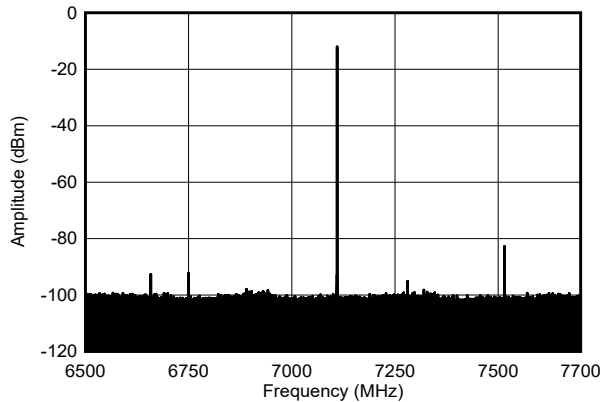
图 4-583. 7.1GHz、-1dBFS (带内) 条件下的单音输出频谱
