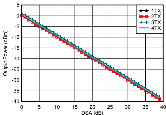
图 4-449. 3.5GHz 条件下 TX 输出功率与 DSA 设置间的关系
