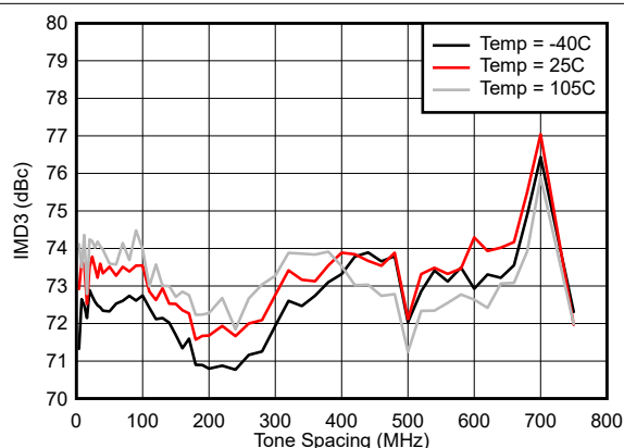
图 4-575. 7.1GHz 条件下 IMD3 与频率间隔和温度间的关系
