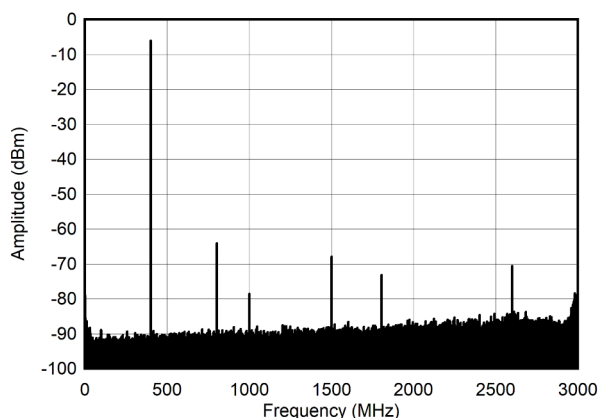
图 4-279. 400MHz 和 -12dBFS (奈奎斯特) 条件下的单音频谱
