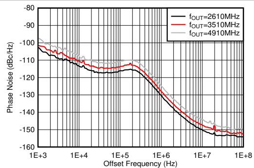
图 4-610. 25^\circ\text{C} 条件下 10GHz VCO 相位噪声与偏移频率和 f_{\text{OUT}} 间的关系
