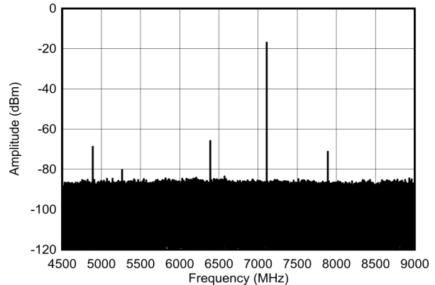
图 4-584. 7.1GHz、-6dBFS (奈奎斯特) 条件下的单音输出频谱
