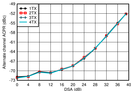
图 4-365. 1.8GHz 条件下 TX 20MHz LTE alt-ACPR 与 DSA 间的关系
