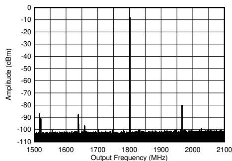
图 4-373. 1.8GHz ( \pm 300\text{MHz} ) 条件下的 TX 单音 ( -1\text{dBFS} ) 输出频谱
