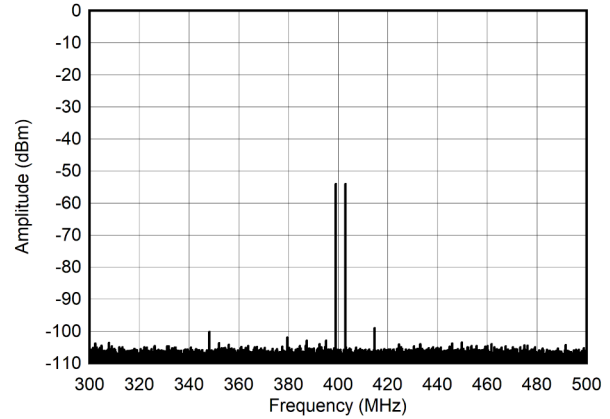
图 4-292. 400MHz 和 -60dBFS (±100MHz) 条件下的双频频谱
