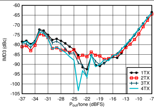
图 4-331. 0.85GHz 条件下 TX IMD3 与数字电平间的关系
