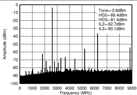
图 4-428. 2.6GHz ( 0-f_{\text{DAC}} ) 条件下的 TX 单频 (-12dBFS) 输出频谱
