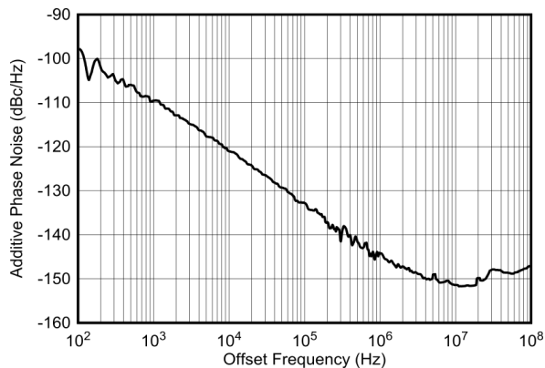
图 4-448. 2.6GHz 条件下的外部时钟附加相位噪声
