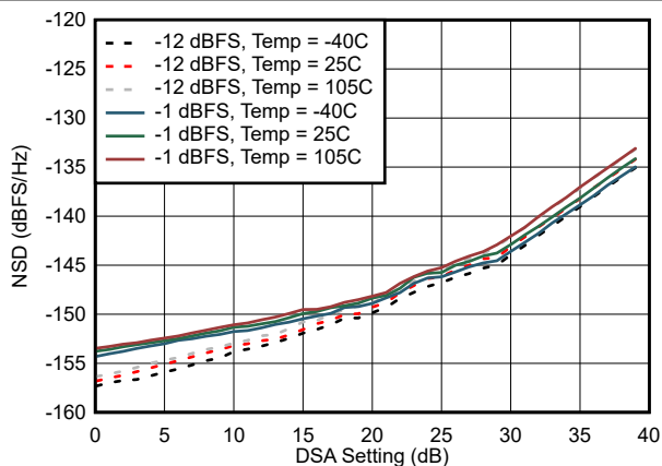
图 4-261. 30MHz 条件下的噪声频谱密度与 DSA 设置间的关系
