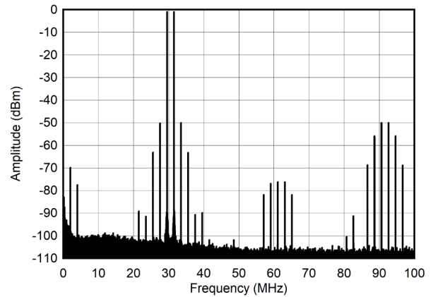
图 4-256. 30MHz 和 -7dBFS (0 - 100MHz) 条件下的双频频谱
