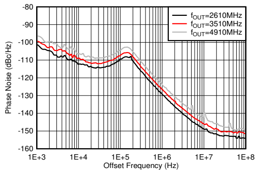
图 4-621. 25^\circ\text{C} 条件下 9GHz VCO 相位噪声与偏移频率和 f_{\text{OUT}} 间的关系
