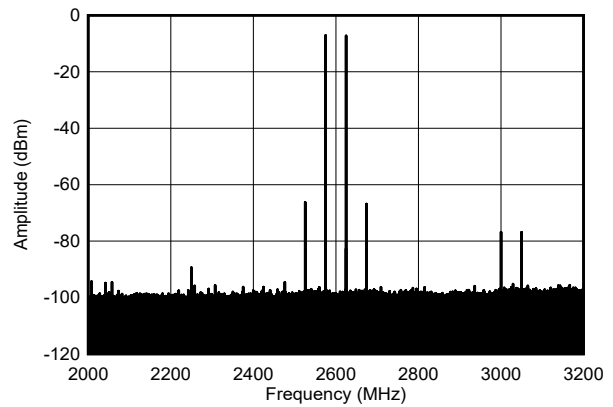
图 4-433. 2.6GHz ( \pm 300\text{MHz} ) 条件下的 TX 单音 (-1dBFS) 输出频谱
