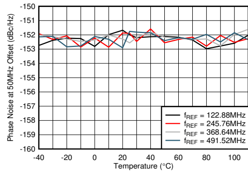
图 4-608. f_{\text{OUT}} = 2.6\text{GHz} 时 12GHz VCO 相位噪声 (50MHz 偏移条件下) 与温度和 f_{\text{REF}} 间的关系
