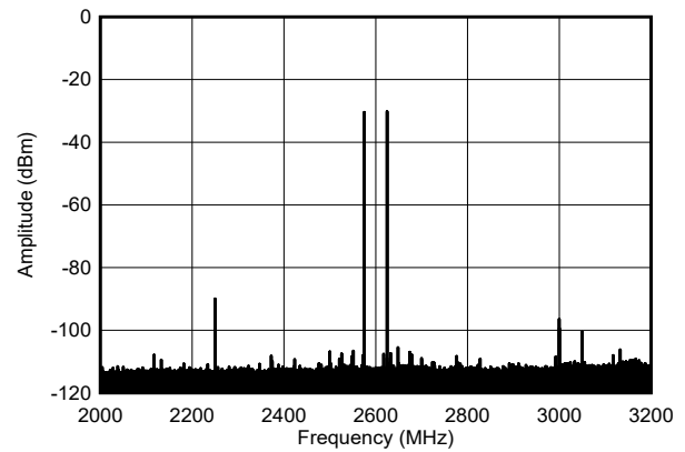
图 4-437. 2.6GHz、单音幅值为 -13dBFS ( \pm 600\text{MHz} ) 条件下的 TX 双音输出频谱
