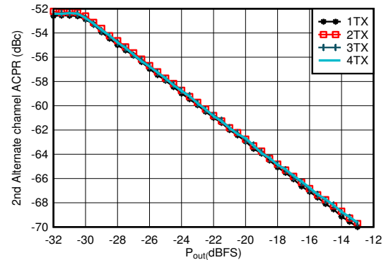
图 4-336. 0.85GHz 条件下 TX 20MHz LTE ACPR 与数字电平间的关系
