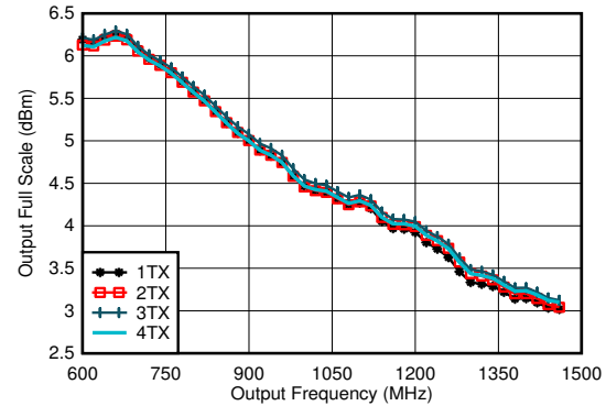
图 4-300. 8847.36MSPS 条件下 TX 满量程与射频频率和通道间的关系, 直接模式
