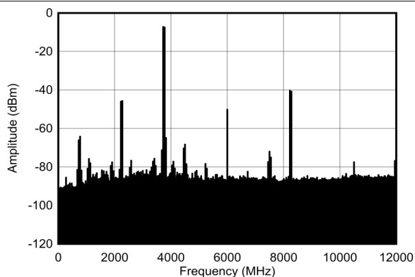
图 4-493. 3.5GHz ( 0-f_{\text{DAC}} ) 条件下的 TX 单频 (-12dBFS) 输出频谱
