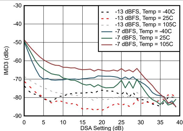
图 4-262. 30MHz 条件下 IMD3 与 DSA 设置间的关系
