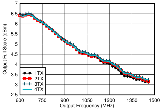
图 4-299. 5898.24MSPS 条件下 TX 满量程与射频频率和通道间的关系, 直接模式
