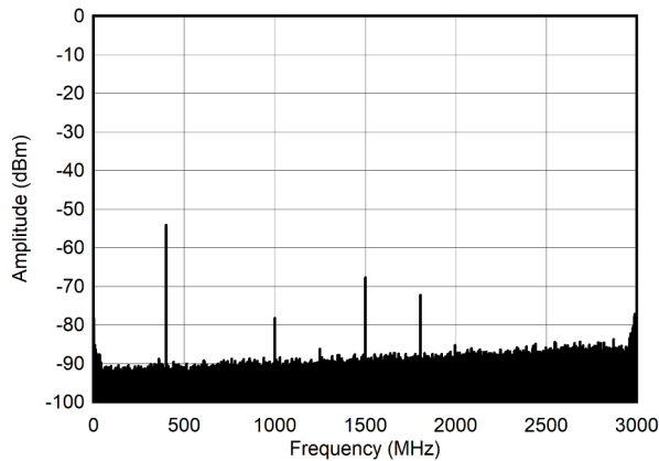
图 4-283. 400MHz 和 -60dBFS (奈奎斯特) 条件下的单音频谱
