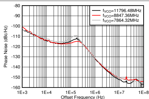
图 4-596. f_{\text{OUT}} = 2610\text{MHz} 时相位噪声与偏移频率和 f_{\text{VCO}} 间的关系
