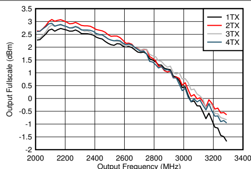
图 4-381. 8847.36MSPS 条件下 TX 满量程与射频频率间的关系
