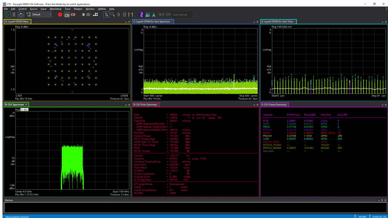
图 4-547. 4.9GHz ( \pm 300\text{MHz} ) 条件下的 TX 单音 (-12dBFS) 输出频谱
