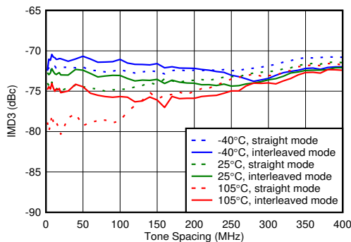
图 4-404. 2.6GHz 条件下 TX IMD3 与频率间隔和温度间的关系
