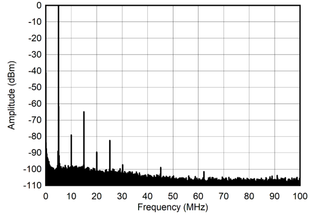
图 4-242. 5MHz 和 -6dBFS (0 - 100MHz) 条件下的单音频谱
