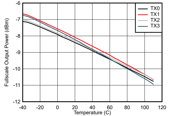
图 4-550. 7.1GHz 条件下 TX 满量程与温度和通道间的关系
