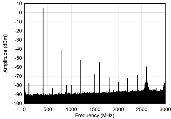
图 4-275. 400MHz 和 -1dBFS (奈奎斯特) 条件下的单音频谱
