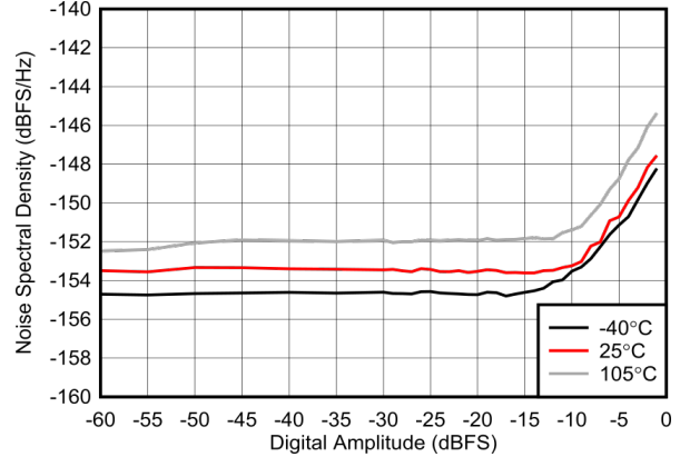
图 4-580. 7.1GHz 条件下 NSD 与数字振幅和温度间的关系
