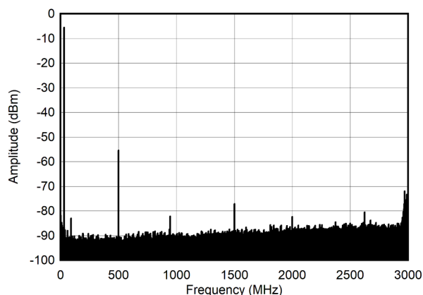
图 4-250. 30MHz 和 -12dBFS (奈奎斯特) 条件下的单音频谱
