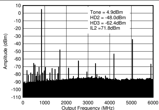
图 4-355. 0.85GHz ( 0-f_{\text{DAC}} ) 条件下的 TX 单频 (-6dBFS) 输出频谱
