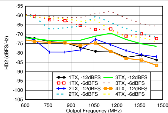
在 0.8GHz 条件下匹配, f_{\text{DAC}} = 8847.36\text{GSPS} , 直接模式
