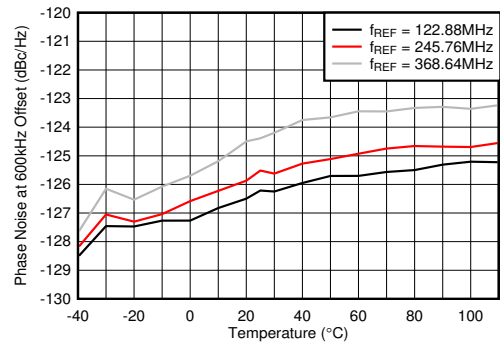
图 4-614. f_{\text{OUT}} = 2.6\text{GHz} 时 10GHz VCO 相位噪声 (600kHz 条件下) 与温度和 f_{\text{REF}} 间的关系
