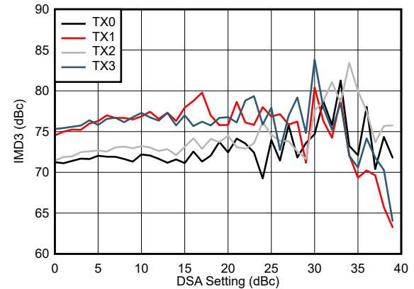
图 4-568. 7.1GHz 条件下 IMD3 与数字振幅和通道间的关系
