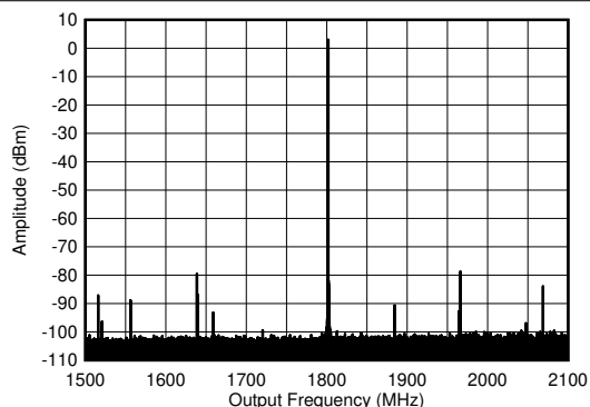
图 4-371. 1.8GHz ( \pm 300\text{MHz} ) 条件下的 TX 单音 ( -6\text{dBFS} ) 输出频谱
