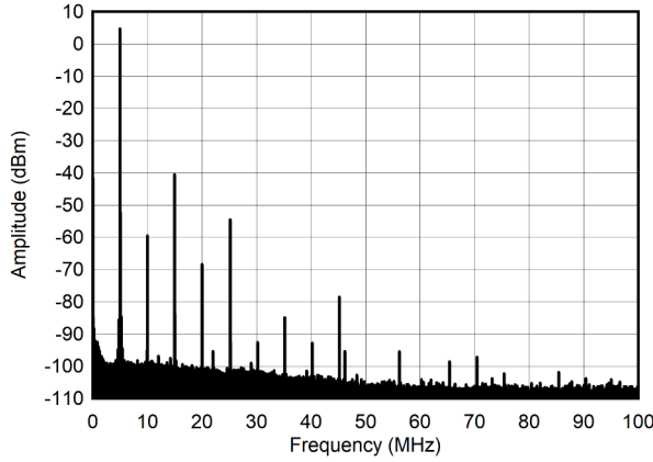
图 4-241. 5MHz 和 -1dBFS (0 - 100MHz) 条件下的单音频谱
