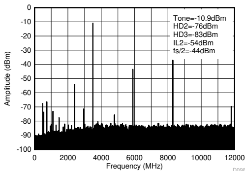
图 4-493. 3.5GHz ( 0-f_{\text{DAC}} ) 条件下的 TX 单频 (-12dBFS) 输出频谱
