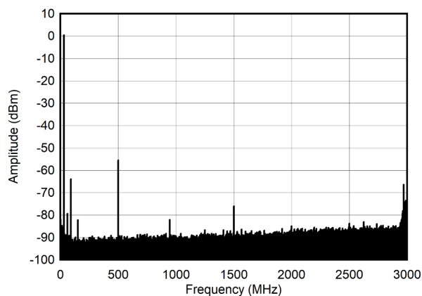
图 4-248. 30MHz 和 -6dBFS (奈奎斯特) 条件下的单音频谱
