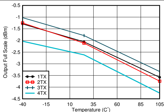
图 4-506. 4.9GHz 条件下 TX 满量程输出功率与温度和通道间的关系
