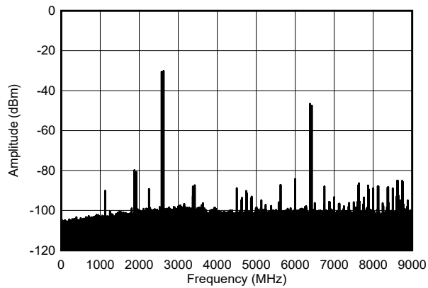
图 4-436. 2.6GHz、单音幅值为 -13dBFS (0 - DAC) 条件下的 TX 双音输出频谱
