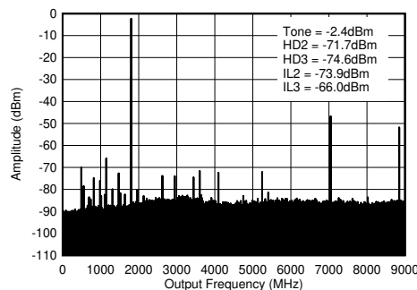
图 4-374. 1.8GHz ( 0-f_{\text{DAC}} ) 条件下的 TX 单频 ( -12\text{dBFS} ) 输出频谱
