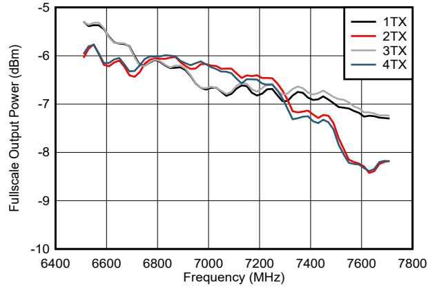
图 4-549. TX 满量程与射频频率和通道间的关系
