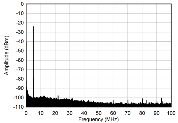
图 4-244. 5MHz 和 -30dBFS (0 - 100MHz) 条件下的单音频谱
