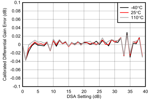
图 4-555. 7.1GHz 条件下校准差分增益误差与温度间的关系
