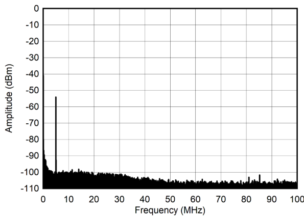
图 4-245. 5MHz 和 -60dBFS (0 - 100MHz) 条件下的单音频谱
