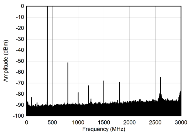
图 4-277. 400MHz 和 -6dBFS (奈奎斯特) 条件下的单音频谱
