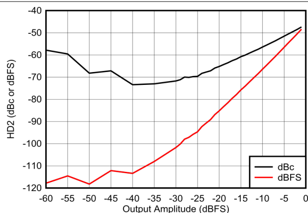
图 4-297. 400MHz 条件下 HD2 与振幅间的关系
