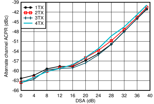
图 4-539. 4.9GHz 条件下 TX 100MHz NR alt-ACPR 与 DSA 间的关系
