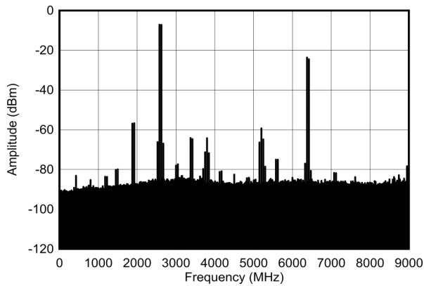
图 4-432. 2.6GHz (0- f_{\text{DAC}} ) 条件下的 TX 单频 (-1dBFS) 输出频谱
