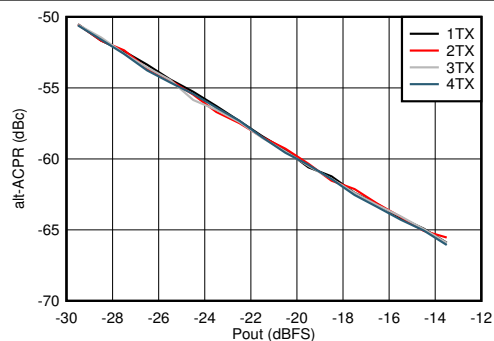
图 4-411. 2.6GHz 条件下 TX 20MHz LTE alt2-ACPR 与数字电平间的关系
