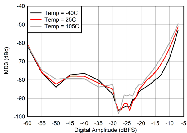
图 4-295. 400MHz 条件下 IMD3 与数字振幅间的关系
