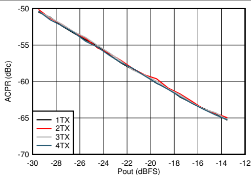
图 4-410. 2.6GHz 条件下 TX 20MHz LTE alt-ACPR 与数字电平间的关系
