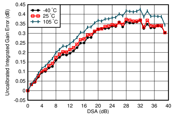
图 4-511. 4.9GHz 条件下 TX 未校准差分增益误差与 DSA 设置和温度间的关系
