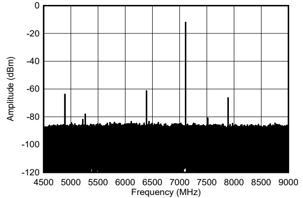
图 4-582. 7.1GHz、-1dBFS (奈奎斯特) 条件下的单音输出频谱
