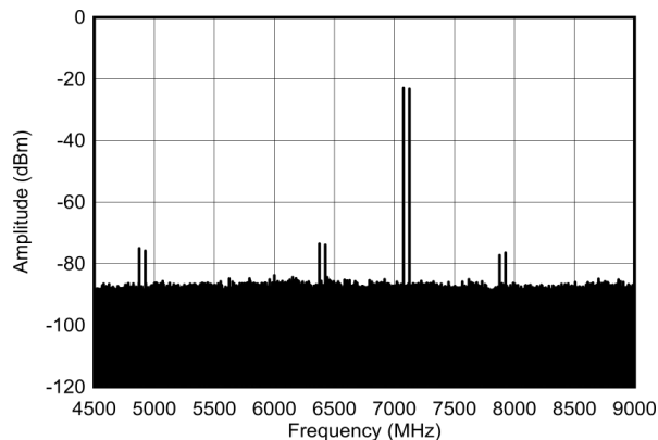
图 4-588. 7.1GHz、单音幅值为 -7dBFS (奈奎斯特) 条件下的双音输出频谱
