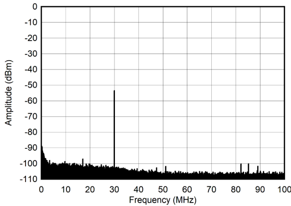
图 4-255. 30MHz 和 -60dBFS (0 - 100MHz) 条件下的单音频谱
