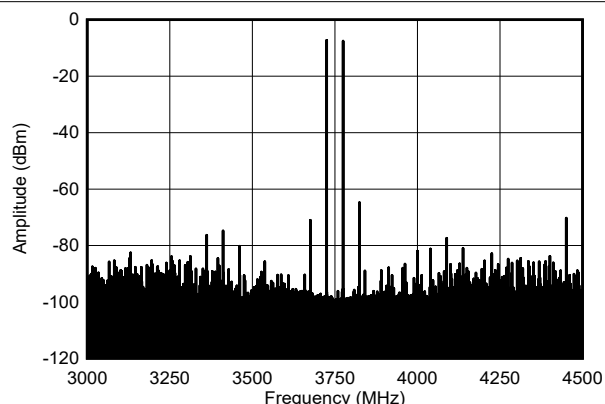
图 4-494. 3.5GHz ( \pm 300\text{MHz} ) 条件下的 TX 单音 (-12dBFS) 输出频谱
