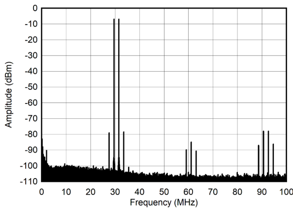
图 4-257. 30MHz 和 -13dBFS (0 - 100MHz) 条件下的双频频谱
