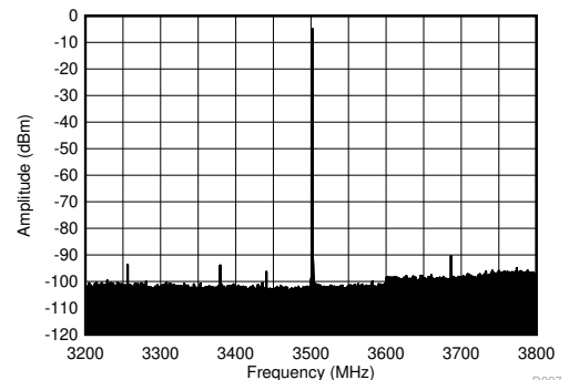
图 4-490. 3.5GHz ( \pm 300\text{MHz} ) 条件下的 TX 单音 (-1dBFS) 输出频谱
