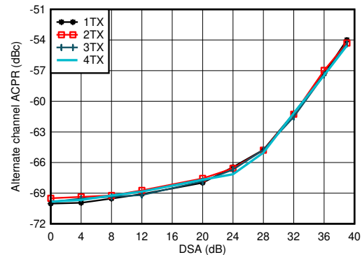
图 4-338. 0.85GHz 条件下 TX 20MHz LTE alt2-ACPR 与数字电平间的关系
