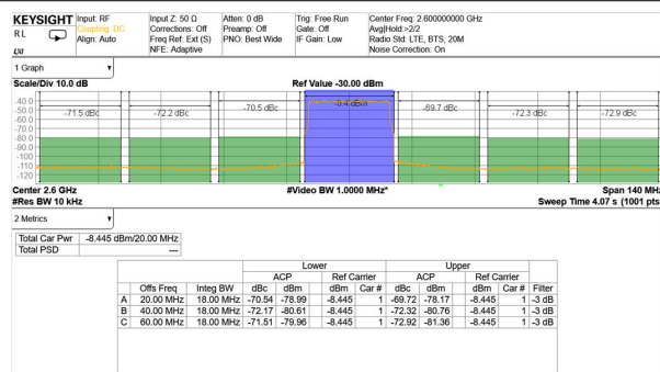
图 4-408. 2.6GHz (频带 41) 条件下的 TX 20MHz LTE 输出频谱
