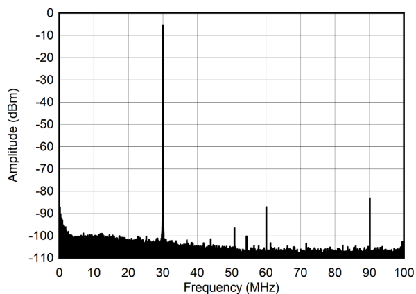
图 4-251. 30MHz 和 -12dBFS (0 - 100MHz) 条件下的单音频谱
