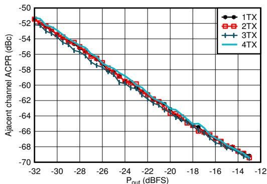
图 4-532. 4.9GHz 条件下 TX 20MHz LTE ACPR 与数字电平间的关系
