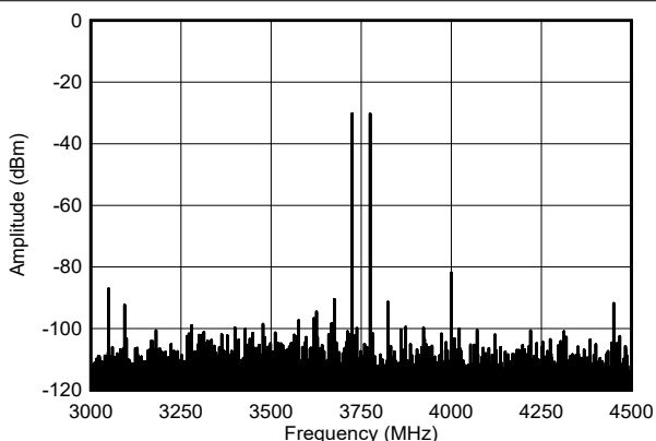
图 4-498. 3.75GHz、单音幅值为 -13dBFS ( \pm 600\text{MHz} ) 条件下的 TX 双音输出频谱
