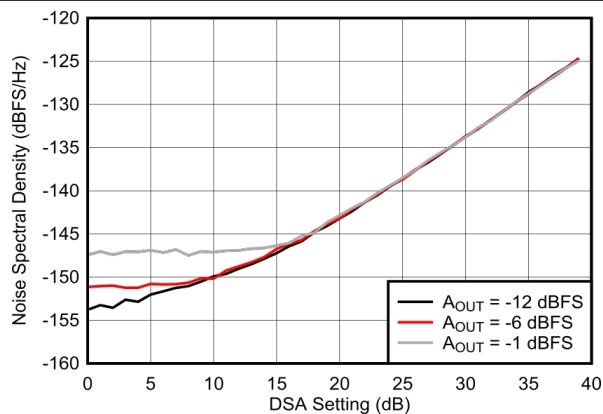
图 4-577. 7.1GHz 条件下 NSD 与 DSA 设置和振幅间的关系
