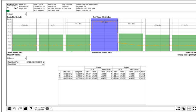
图 4-335. 0.85GHz 条件下 TX 20MHz LTE 输出频谱
