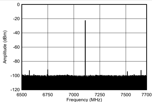
图 4-587. 7.1GHz、-12dBFS (带内) 条件下的单音输出频谱
