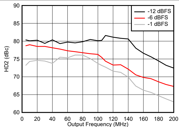
图 4-263. HD2 与频率 (0 - 200MHz) 间的关系
