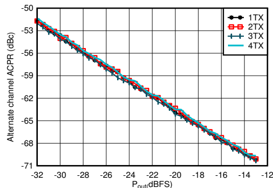
图 4-533. 4.9GHz 条件下 TX 20MHz LTE alt-ACPR 与数字电平间的关系
