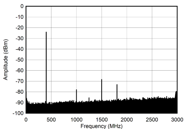
图 4-281. 400MHz 和 -30dBFS (奈奎斯特) 条件下的单音频谱
