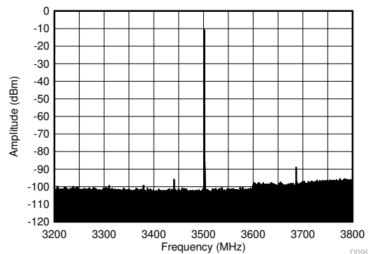
图 4-494. 3.5GHz ( \pm 300\text{MHz} ) 条件下的 TX 单音 (-12dBFS) 输出频谱
