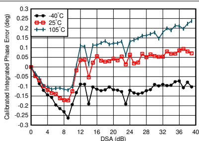
图 4-398. 2.6GHz 条件下 TX 校准差分相位误差与 \text{DSA} 设置和温度间的关系
