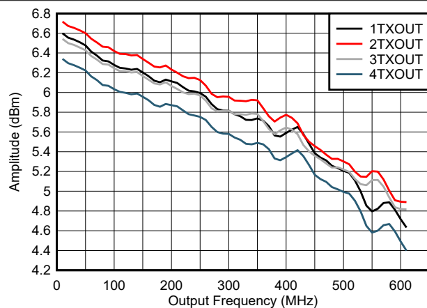
图 4-229. TX 输出满量程与输出频率间的关系：5MHz 至 600MHz
