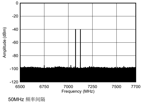
图 4-593. 7.1GHz、单音幅值为 -30dBFS (带内) 条件下的双音输出频谱
