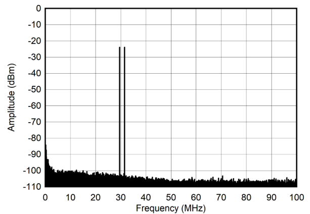
图 4-258. 30MHz 和 -30dBFS (0 - 100MHz) 条件下的双频频谱
