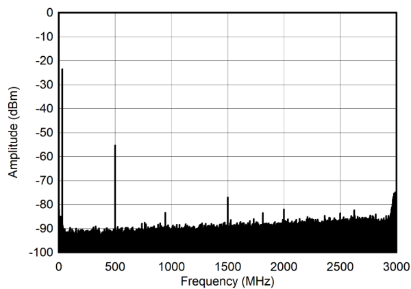
图 4-252. 30MHz 和 -30dBFS (奈奎斯特) 条件下的单音频谱
