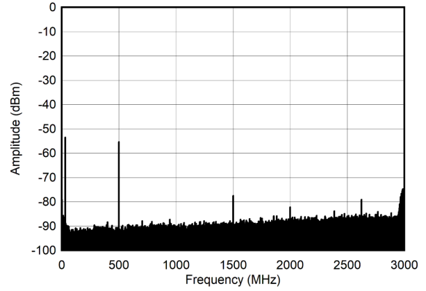
图 4-254. 30MHz 和 -60dBFS (奈奎斯特) 条件下的单音频谱
