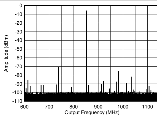
图 4-352. 0.85GHz ( \pm 300\text{MHz} ) 条件下的 TX 单音 ( -1\text{dBFS} ) 输出频谱
