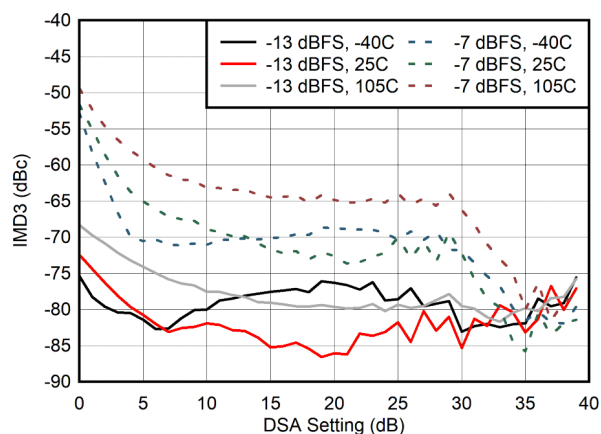
图 4-296. 400MHz 条件下 IMD3 与 DSA 设置间的关系
