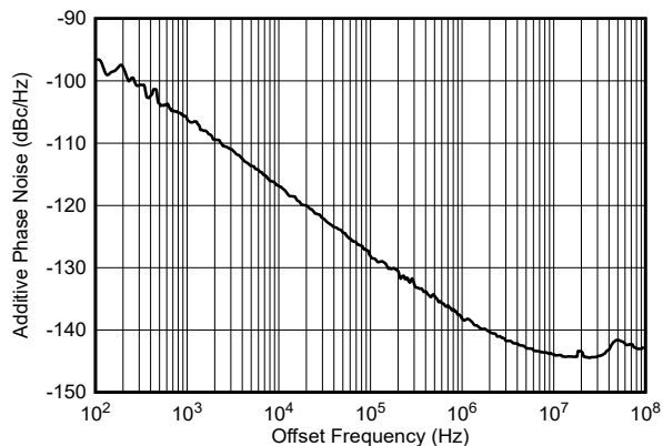
图 4-501. 3.7GHz 条件下的外部时钟附加相位噪声
