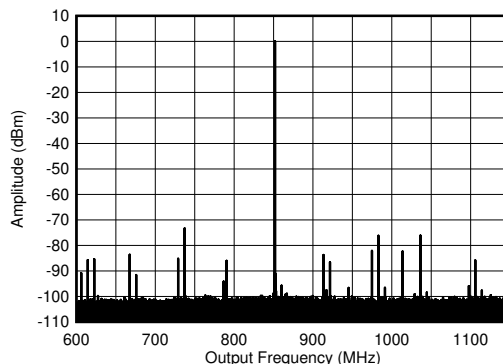
图 4-348. 0.85GHz ( \pm 300\text{MHz} ) 条件下的 TX 单音 (-12dBFS) 输出频谱
