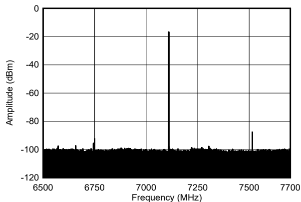
图 4-585. 7.1GHz、-6dBFS (带内) 条件下的单音输出频谱
