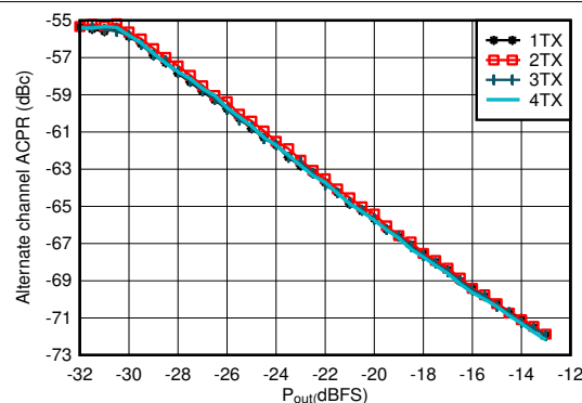
图 4-362. 1.8425GHz 条件下 TX 20MHz LTE alt-ACPR 与数字电平间的关系
