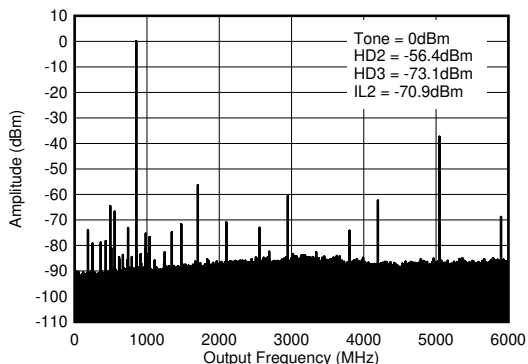
图 4-347. 0.85GHz ( 0-f_{\text{DAC}} ) 条件下的 TX 单频 (-12dBFS) 输出频谱
