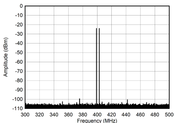
图 4-288. 400MHz 和 -13dBFS ( \pm 100\text{MHz} ) 条件下的双频频谱
