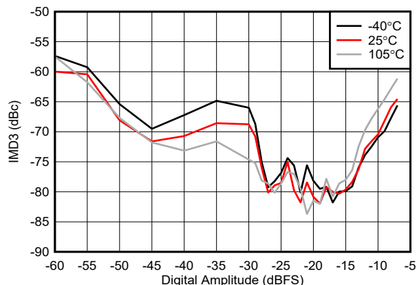
图 4-474. 3.75GHz 条件下 TX IMD3 与数字振幅和温度间的关系
