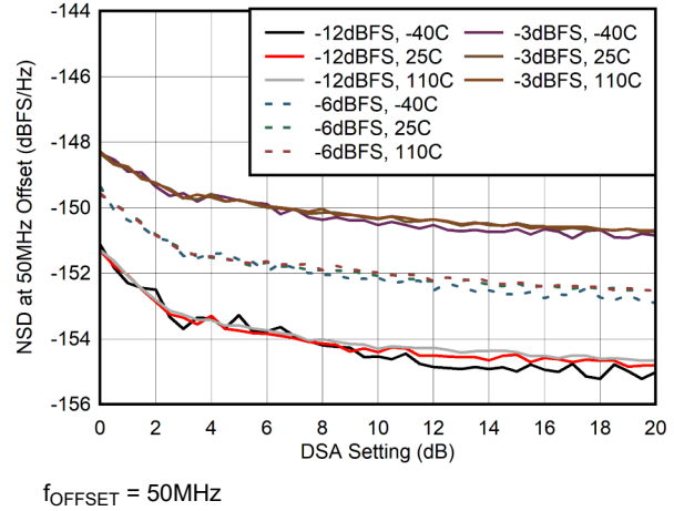
图 4-44. 400MHz 条件下 NSD 与 DSA 设置间的关系
