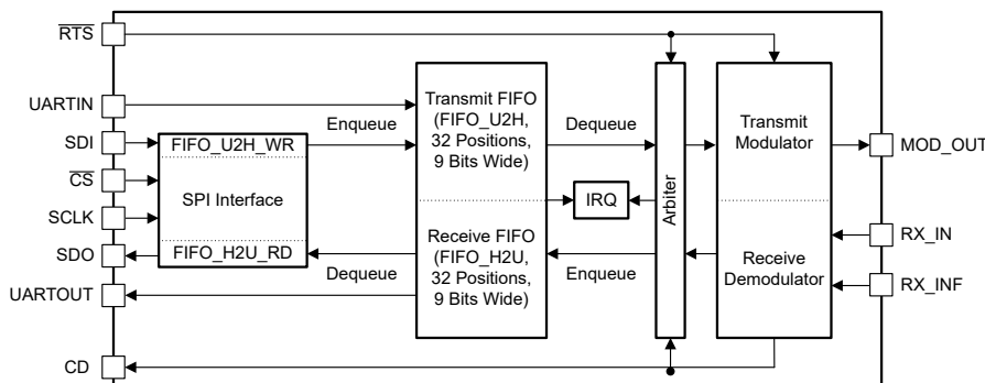
图 6-17. HART 架构
