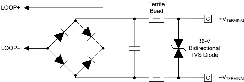
图 8-5. 环路输入保护
