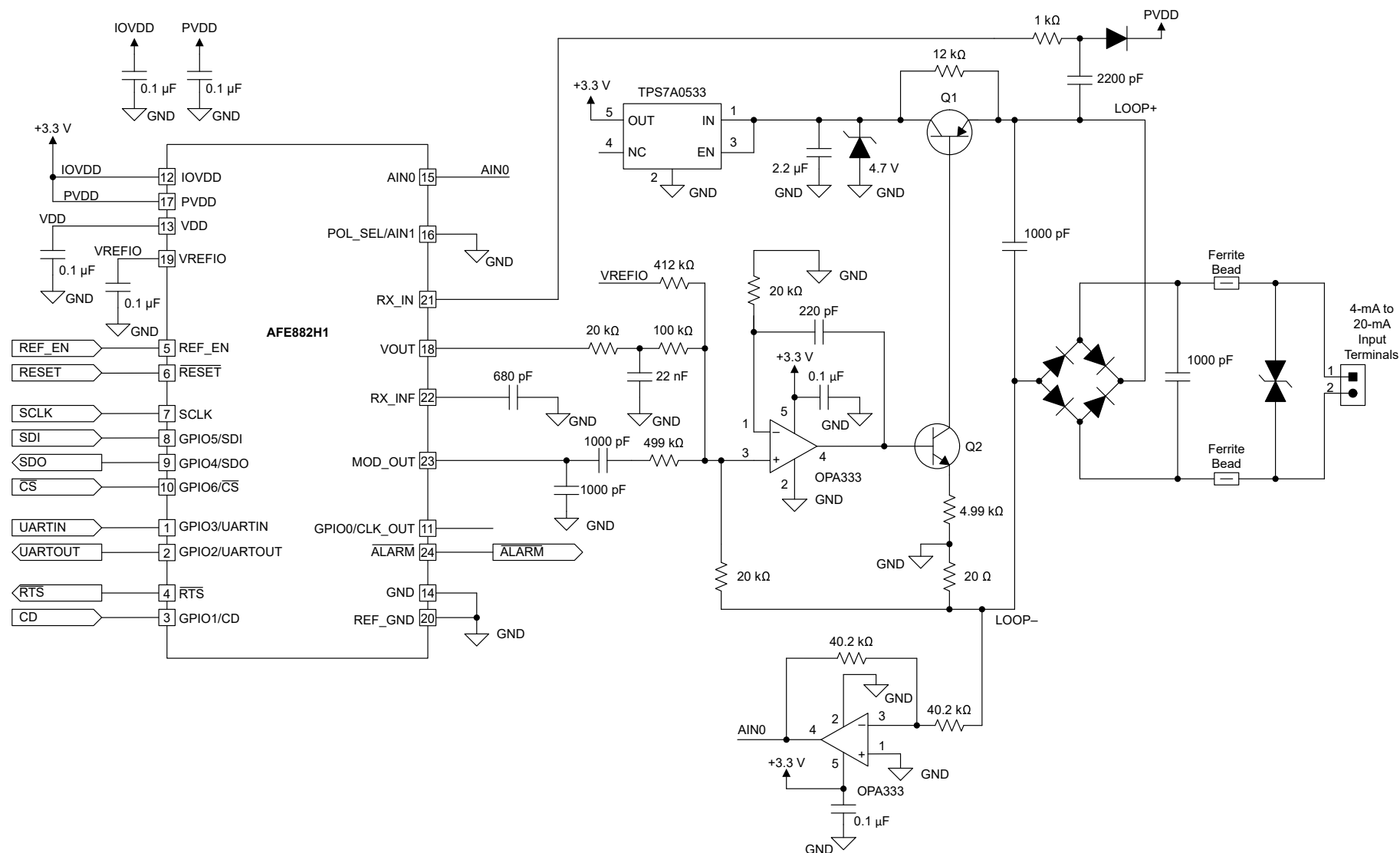
图 8-2. 4mA 至 20mA 电流变送器中的 AFEx82H1
