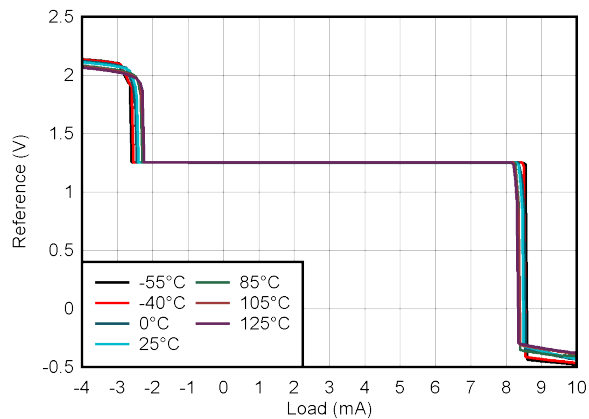
图 5-42. 基准拉电流和灌电流能力
