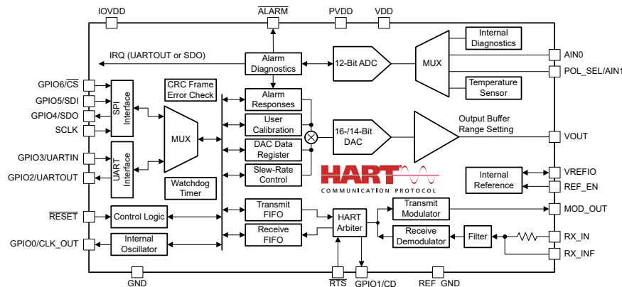
功能方框图
