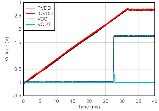
图 5-26. DAC 电源上电，PVDD = 2.7V
