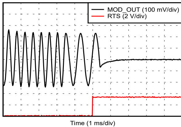
图 8-8. \overline{\text{RTS}} 停止时序
