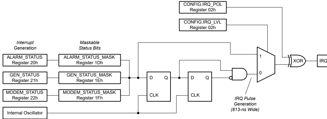
图 6-15. IRQ 方框图
