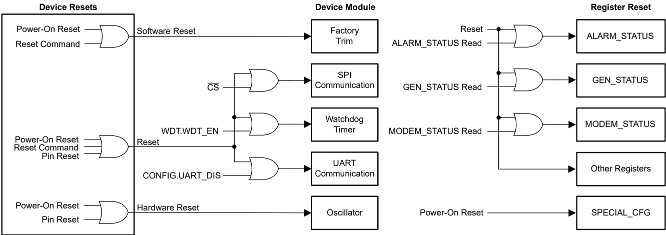
图 6-25. 复位条件
