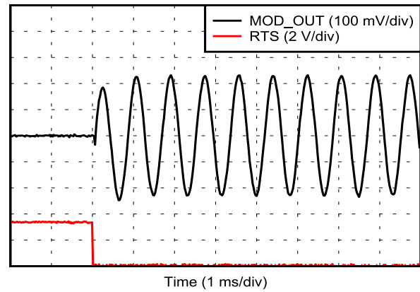
图 8-7. \overline{\text{RTS}} 启动时序
