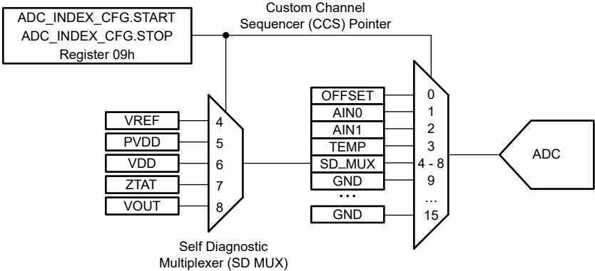
图 6-9. ADC 多路复用器控制
