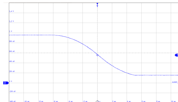
在 40 \Omega 分流器上测得的 24mA (0xF45D) 至 4mA (0x0BA3) 电流
