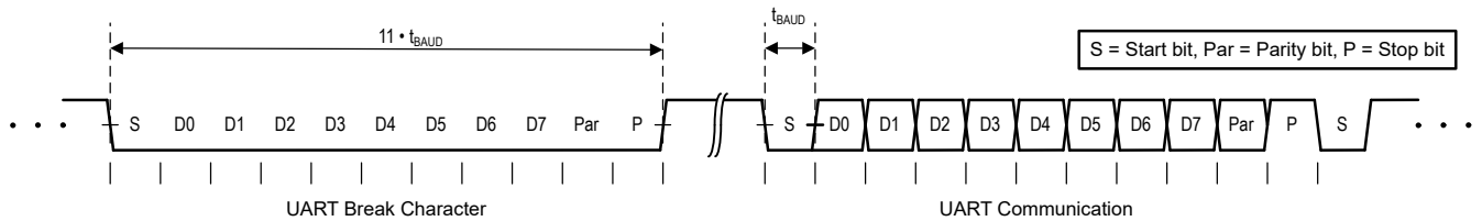
图 5-2. UBM 时序
