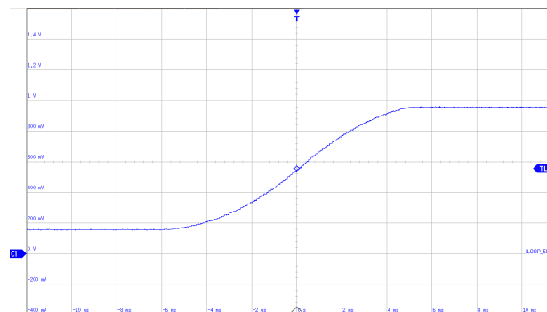
在 40 \Omega 分流器上测得的 4mA (0x0BA3) 至 24mA (0xF45D) 电流
