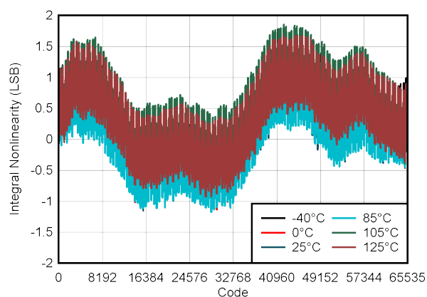
图 6-6. DAC INL vs Digital Input Code
