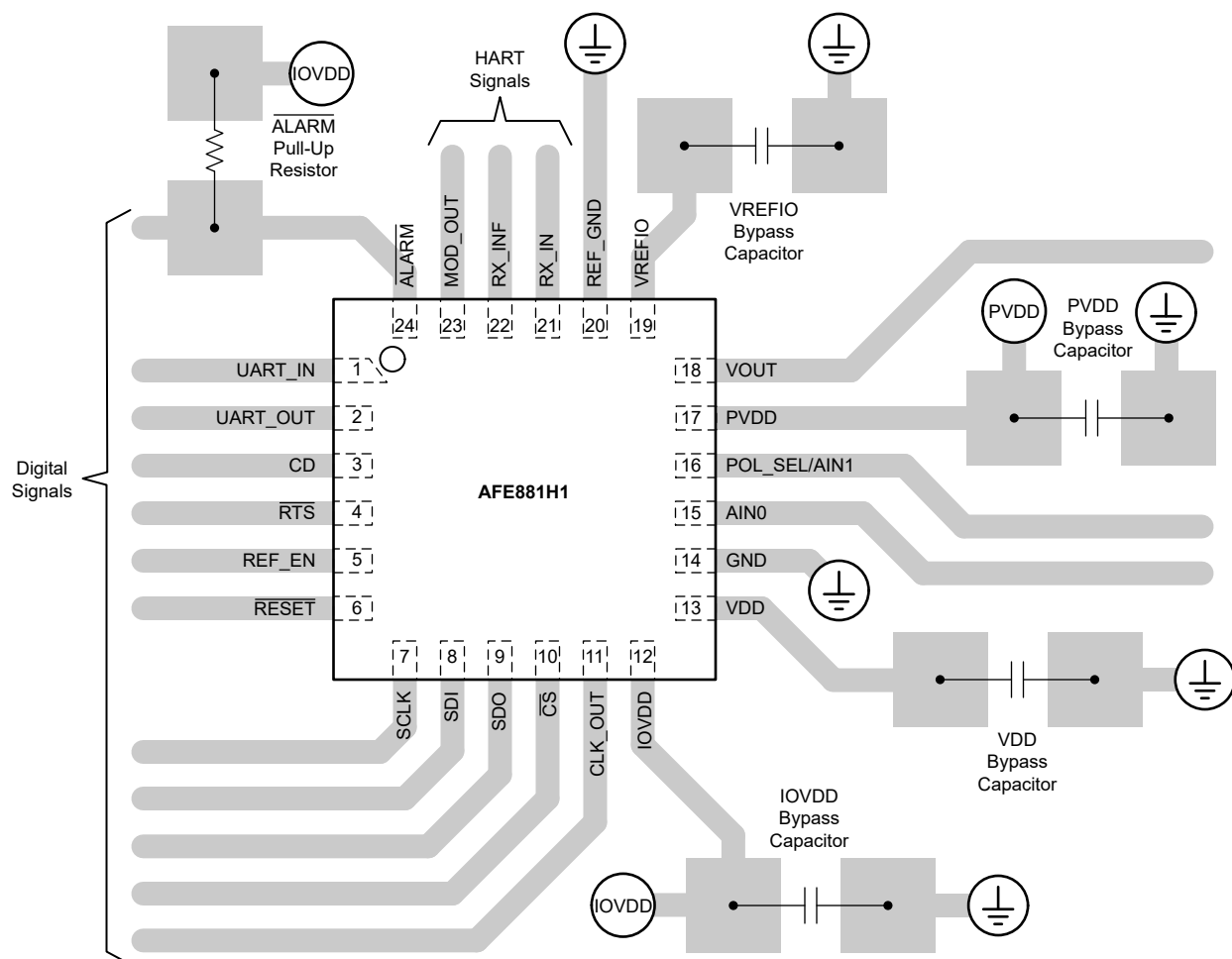
图 8-12. Layout Example
