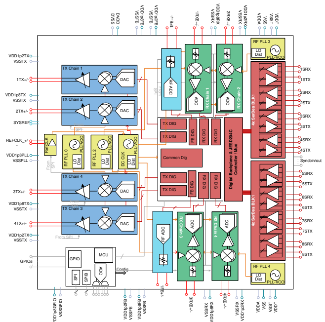
AFE7769 方框图
