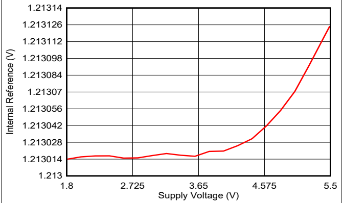
图 6-41. 内部基准与电源电压间的关系
