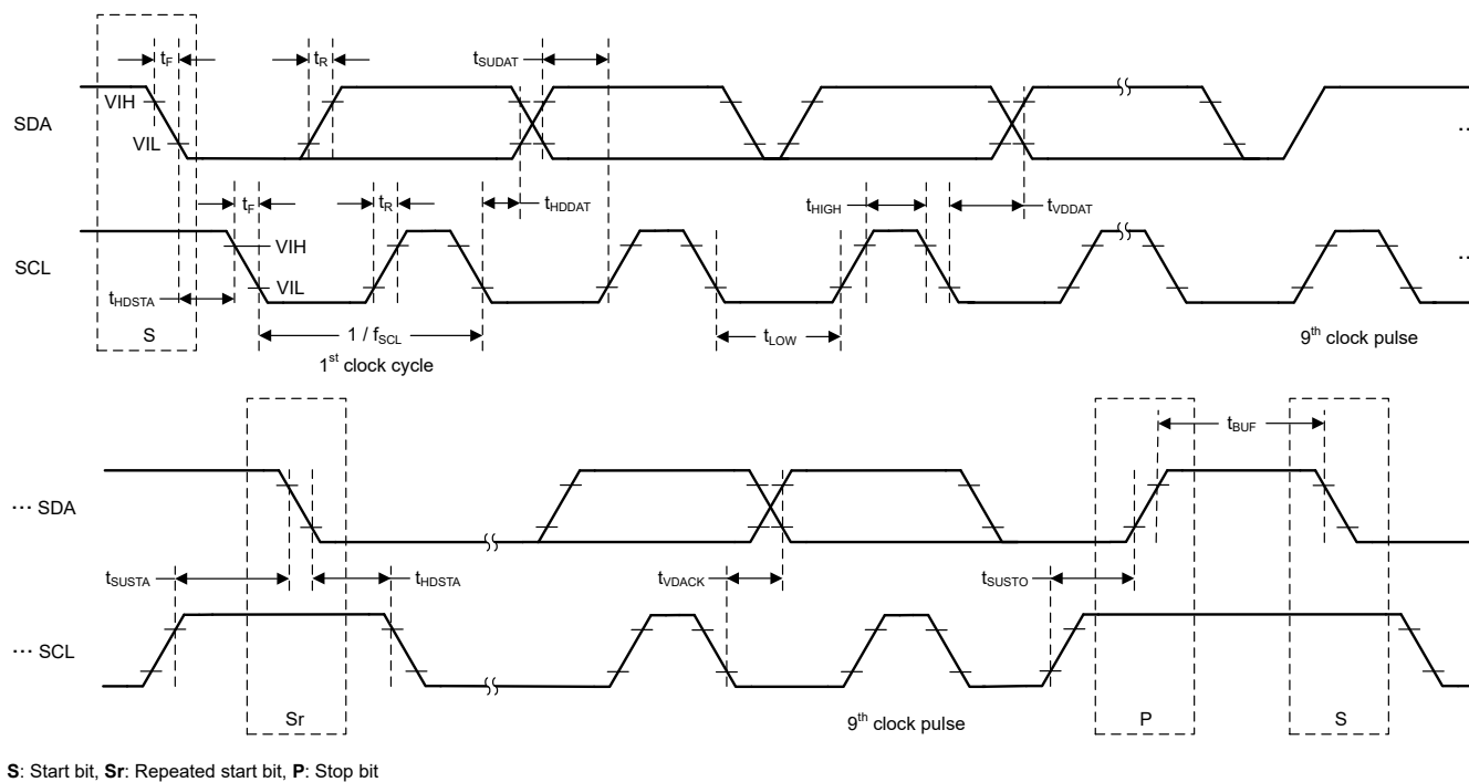
图 6-1. I²C 时序图
