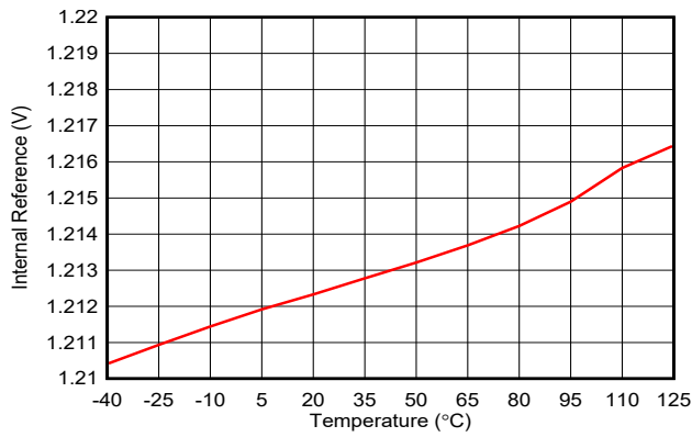
图 6-40. 内部基准与温度间的关系
