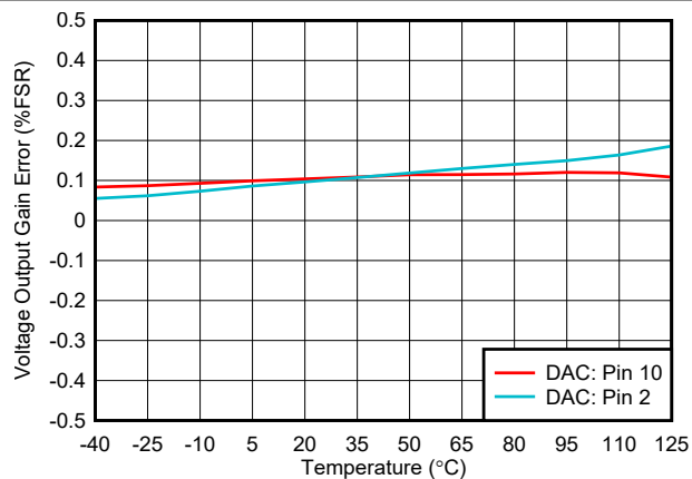
图 6-17. 电压输出增益误差与温度间的关系
