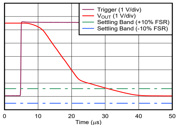
图 6-22. 电压输出建立时间 - 下降沿
