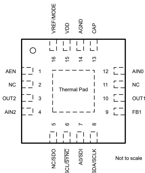
图 5-2. AFE539A4 : RTE 封装, 16 引脚 WQFN (顶视图)
