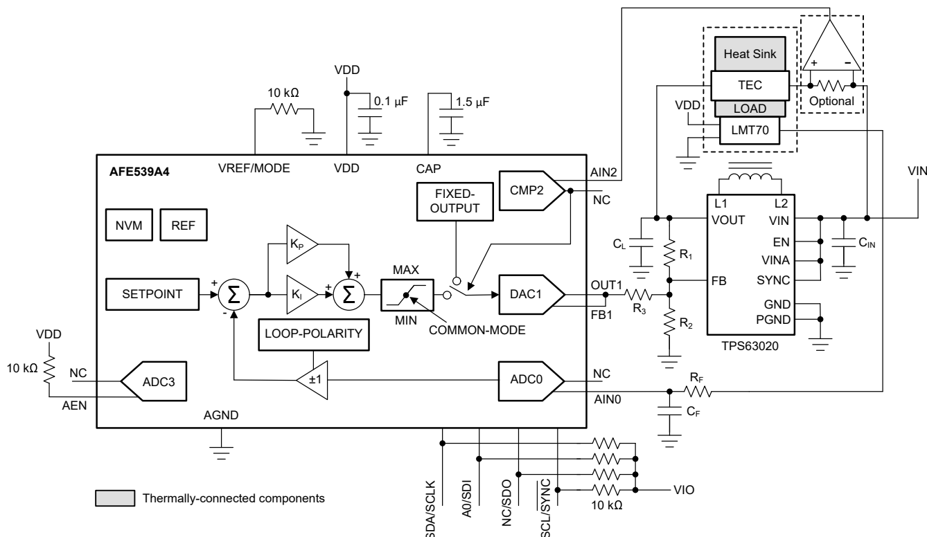
图 8-1. TEC 控制
