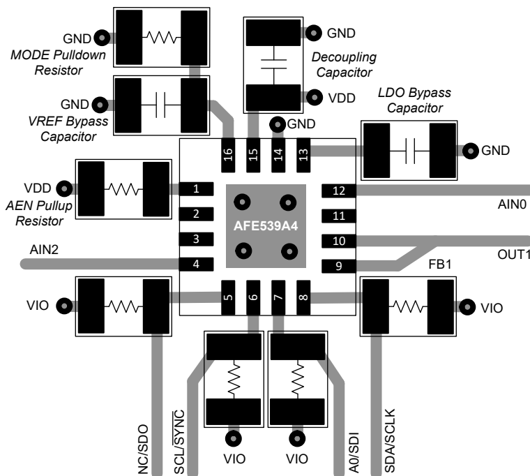
图 8-4. 布局示例
