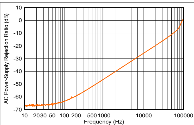
图 6-29. 电压输出交流 PSRR 与频率间的关系
