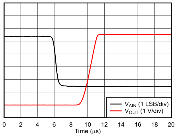
推挽模式下的比较器输出
