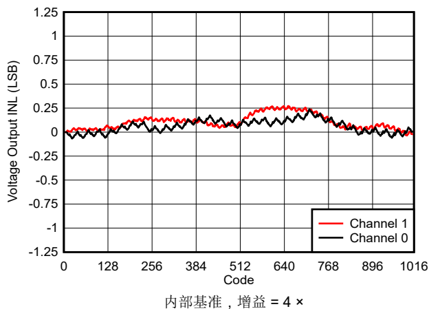
图 5-4. 电压输出 INL 与数字输入代码间的关系
