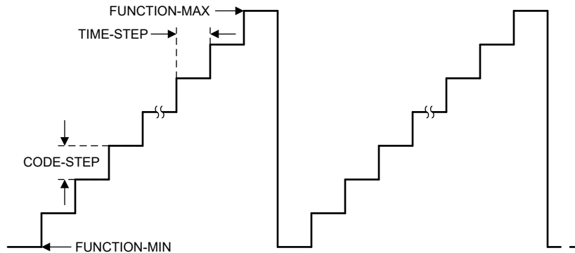
图 6-12. 锯齿波形
