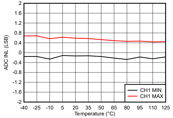
图 5-54. ADC INL 与温度间的关系
