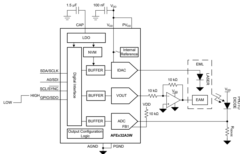
使用 AFE x 32A3W 的电吸收调制激光器 (EML) 控制
