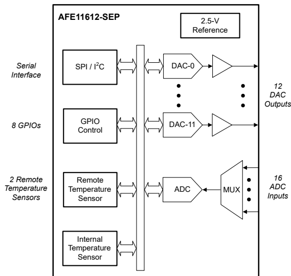
简化原理图
