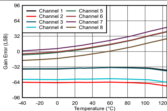
图 5-37. 增益误差与温度间的关系, 范围 = \pm 5V
