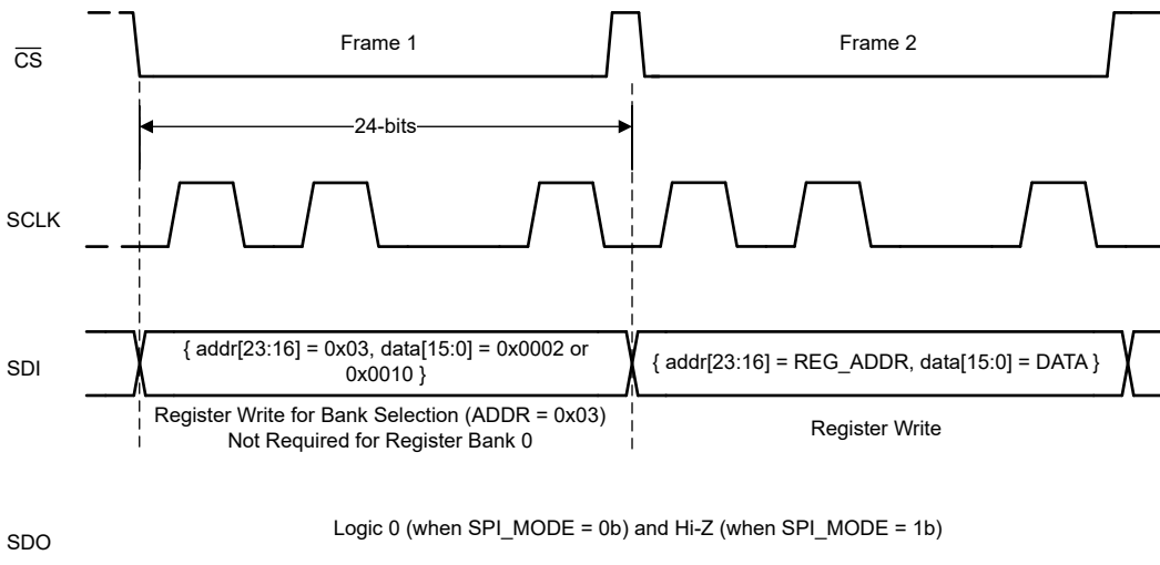
图 6-10. 寄存器写入
