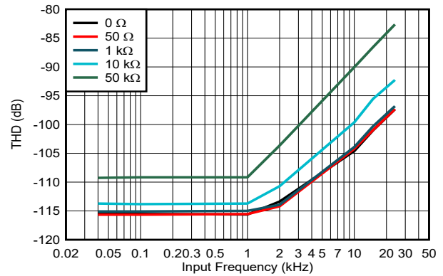
图 5-25. THD 与输入频率间的关系, 高带宽模式, RANGE = \pm 10V , AD9817
