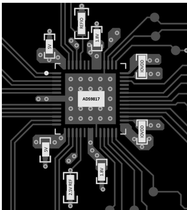
图 8-5. 示例布局
