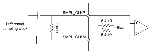
图 6-4. 交流耦合差分采样时钟
