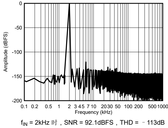
图 5-12. 使用低带宽 LPF 时的典型 FFT, RANGE = \pm 10V
