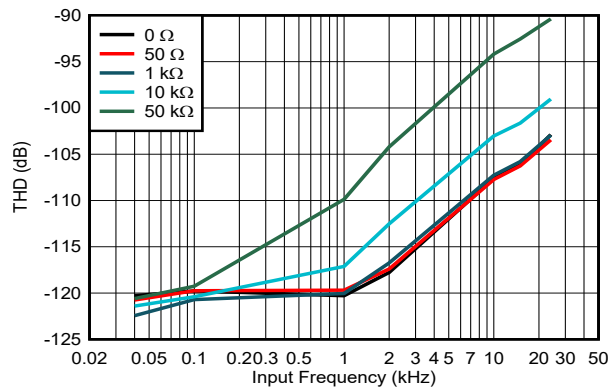
图 5-26. THD 与输入频率间的关系, 低带宽模式, RANGE = \pm 5V , AD9815
