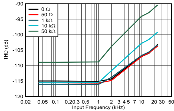
图 5-24. THD 与输入频率间的关系, 低带宽模式, RANGE = \pm 10V , AD9817
