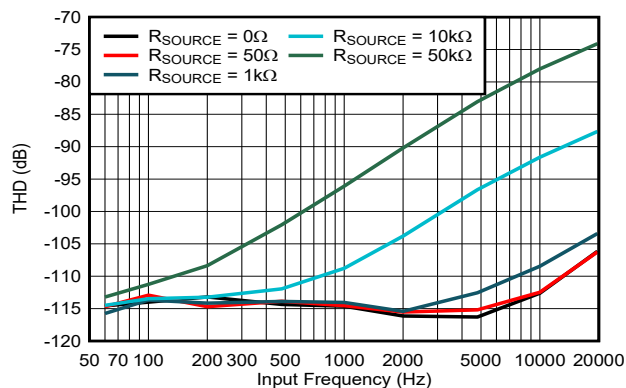
低带宽 LPF 且 RANGE = \pm 10V
