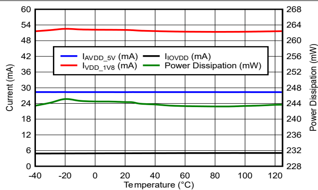
图 5-36. 电源电流和总功率损耗与温度间的关系
