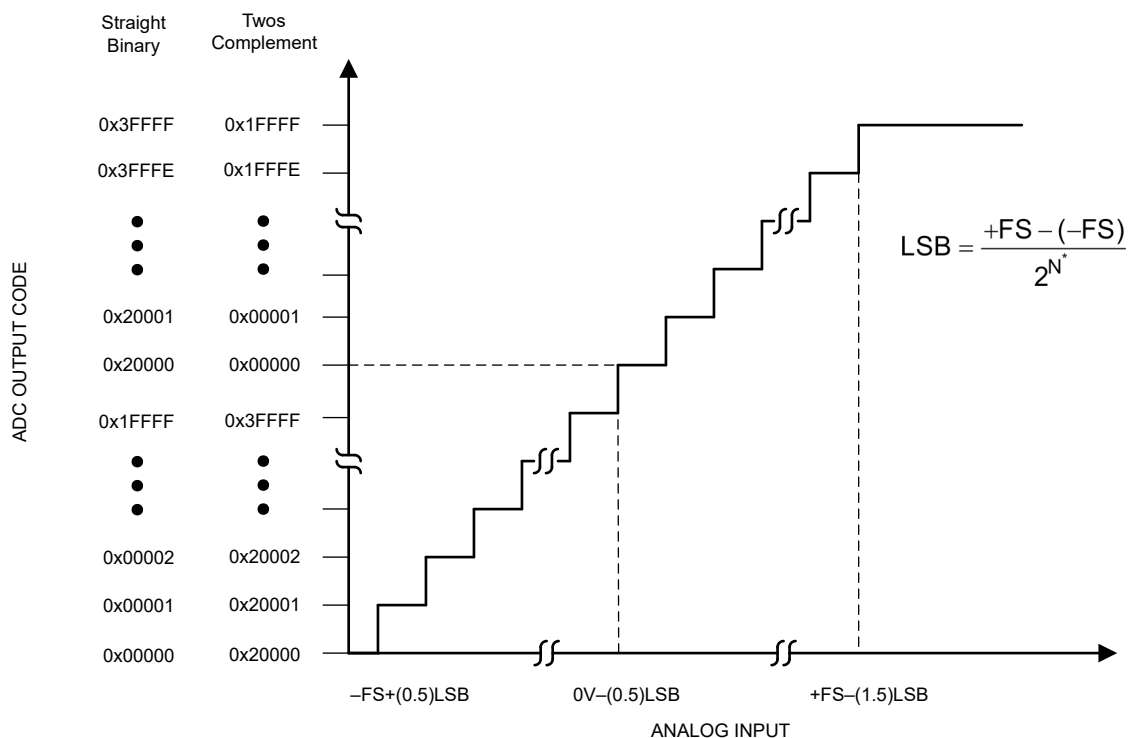
图 6-3. 传输特性
