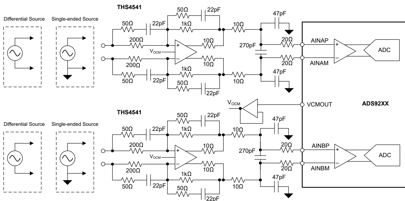
图 9-7. \leq 1\text{MHz} 输入信号带宽的数据采集 (DAQ) 电路
