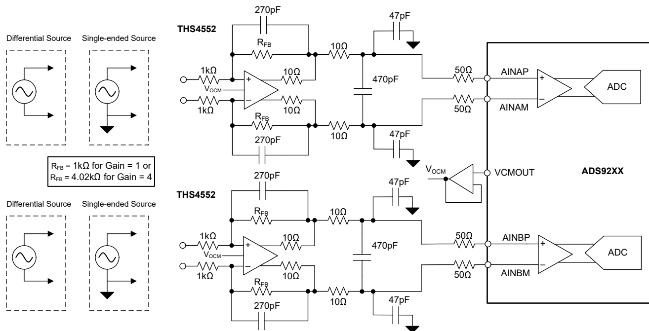
图 9-4. \leq 100\text{kHz} 输入信号带宽的数据采集 (DAQ) 电路
