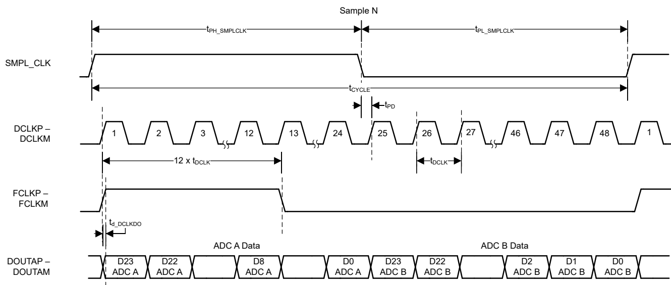
图 6-4. LVDS 数据接口：单路 SDR
