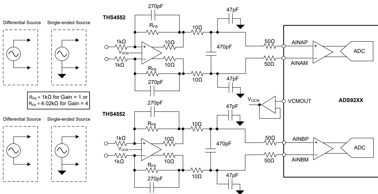
图 9-1. \leq 20\text{kHz} 输入信号带宽的数据采集 (DAQ) 电路
