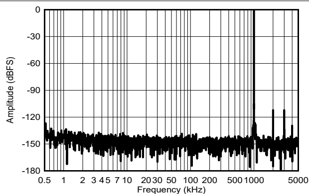
f_{IN} = 1\text{MHz} ， \text{SNR} = 95\text{dBFS} ， \text{THD} = -106\text{dB}
