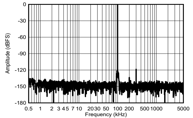
f_{IN} = 100\text{kHz} ， \text{SNR} = 95.5\text{dBFS} ， \text{THD} = -118.2\text{dB}
