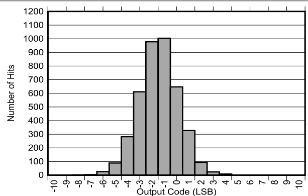
标准偏差 = 1.63\text{LSB}
