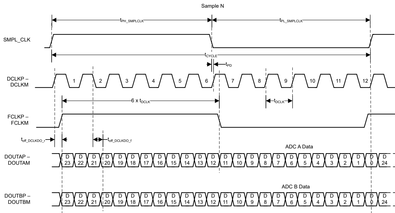
图 6-1. LVDS 数据接口：双路 DDR
