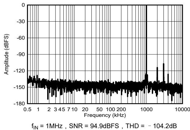
图 6-23. f_{IN} = 1\text{MHz} 时的典型 FFT
