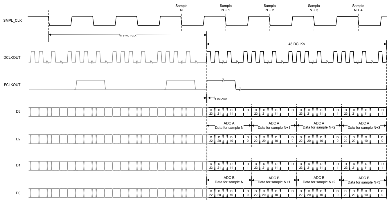
图 5-4. 4-SDO SDR CMOS 数据接口
