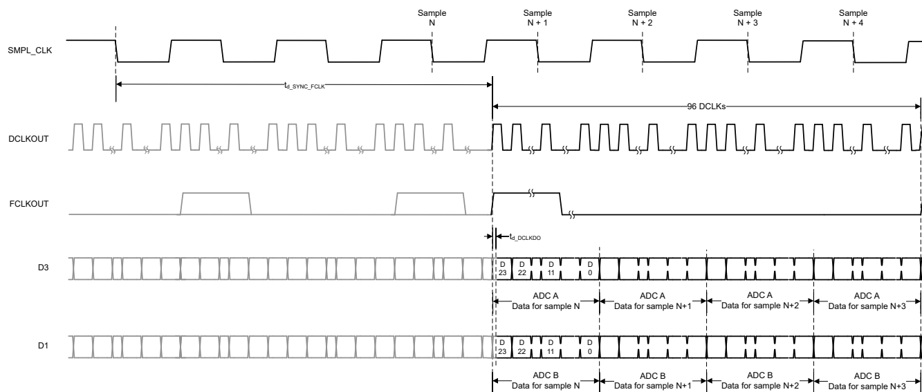
图 5-5. 2-SDO SDR CMOS 数据接口
