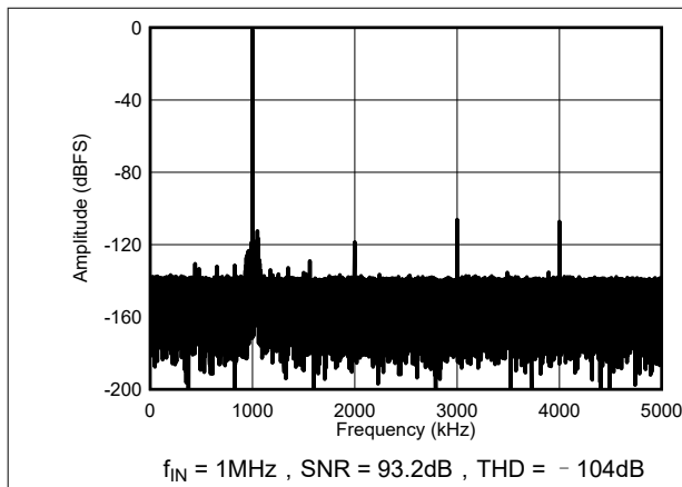
图 8-8. 10MSPS 时的典型 FFT : ADS9128
