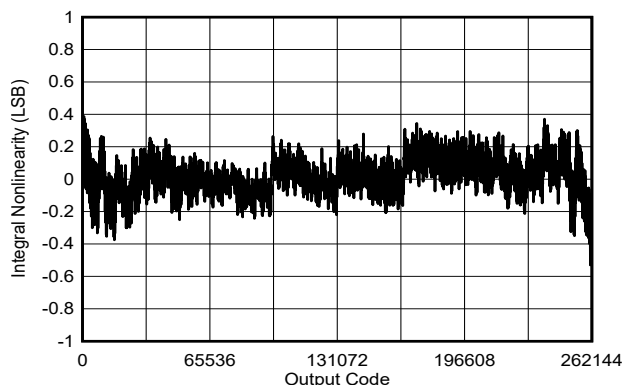
图 6-17. 典型 INL
