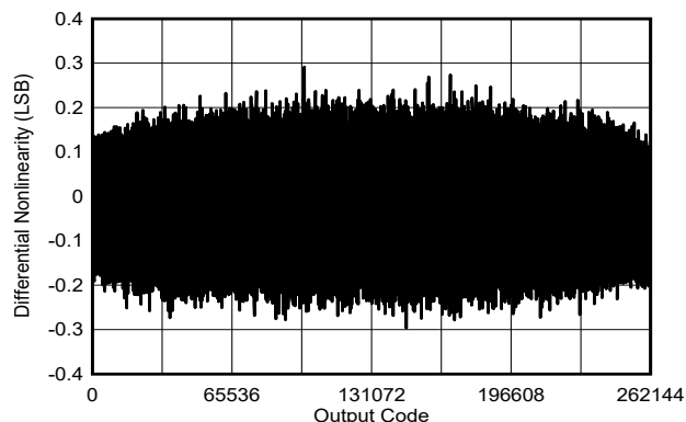
图 6-18. 典型 DNL
