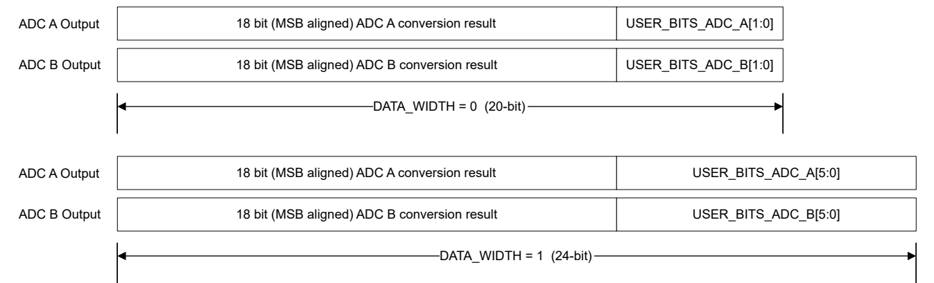
图 7-8. 启用 LSB XOR 的数据帧宽度组成
