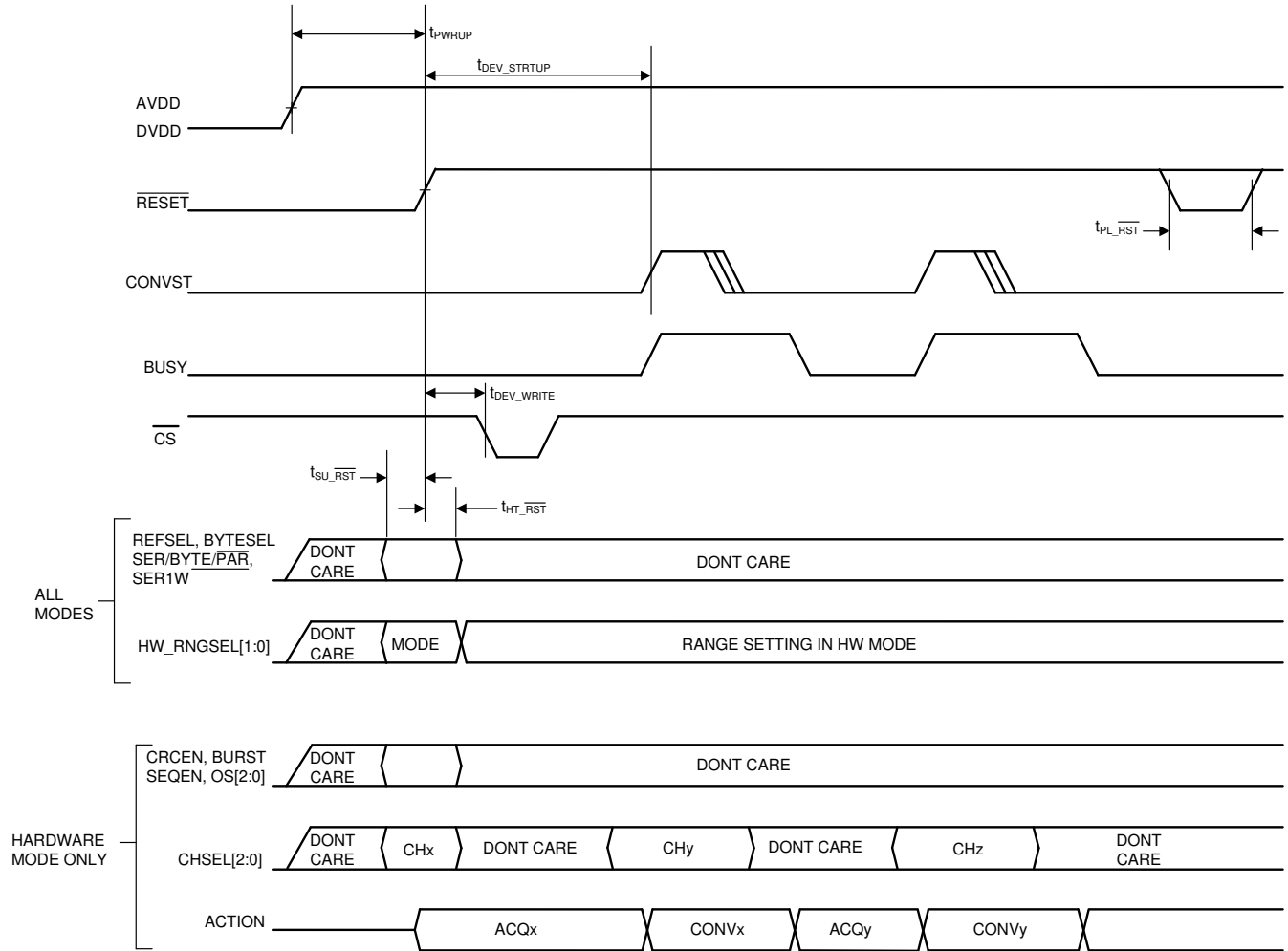
图 6-2. 复位时序
