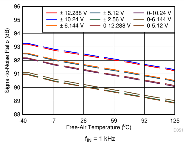
图 6-37. SNR vs Temperature
