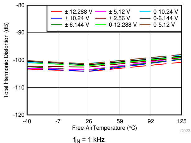
图 6-40. THD vs Temperature
