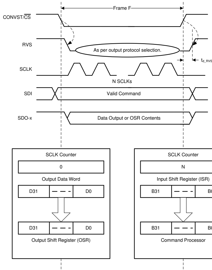
图 7-25. Data Transfer Frame
