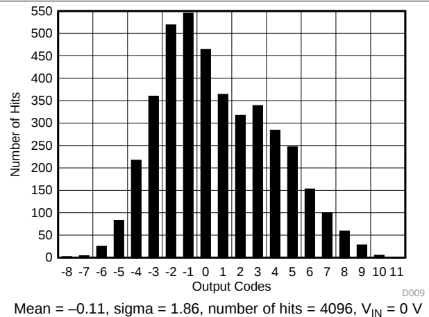
图 13. DC Histogram of Codes ( \pm 10\text{ V} )
