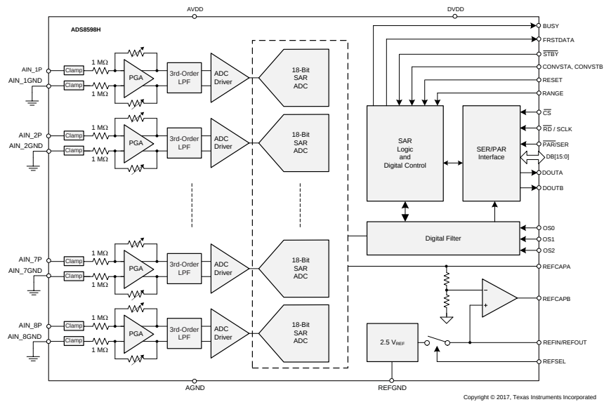
简化框图
