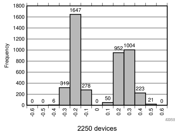
图 5-7. Typical INL Distribution (LSB)
