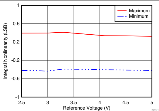
图 5-11. INL vs Reference Voltage
