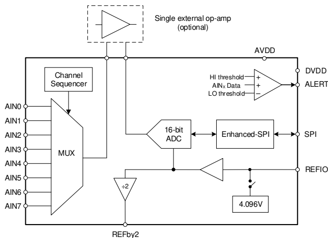
ADS816x 方框图
