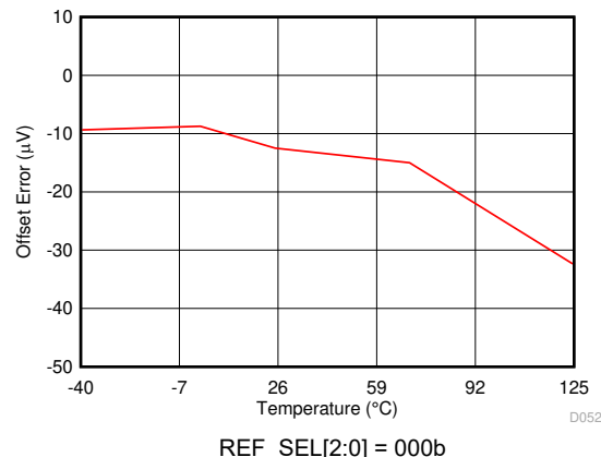
图 5-14. Offset Error vs Temperature
