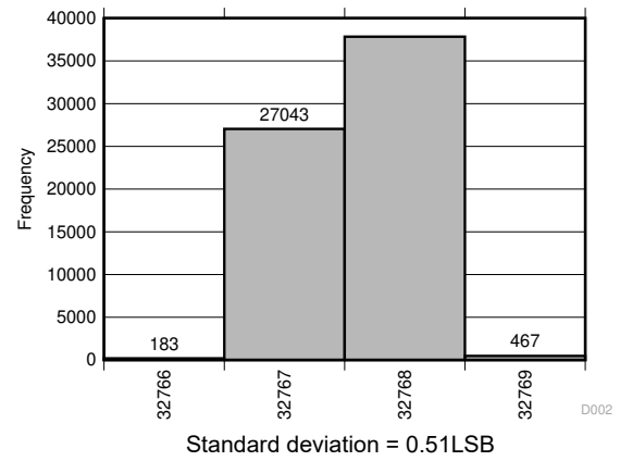
图 5-18. DC Input Histogram
