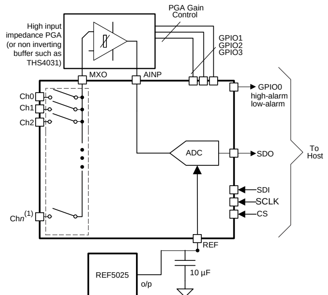
详细方框图
