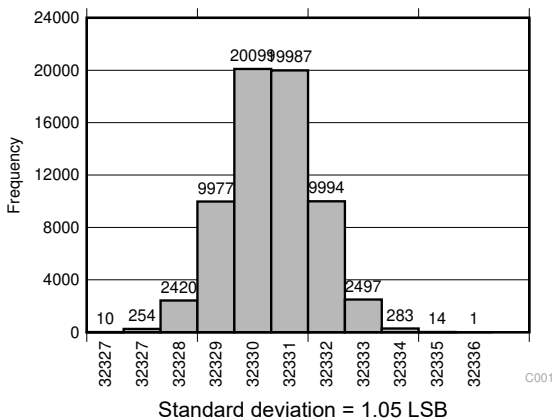
图 5-13. DC Input Histogram
