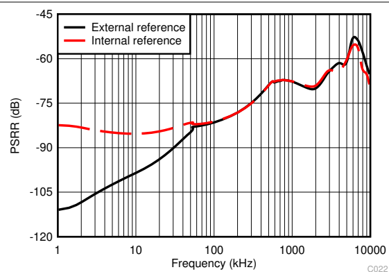
图 5-22. PSRR vs Frequency
