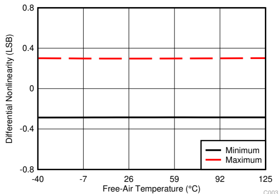
图 5-3. Typical DNL
