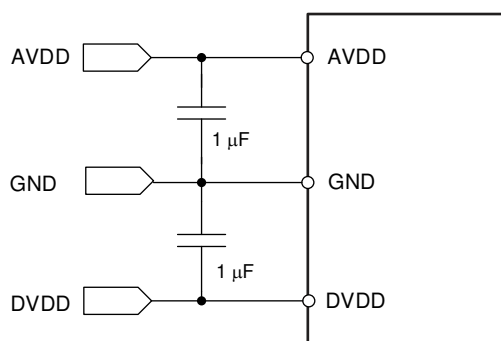
图 7-3. Power-Supply Decoupling
