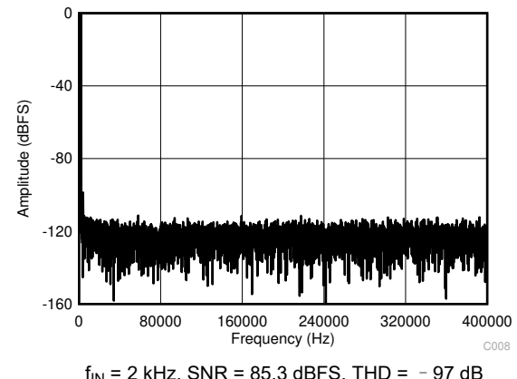
图 5-14. Typical FFT
