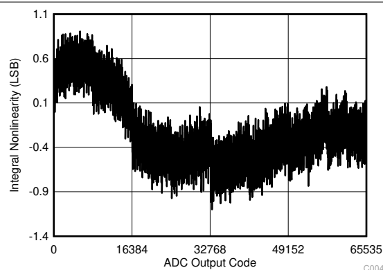
图 5-4. Typical INL
