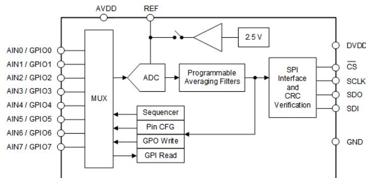
ADS7067 方框图
