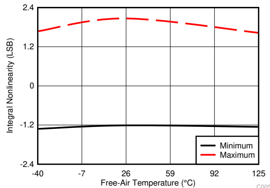
图 5-4. Typical INL
