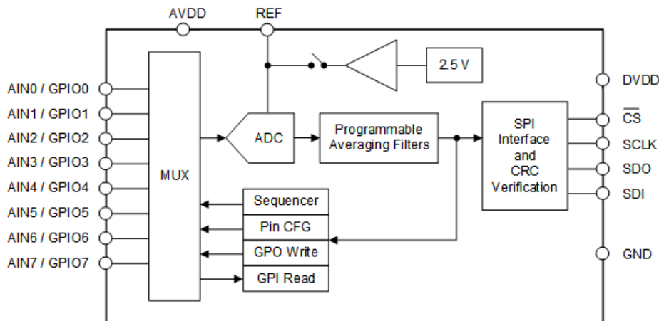
ADS7066 方框图
