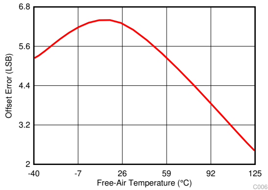
图 6-9. Offset Error vs Temperature
