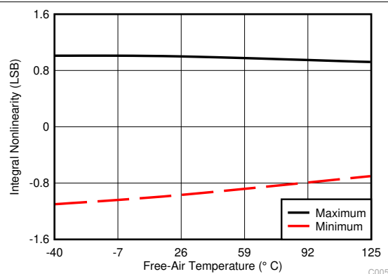
图 6-4. Typical INL
