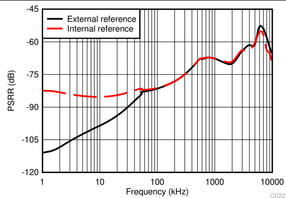
图 6-22. PSRR vs Frequency
