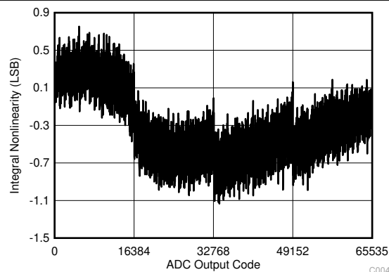
图 6-4. Typical INL
