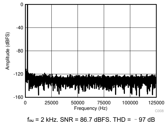
图 6-14. Typical FFT
