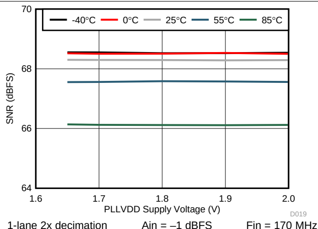
图 23. SNR vs. PLLVDD
