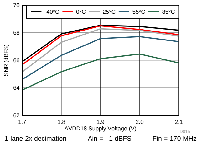
图 19. SNR vs. AVDD18
