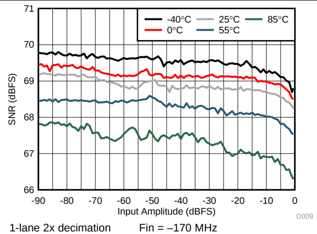
图 13. SNR vs. Amplitude
