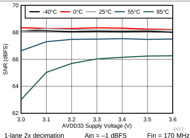
图 21. SNR vs. AVDD33
