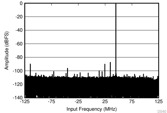
图 6-41. FFT for 170-MHz Input Signal
