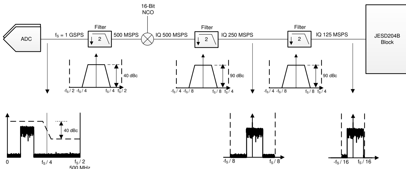
图 7-14. Operating Mode 6
