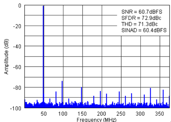
图 7-9. FFT for 700-MHz Input Signal (Auto Off)
