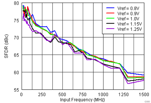
图 7-15. SFDR vs. Vref (Auto On)
