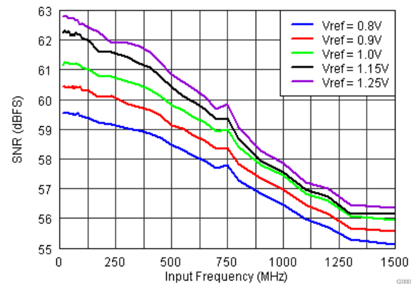
图 7-17. SNR vs. Vref (Auto On)
