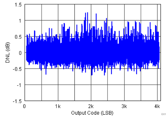
图 7-25. DNL
