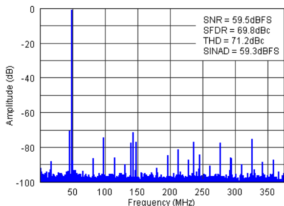
图 7-8. FFT for 700-MHz Input Signal (Auto On)
