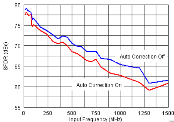
图 7-10. SFDR vs. Input Frequency
