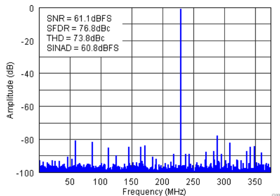
图 7-5. FFT for 230-MHz Input Signal (Auto Off)
