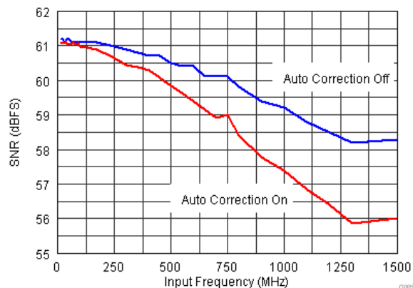
图 7-11. SNR vs. Input Frequency
