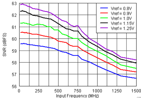
图 7-18. SNR vs. Vref (Auto Off)
