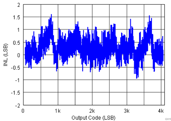
图 7-24. INL
