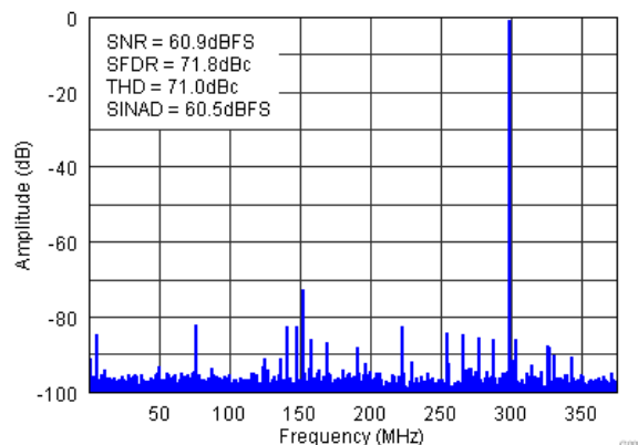
图 7-7. FFT for 450-MHz Input Signal (Auto Off)
