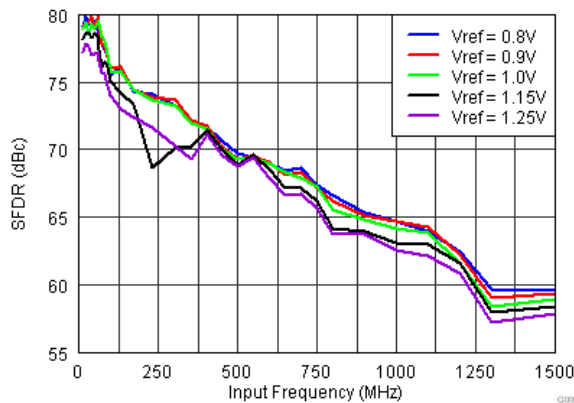
图 7-16. SFDR vs. Vref (Auto Off)
