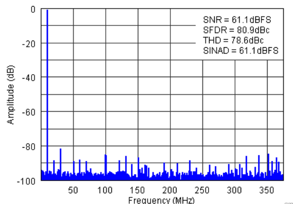
图 7-3. FFT for 10-MHz Input Signal (Auto Off)
