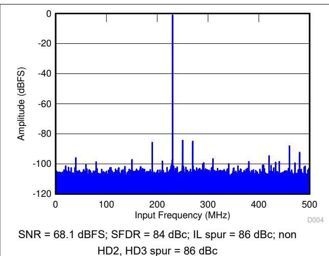
图 9-19. FFT for 230-MHz Input Signal
