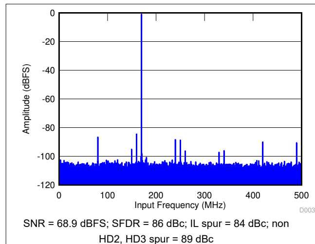
图 9-18. FFT for 170-MHz Input Signal
