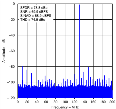
图 5-5. 130MHz 输入信号的频谱性能 FFT
