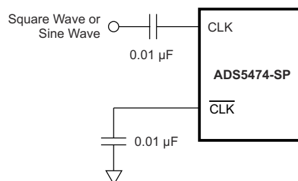
图 6-6. 单端时钟
