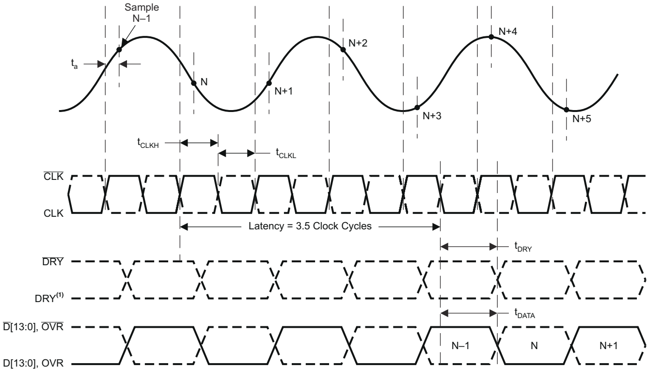
图 5-2. 时序图
