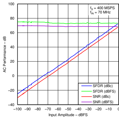
图 5-19. 交流性能与输入幅度间的关系 (70MHz 输入信号)
