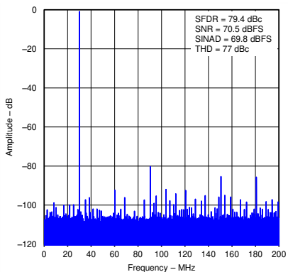
图 5-3. 30MHz 输入信号的频谱性能 FFT
