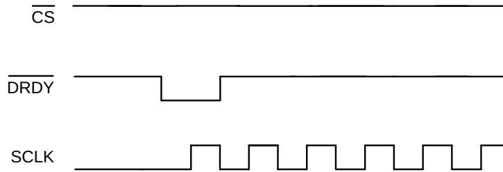
Figure 60. SPI 总线多路复用的 \overline{\text{DRDY}} 和 SCLK 行为
