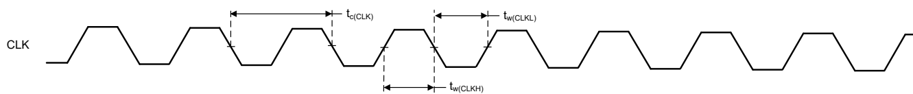
图 5-1. 时钟时序要求
