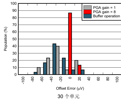
图 5-16. 偏移电压误差分布
