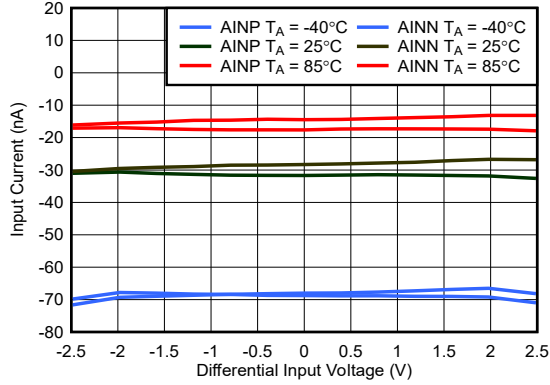
图 5-27. PGA 输入电流与输入电压间的关系
