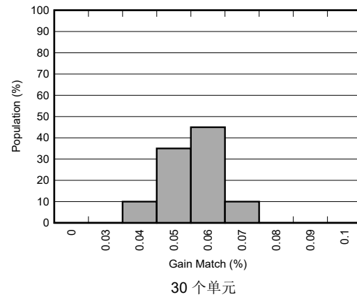
图 5-22. 增益匹配分布
