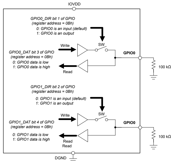
图 7-19. GPIO 操作
