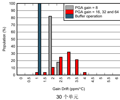
图 5-21. 增益漂移分布图
