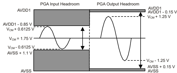
图 7-6. PGA 余量 (AVDD1 = 3.3V、增益 = 2)
