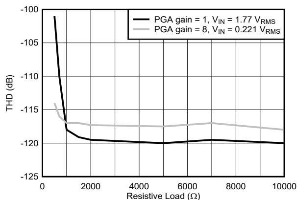
图 7-3. THD 性能与 R_{LOAD} 间的关系
