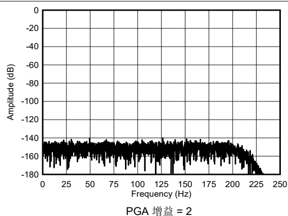
图 5-10. 短接输入 FFT
