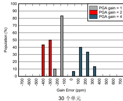
图 5-18. 增益误差分布图
