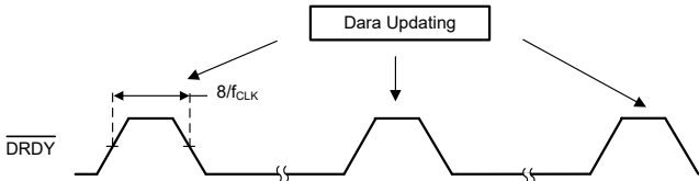
图 7-22. 未检索到数据的 \overline{\text{DRDY}}
