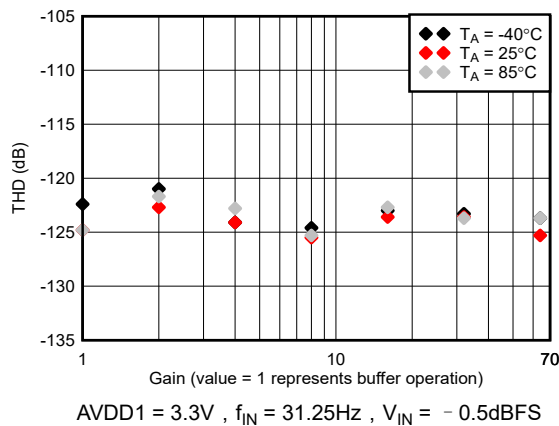
图 5-23. THD 与 PGA 增益间的关系
