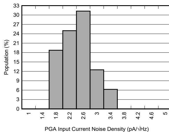
图 9-2. PGA 输入电流噪声分布
