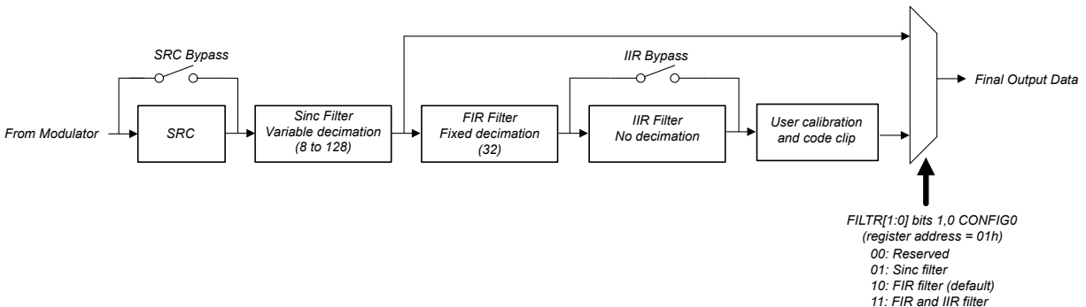
图 7-10. 数字滤波器方框图
