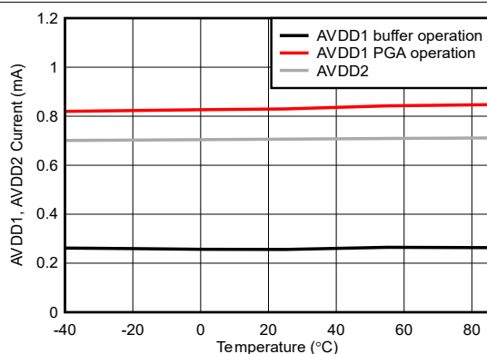
图 5-33. 电源电流与温度间的关系
