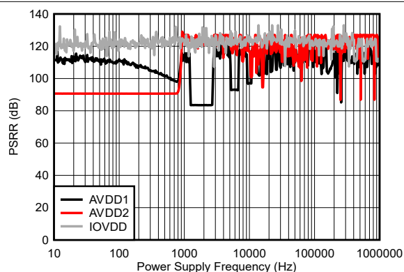
图 5-34. PSRR 与电源频率间的关系
