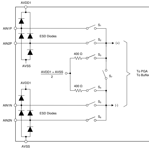
图 7-1. 模拟输入和多路复用器
