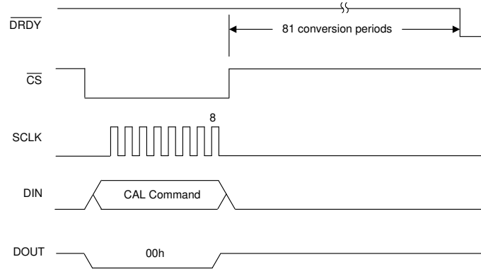
图 7-21. 校准命令
