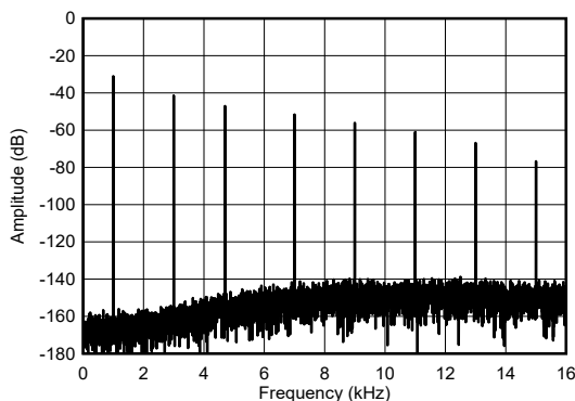
图 7-13. Sinc 滤波器的 FFT 输出 ( f_{\text{DATA}} = 32\text{kSPS} )
