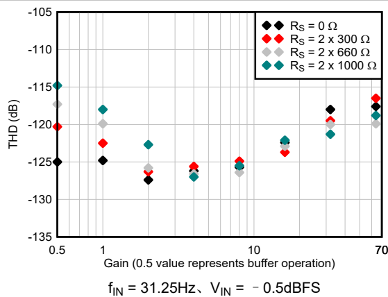
图 5-25. THD 与源阻抗间的关系
