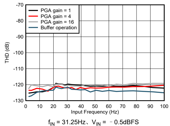
图 5-24. THD 与输入频率间的关系
