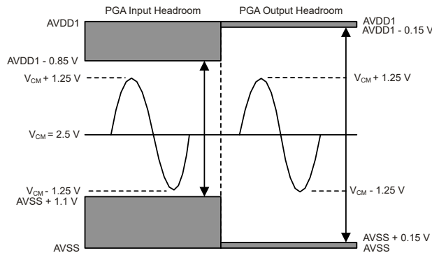
图 7-5. PGA 余量 (AVDD1 = 5V、增益 = 1)
