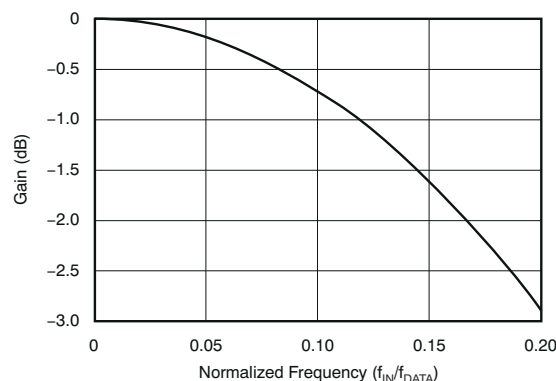
图 7-12. Sinc 滤波器 -3dB 响应
