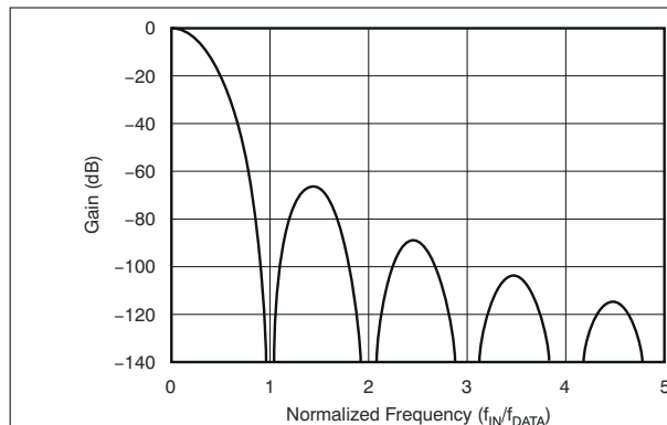
图 7-11. Sinc 滤波器频率响应
