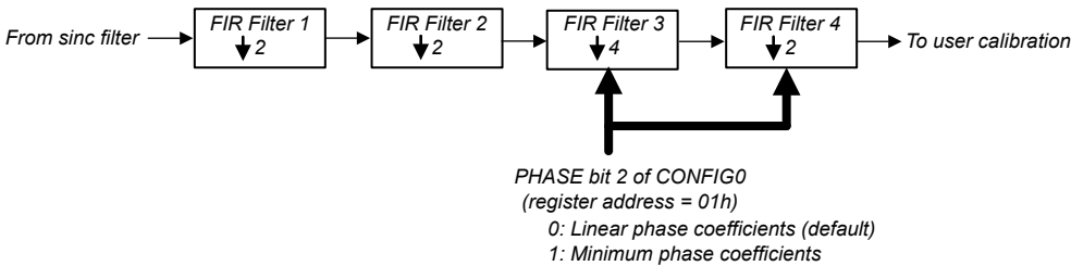
图 7-14. FIR 滤波器
