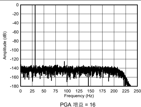
图 5-11. 短接输入 FFT
