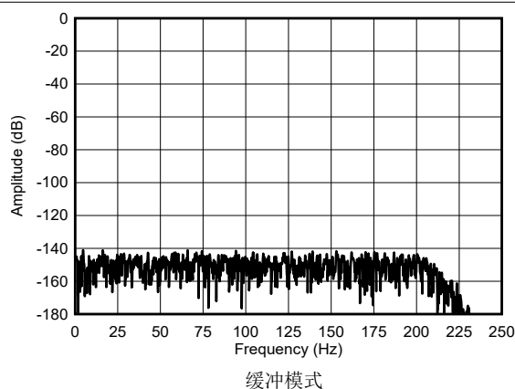
图 5-9. 短接输入 FFT
