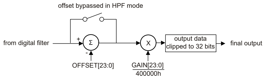
图 7-20. 校准方框图
