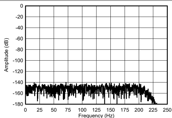
图 5-12. 满量程输入 FFT
