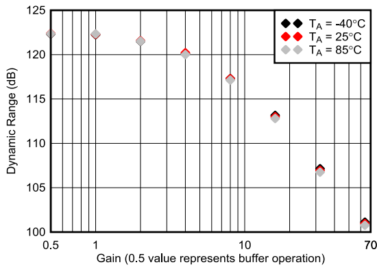
图 5-15. 动态范围与 PGA 增益间的关系
