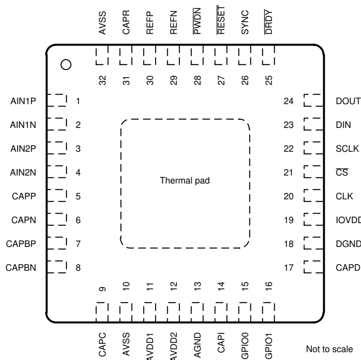
图 4-1. RHB 封装，32 引脚，5mm × 5mm VQFN（顶视图）
