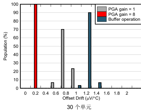
图 5-17. 偏移电压漂移分布
