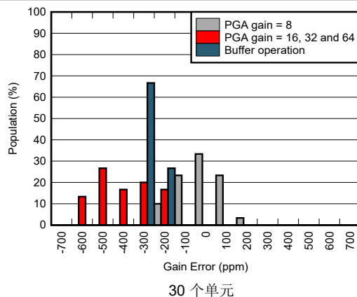
图 5-19. 增益误差分布图
