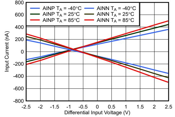
图 5-28. 缓冲器输入电流与输入电压间的关系
