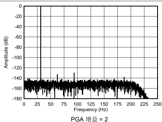
图 5-12. 满量程输入 FFT
