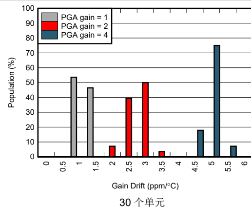
图 5-20. 增益漂移分布图
