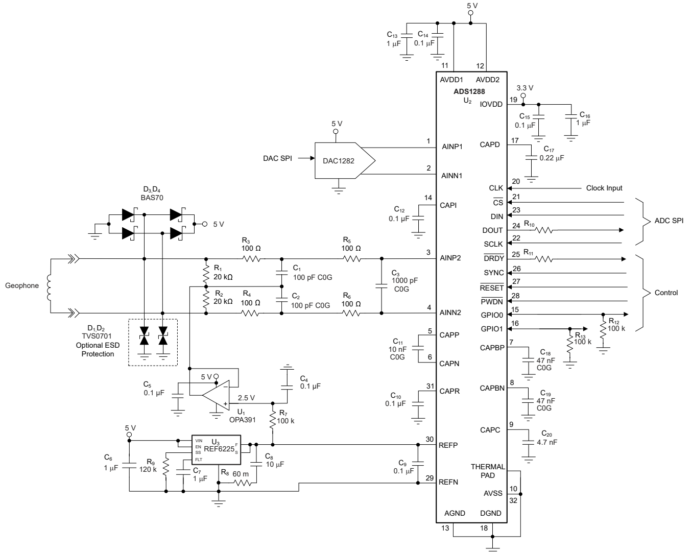
图 9-1. 地震检波器输入应用示例
