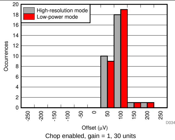
图 34. Offset Error Histogram
