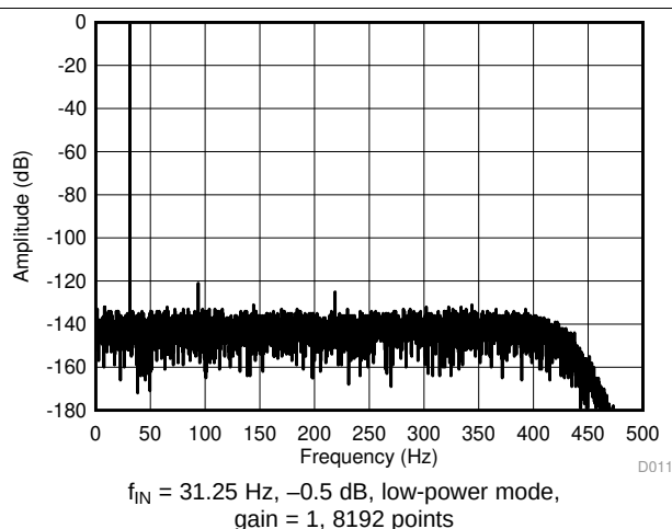
图 18. Output Spectrum
