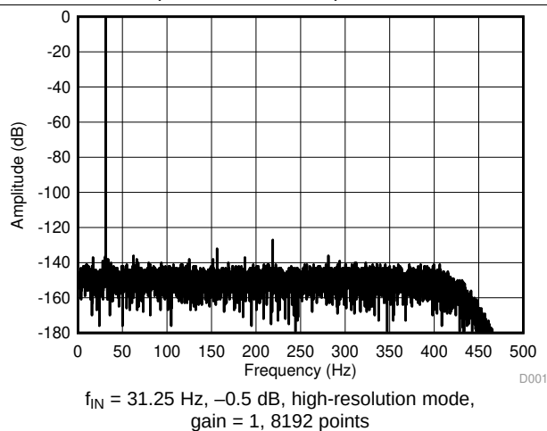
图 14. Output Spectrum
