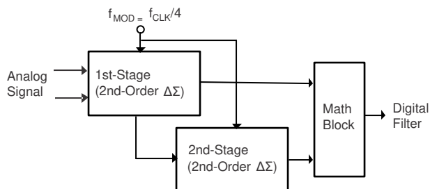
图 46. Modulator
