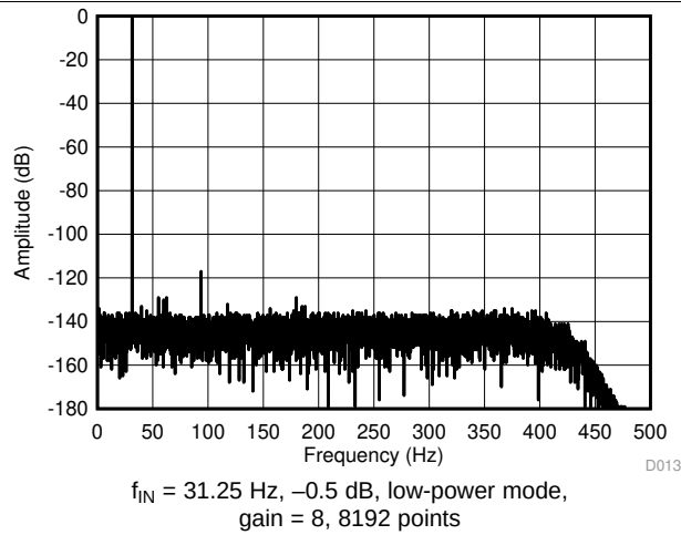
图 20. Output Spectrum
