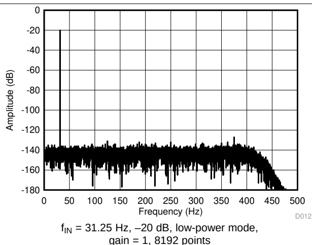
图 19. Output Spectrum
