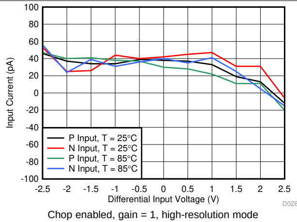
图 32. Input Current vs Input Voltage
