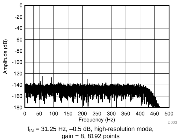
图 16. Output Spectrum
