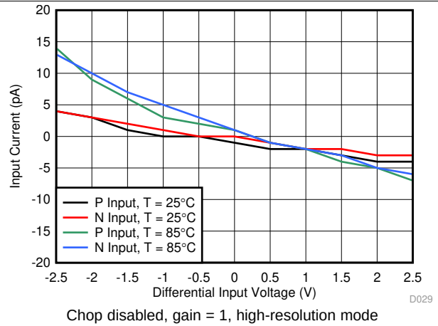
图 33. Input Current vs Input Voltage
