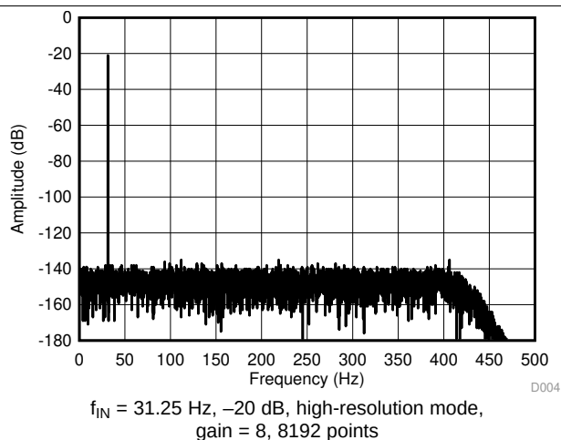
图 17. Output Spectrum
