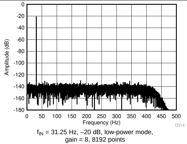
图 21. Output Spectrum
