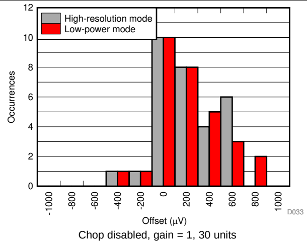
图 35. Offset Error Histogram
