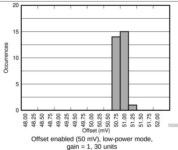
图 36. Offset Error Histogram
