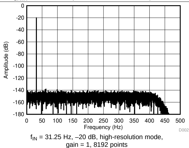
图 15. Output Spectrum
