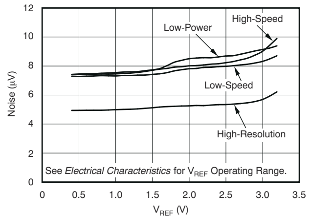
图 5-46. 噪声与基准电压间的关系
