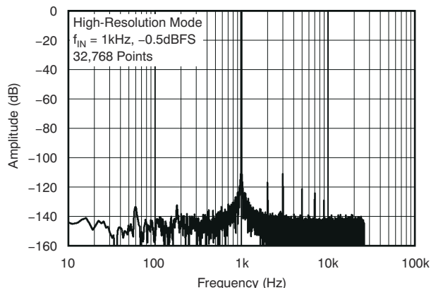
图 5-7. 输出频谱
