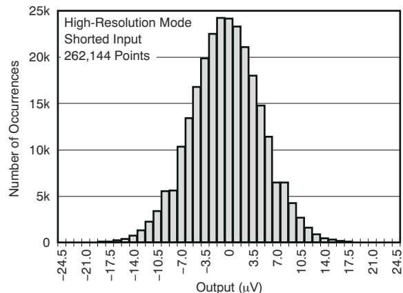
图 5-10. 噪声直方图
