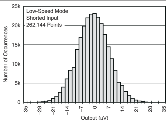
图 5-18. 噪声直方图
