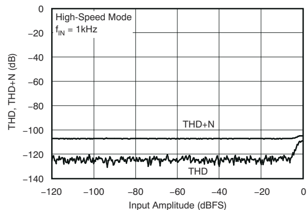
图 5-20. 总谐波失真与输入幅度间的关系
