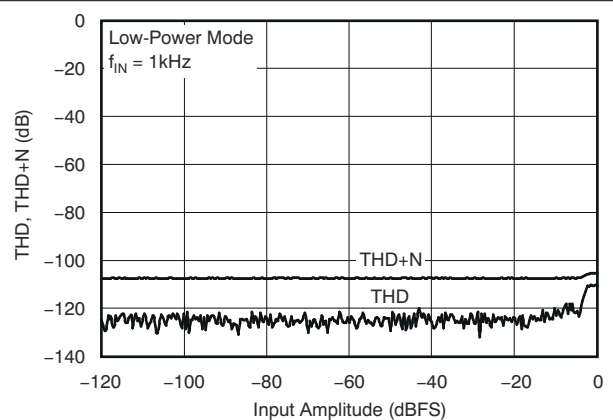
图 5-24. 总谐波失真与输入幅度间的关系
