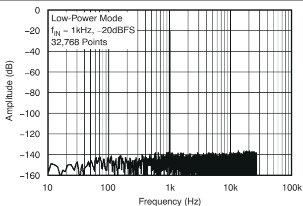
图 5-12. 输出频谱
