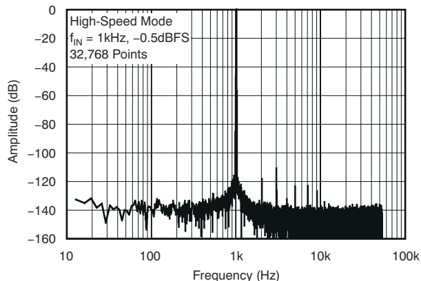
图 5-3. 输出频谱
