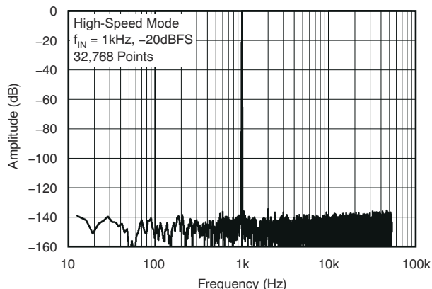
图 5-4. 输出频谱
