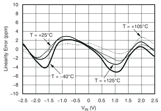
图 5-42. 线性误差与输入电平间的关系
