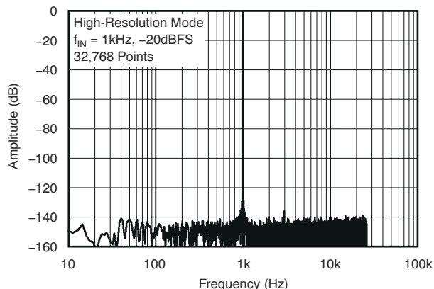
图 5-8. 输出频谱
