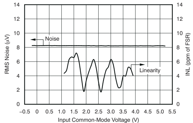
图 5-44. 噪声和线性与输入共模电压间的关系
