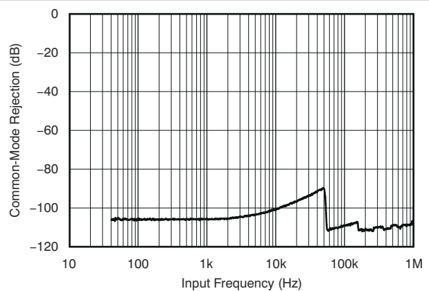
图 5-48. 共模抑制与输入频率间的关系
