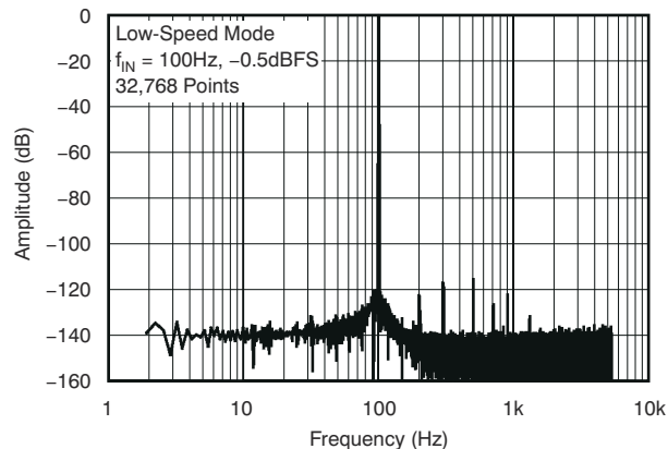
图 5-15. 输出频谱
