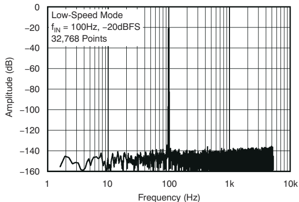
图 5-16. 输出频谱
