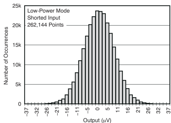
图 5-14. 噪声直方图
