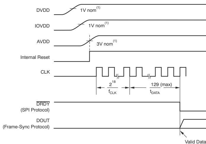
图 7-3. 启动序列
