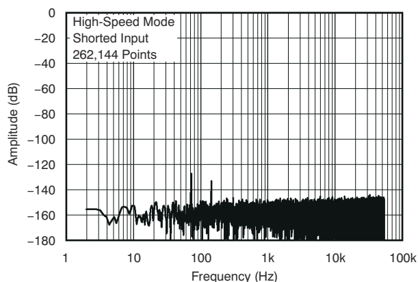
图 5-5. 输出频谱
