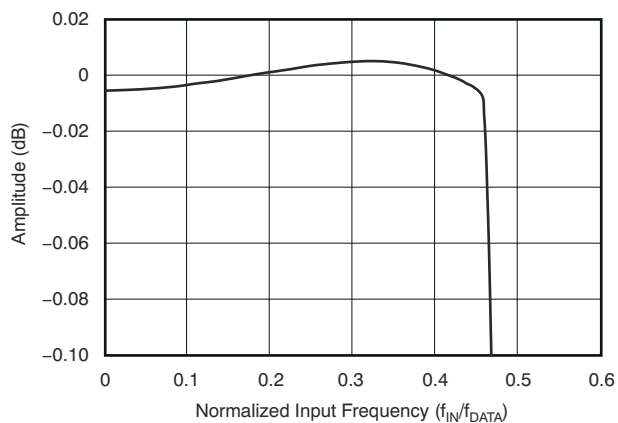
图 6-6. 高分辨率模式的通带响应
